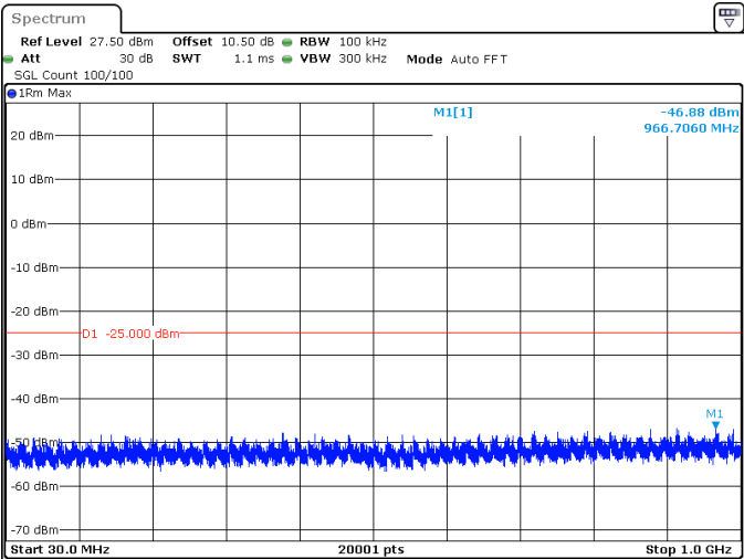
25MHz_30kHz_2607.5MHz_DFT-s-OFDM QPSK_RB1@0 -46.88 dBm
