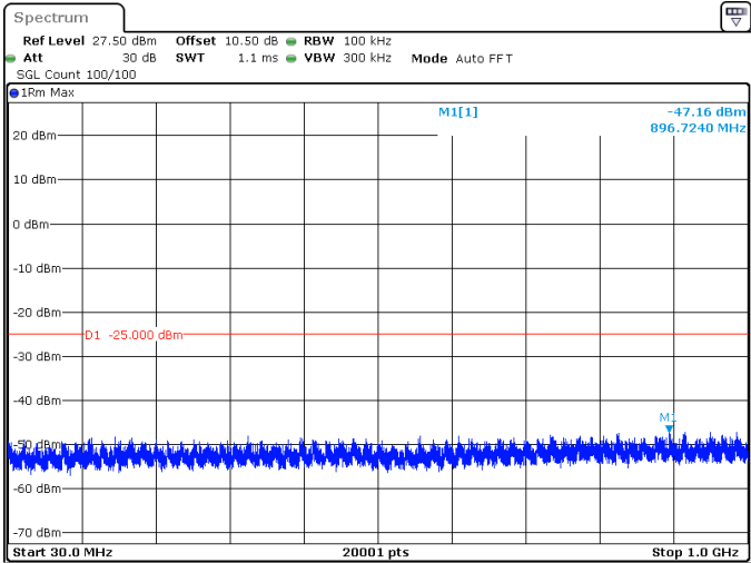
20MHz_30kHz_2610MHz_DFT-s-OFDM QPSK_RB1@50 -47.16 dBm
