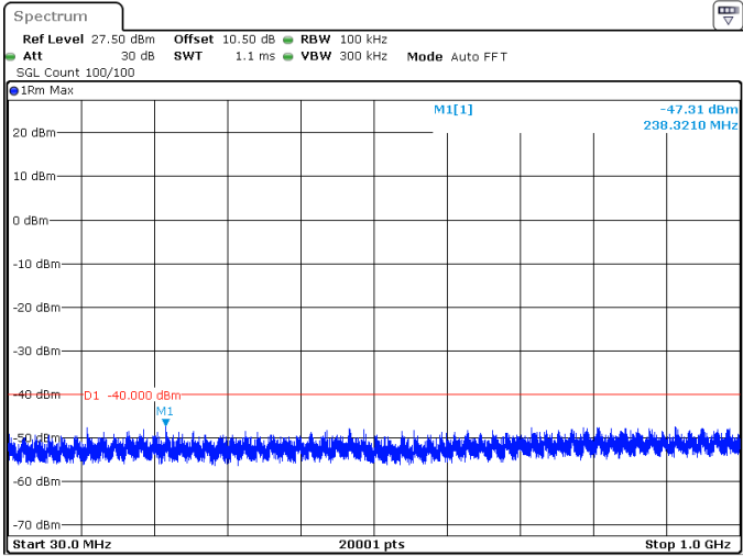
10MHz_30kHz_2355MHz_DFT-s-OFDM QPSK_RB1@0 -47.31 dBm
