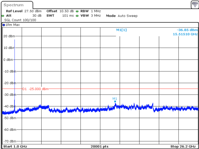
25MHz_30kHz_2595MHz_DFT-s-OFDM QPSK_RB1@0 -36.85 dBm
