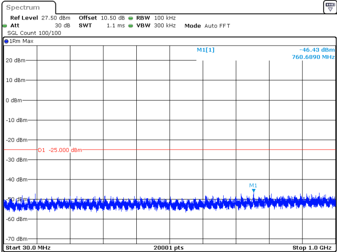
10MHz_15kHz_2685MHz_DFT-s-OFDM QPSK_RB1@0 -46.43 dBm
