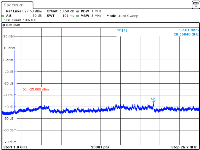
20MHz_30kHz_2595MHz_DFT-s-OFDM QPSK_RB50@0 -37.01 dBm
