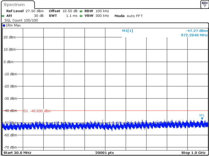
10MHz_30kHz_2310MHz_DFT-s-OFDM QPSK_RB1@0 -47.27 dBm
