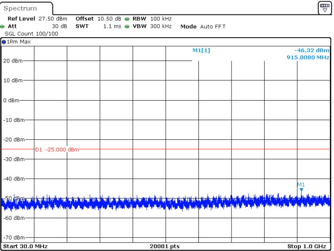
10MHz_15kHz_2593.005MHz_DFT-s-OFDM QPSK_RB50@0 -46.32 dBm
