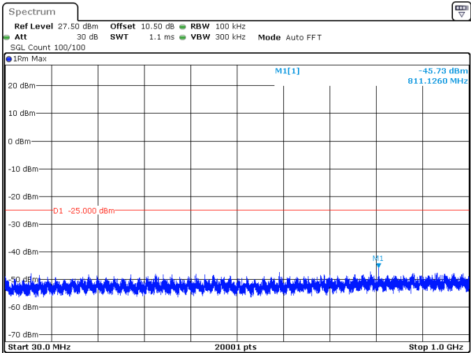
30MHz_30kHz_2595MHz_DFT-s-OFDM QPSK_RB1@0 -45.73 dBm
