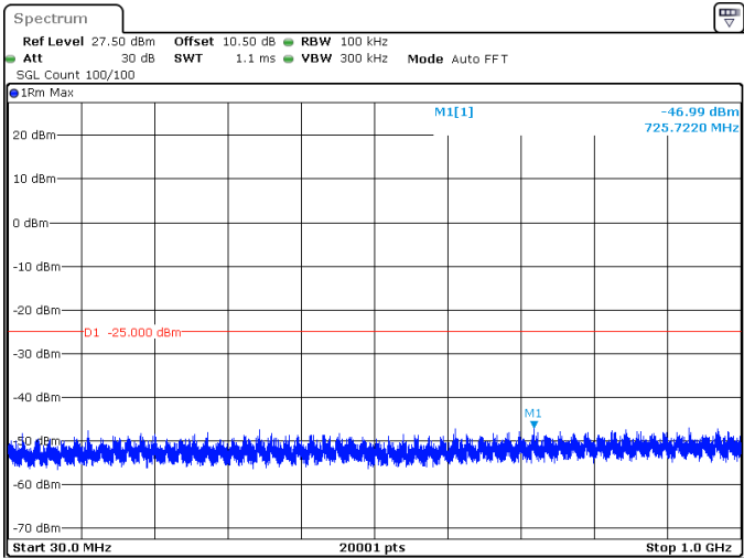
10MHz_30kHz_2615MHz_DFT-s-OFDM QPSK_RB24@0 -46.99 dBm
