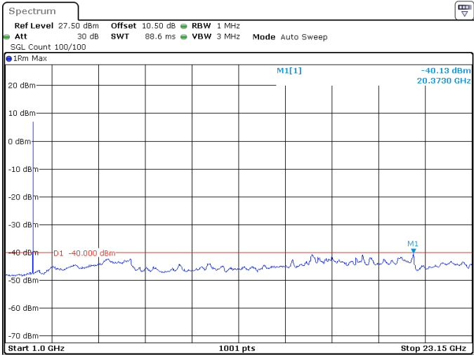
10MHz_30kHz_2310MHz_DFT-s-OFDM QPSK_RB1@23 -40.13 dBm
