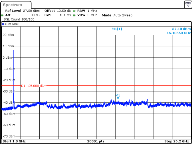
25MHz_30kHz_2607.5MHz_DFT-s-OFDM QPSK_RB64@0 -37.10 dBm
