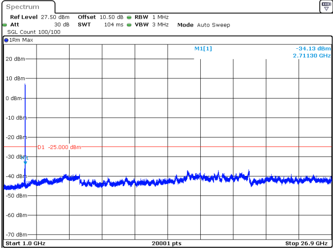
10MHz_15kHz_2685MHz_DFT-s-OFDM QPSK_RB50@0 -34.13 dBm
