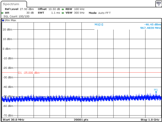
10MHz_30kHz_2595MHz_DFT-s-OFDM QPSK_RB24@0 -46.45 dBm
