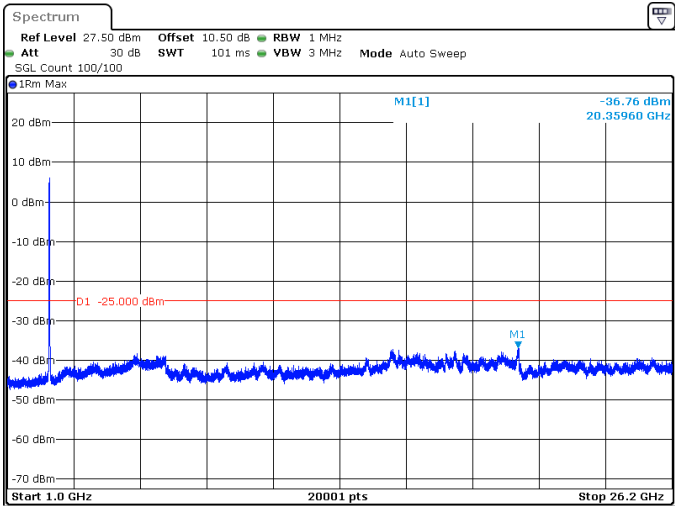
30MHz_30kHz_2585MHz_DFT-s-OFDM QPSK_RB75@0 -36.76 dBm
