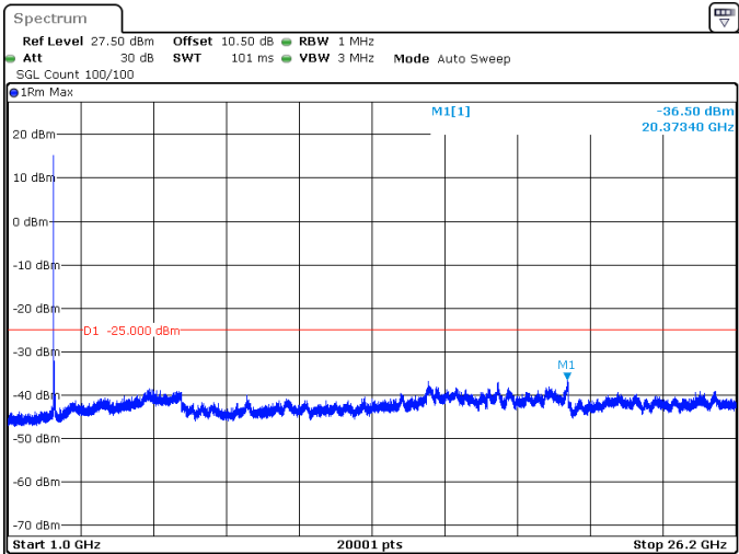
40MHz_30kHz_2590MHz_DFT-s-OFDM QPSK_RB1@0 -36.50 dBm
