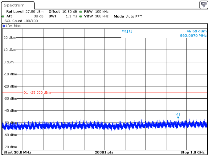
20MHz_30kHz_2610MHz_DFT-s-OFDM QPSK_RB1@0 -46.63 dBm
