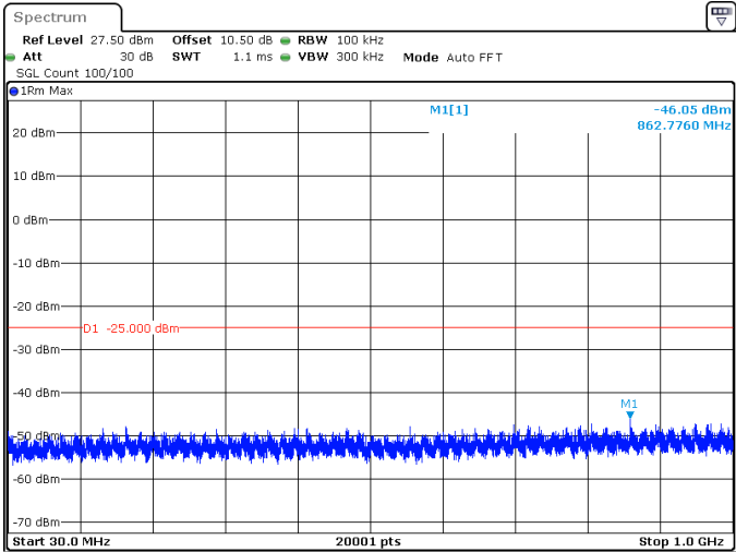
30MHz_30kHz_2595MHz_DFT-s-OFDM QPSK_RB1@77 -46.05 dBm
