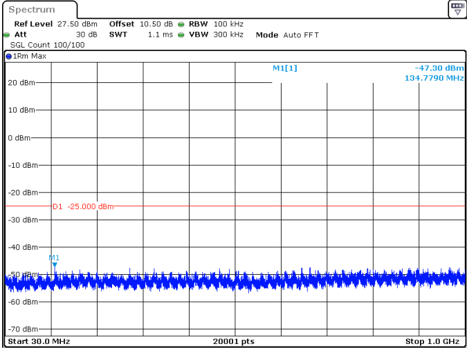
10MHz_15kHz_2685MHz_DFT-s-OFDM QPSK_RB1@51 -47.30 dBm
