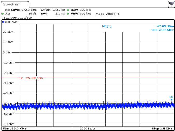
20MHz_30kHz_2610MHz_DFT-s-OFDM QPSK_RB50@0 -47.03 dBm
