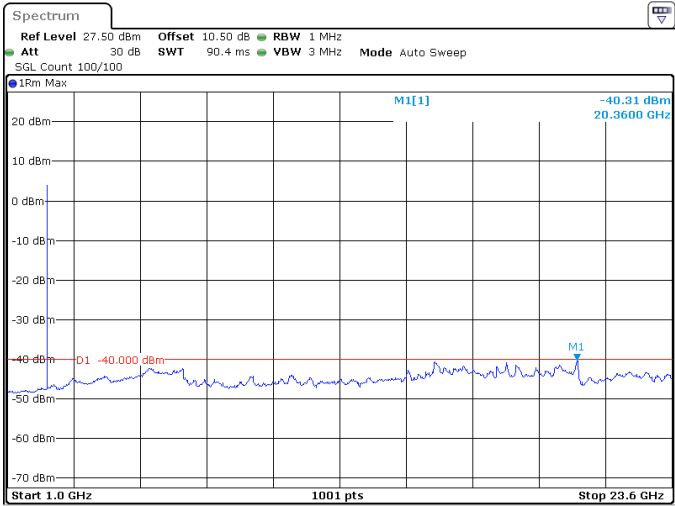
10MHz_30kHz_2355MHz_DFT-s-OFDM QPSK_RB24@0 -40.31 dBm
