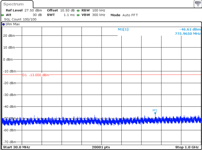
20MHz_15kHz_1720MHz_DFT-s-OFDM QPSK_RB100@0 -46.61 dBm
