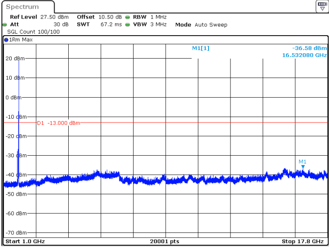
40MHz_15kHz_1760MHz_DFT-s-OFDM QPSK_RB1@215 -36.58 dBm
