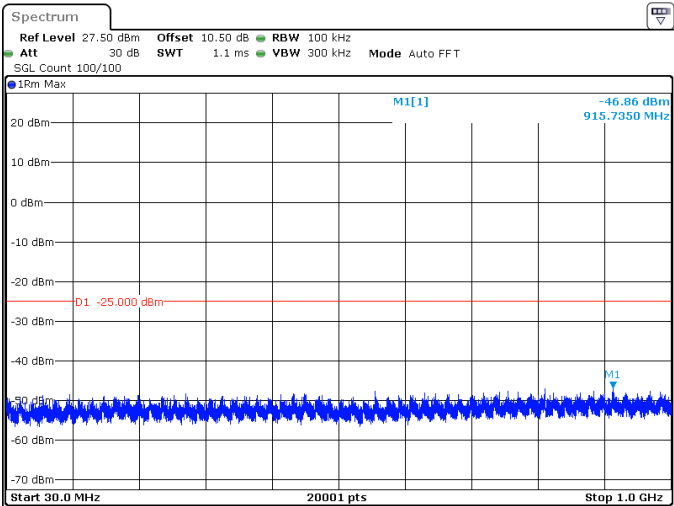
90MHz_30kHz_2541MHz_DFT-s-OFDM QPSK_RB1@0 -46.86 dBm
