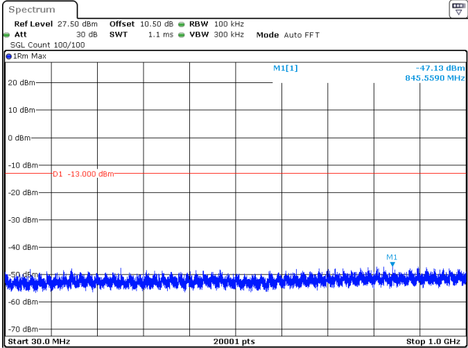
10MHz_15kHz_1745MHz_DFT-s-OFDM QPSK_RB50@0 -47.13 dBm
