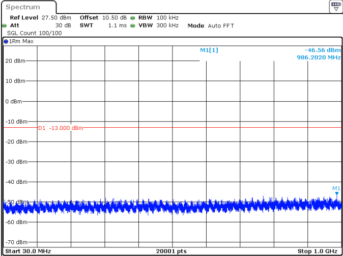
10MHz_15kHz_1775MHz_DFT-s-OFDM QPSK_RB50@0 -46.56 dBm
