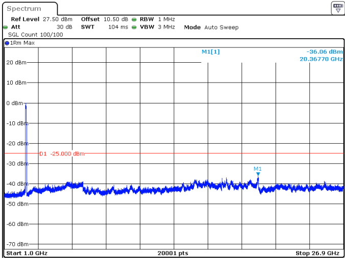
90MHz_30kHz_2644.98MHz_DFT-s-OFDM QPSK_RB243@0 -36.06 dBm
