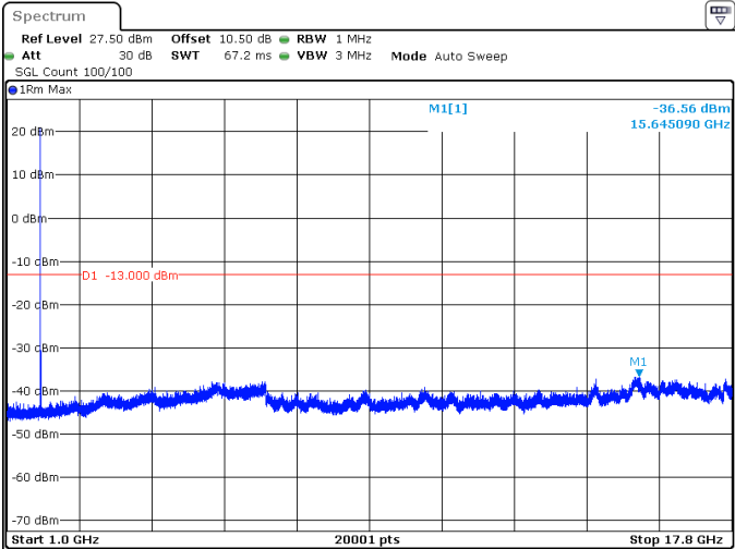
10MHz_15kHz_1775MHz_DFT-s-OFDM QPSK_RB1@0 -36.56 dBm
