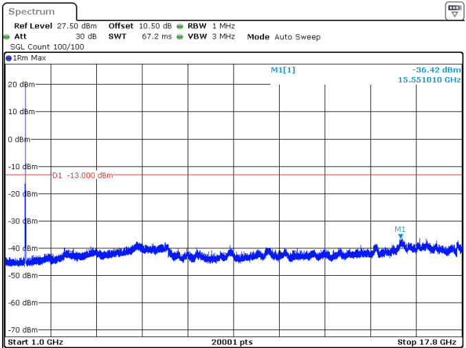
20MHz_15kHz_1745MHz_DFT-s-OFDM QPSK_RB1@0 -36.42 dBm
