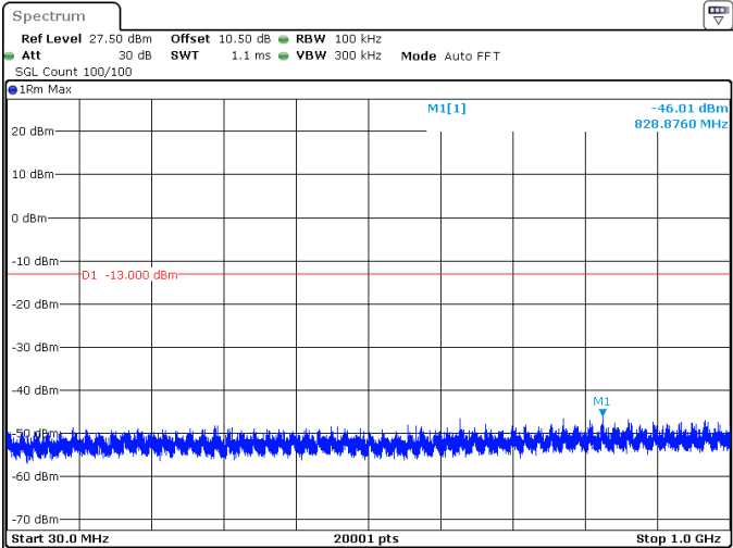
20MHz_15kHz_1720MHz_DFT-s-OFDM QPSK_RB1@0 -46.01 dBm
