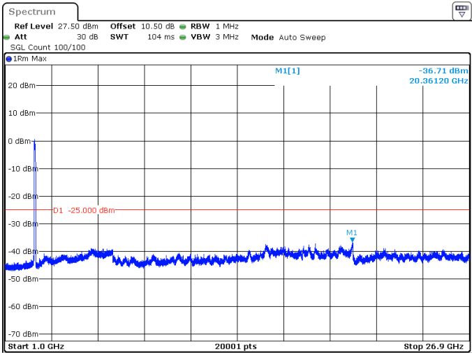
80MHz_30kHz_2649.99MHz_DFT-s-OFDM QPSK_RB216@0 -36.71 dBm
