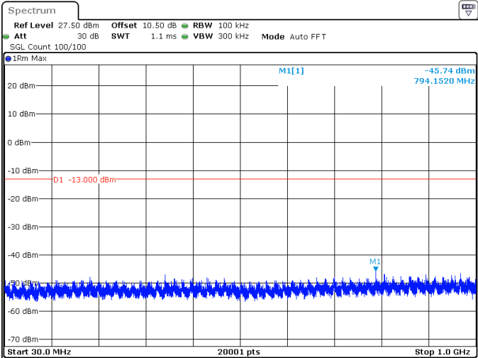
20MHz_15kHz_1770MHz_DFT-s-OFDM QPSK_RB1@0 -45.74 dBm
