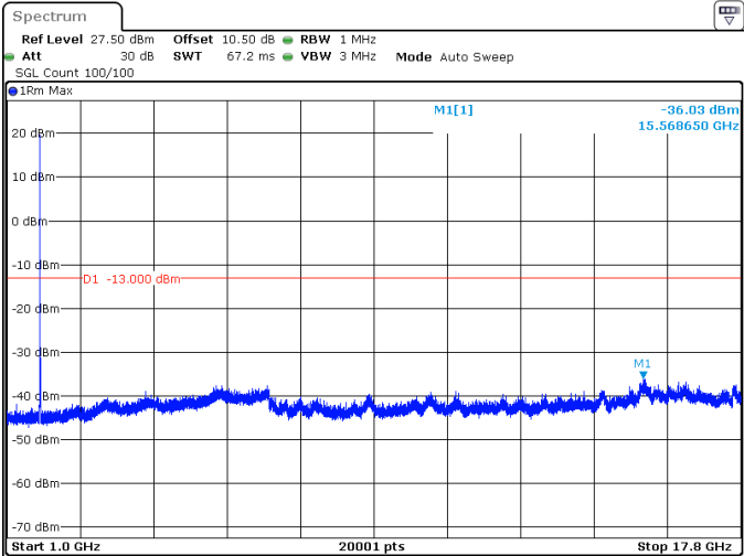
10MHz_15kHz_1745MHz_DFT-s-OFDM QPSK_RB1@0 -36.03 dBm
