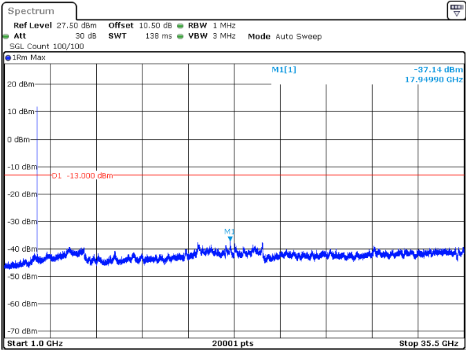
10MHz_30kHz_3455MHz_DFT-s-OFDM QPSK_RB1@23 -37.14 dBm
