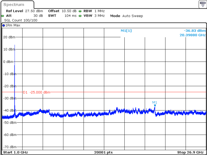
100MHz_30kHz_2640MHz_DFT-s-OFDM QPSK_RB1@0 -36.83 dBm
