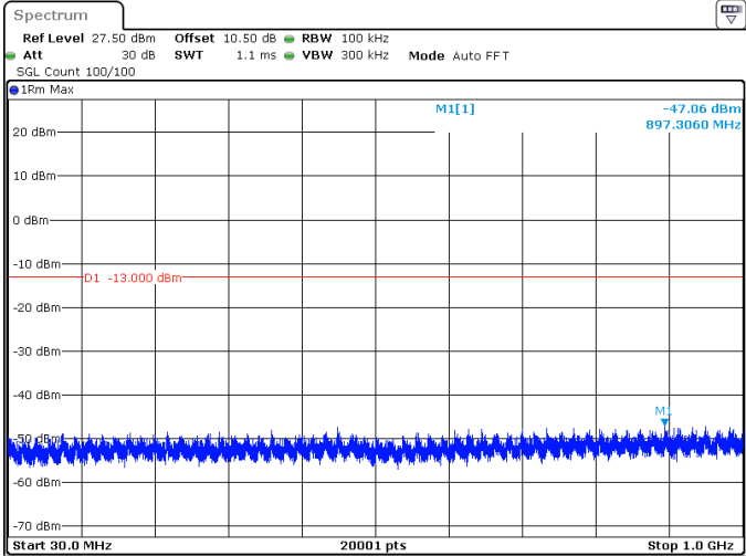
40MHz_15kHz_1760MHz_DFT-s-OFDM QPSK_RB216@0 -47.06 dBm
