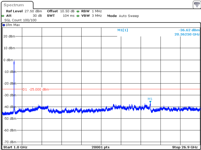
90MHz_30kHz_2541MHz_DFT-s-OFDM QPSK_RB243@0 -36.62 dBm
