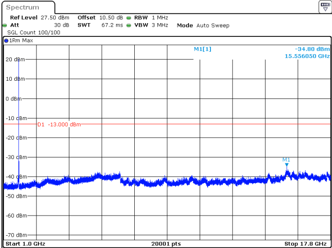
20MHz_15kHz_1770MHz_DFT-s-OFDM QPSK_RB1@0 -34.80 dBm
