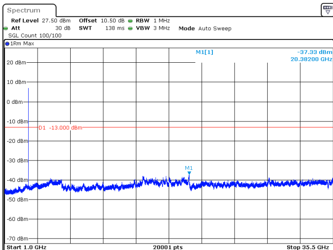
10MHz_30kHz_3500MHz_DFT-s-OFDM QPSK_RB24@0 -37.33 dBm
