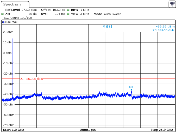
90MHz_30kHz_2644.98MHz_DFT-s-OFDM QPSK_RB1@0 -36.35 dBm
