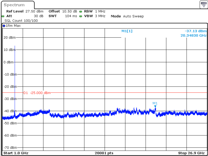
90MHz_30kHz_2541MHz_DFT-s-OFDM QPSK_RB1@244 -37.13 dBm
