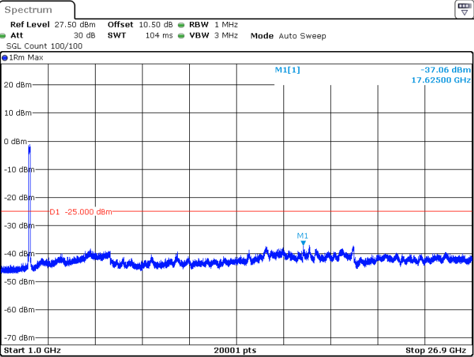
100MHz_30kHz_2546.01MHz_DFT-s-OFDM QPSK_RB270@0 -37.06 dBm
