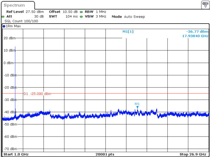
80MHz_30kHz_2649.99MHz_DFT-s-OFDM QPSK_RB1@0 -36.77 dBm
