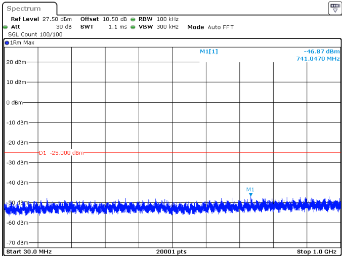
80MHz_30kHz_2649.99MHz_DFT-s-OFDM QPSK_RB1@0 -46.87 dBm
