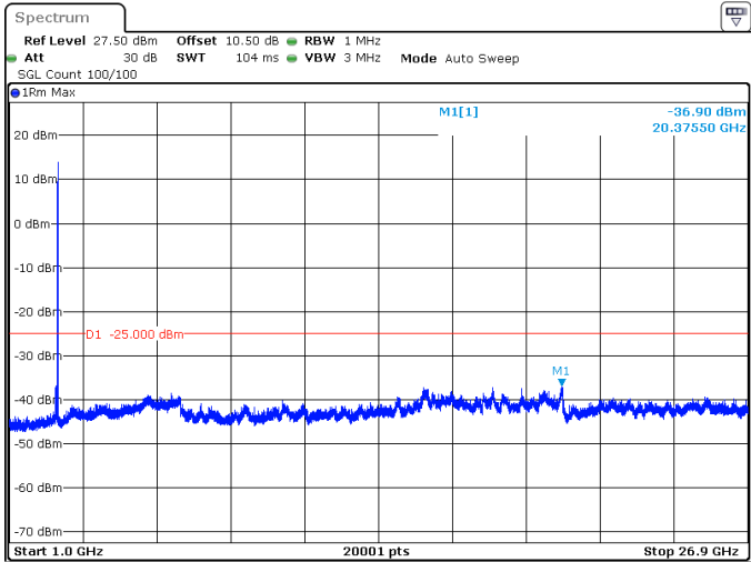
80MHz_30kHz_2649.99MHz_DFT-s-OFDM QPSK_RB1@216 -36.90 dBm
