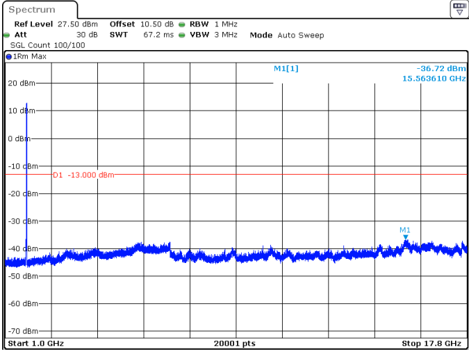
10MHz_15kHz_1775MHz_DFT-s-OFDM QPSK_RB50@0 -36.72 dBm
