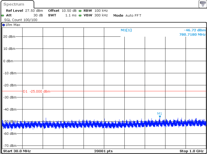
100MHz_30kHz_2640MHz_DFT-s-OFDM QPSK_RB1@272 -46.72 dBm
