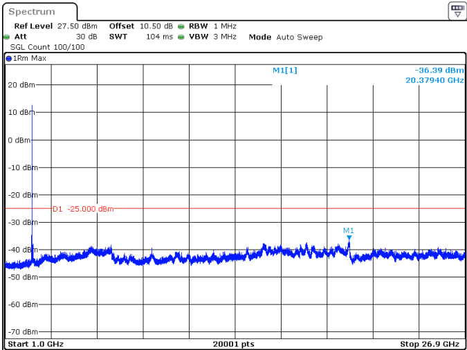
90MHz_30kHz_2541MHz_DFT-s-OFDM QPSK_RB1@0 -36.39 dBm
