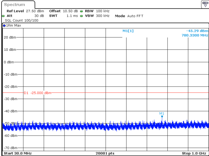
100MHz_30kHz_2640MHz_DFT-s-OFDM QPSK_RB1@0 -45.29 dBm
