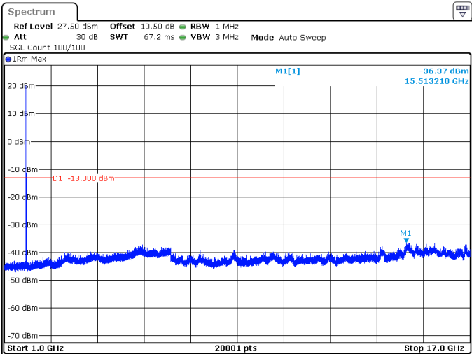
5MHz_15kHz_1777.5MHz_DFT-s-OFDM QPSK_RB1@0 -36.37 dBm
