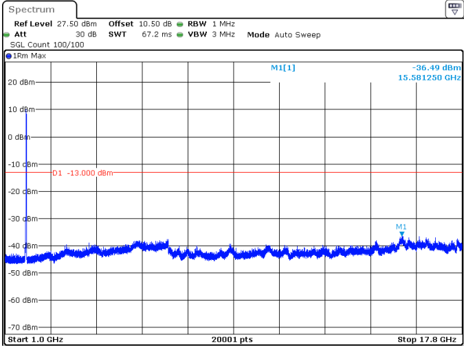
20MHz_15kHz_1770MHz_DFT-s-OFDM QPSK_RB100@0 -36.49 dBm
