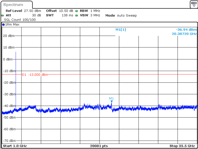
10MHz_30kHz_3455MHz_DFT-s-OFDM QPSK_RB24@0 -36.94 dBm
