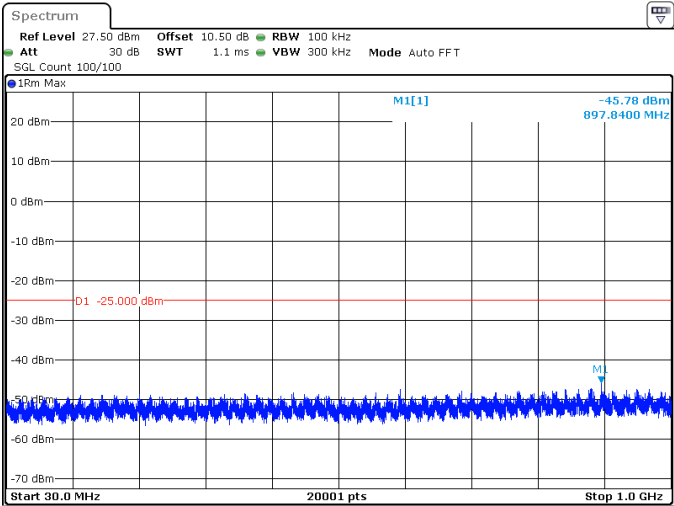
90MHz_30kHz_2541MHz_DFT-s-OFDM QPSK_RB1@244 -45.78 dBm
