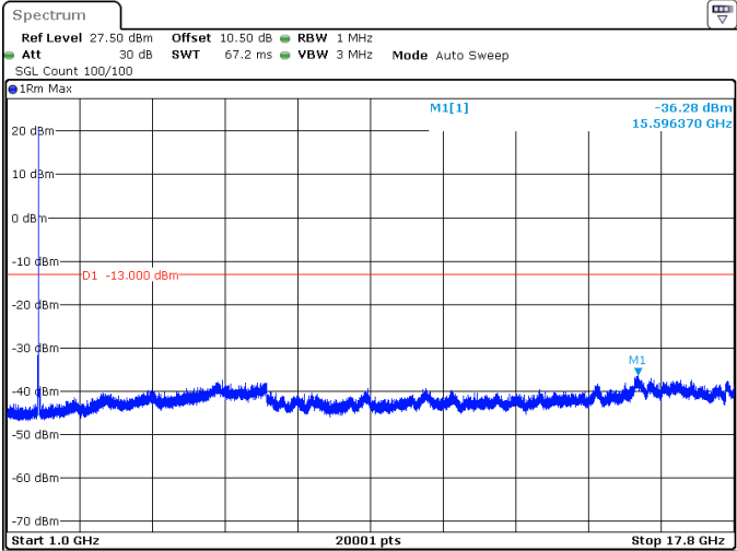
20MHz_15kHz_1720MHz_DFT-s-OFDM QPSK_RB1@105 -36.28 dBm
