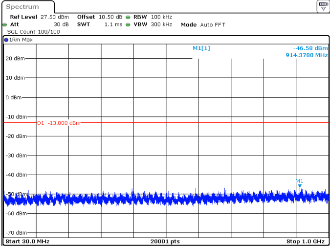
100MHz_30kHz_3500MHz_DFT-s-OFDM QPSK_RB270@0 -46.58 dBm
