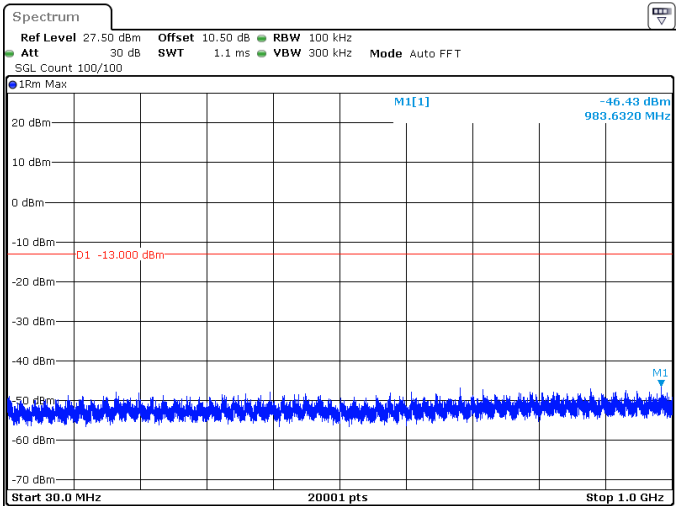
90MHz_30kHz_3500MHz_DFT-s-OFDM QPSK_RB1@0 -46.43 dBm
