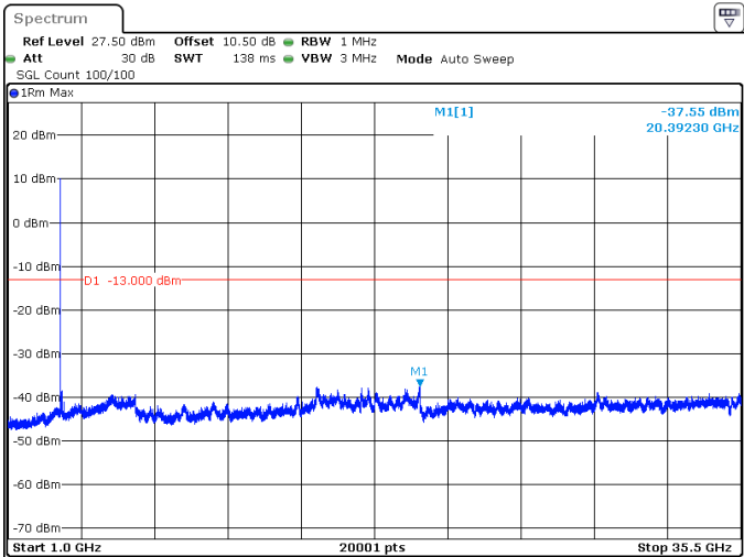
90MHz_30kHz_3495MHz_DFT-s-OFDM QPSK_RB1@0 -37.55 dBm
