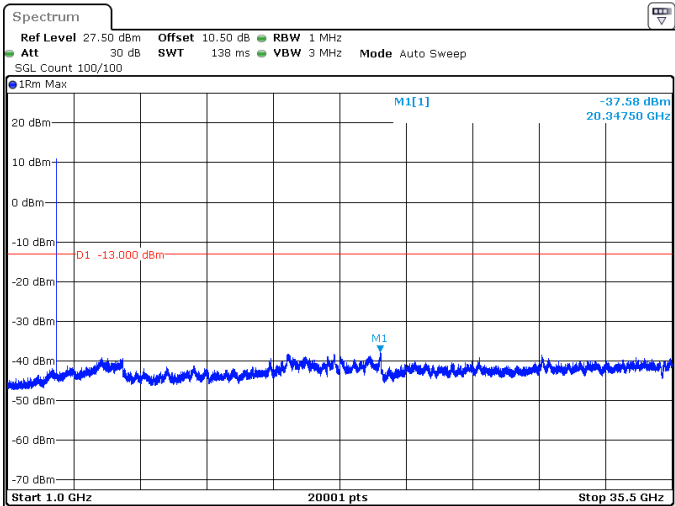
20MHz_30kHz_3540MHz_DFT-s-OFDM QPSK_RB1@0 -37.58 dBm
