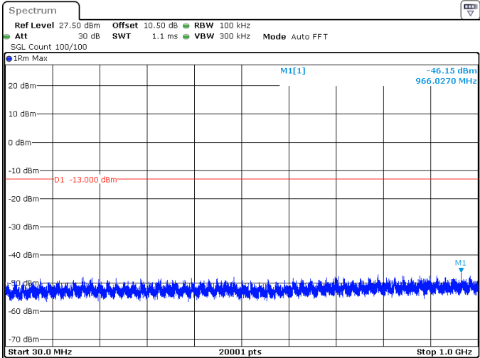
20MHz_15kHz_3710MHz_DFT-s-OFDM QPSK_RB1@0 -46.15 dBm
