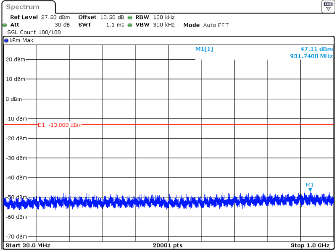
20MHz_15kHz_3710MHz_DFT-s-OFDM QPSK_RB100@0 -47.11 dBm
