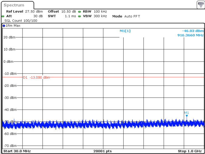
70MHz_30kHz_3485MHz_DFT-s-OFDM QPSK_RB180@0 -46.03 dBm
