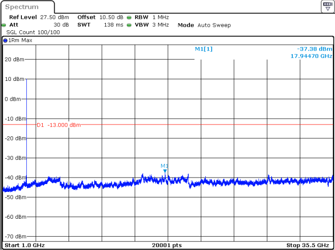
40MHz_30kHz_3470MHz_DFT-s-OFDM QPSK_RB1@105 -37.38 dBm
