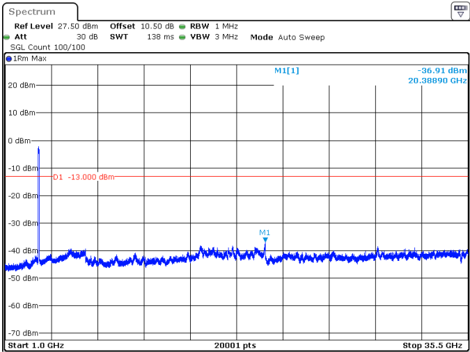
90MHz_30kHz_3495MHz_DFT-s-OFDM QPSK_RB243@0 -36.91 dBm
