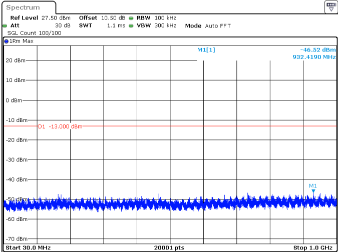
20MHz_15kHz_3840MHz_DFT-s-OFDM QPSK_RB1@0 -46.52 dBm
