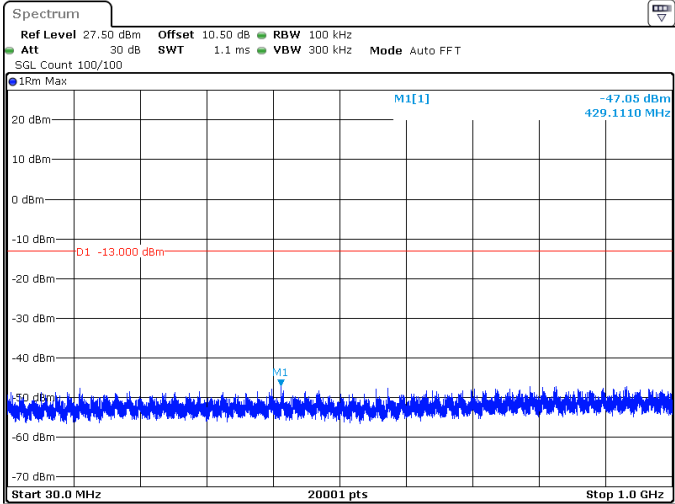
100MHz_30kHz_3500MHz_DFT-s-OFDM QPSK_RB1@272 -47.05 dBm
