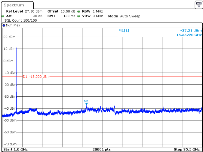
90MHz_30kHz_3505MHz_DFT-s-OFDM QPSK_RB1@0 -37.21 dBm
