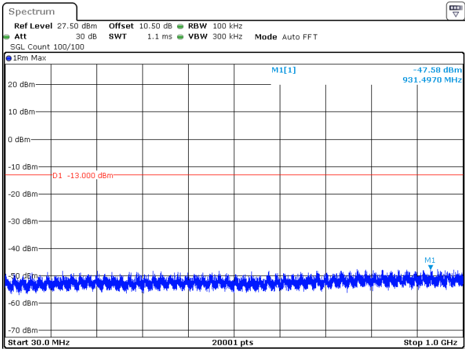
80MHz_30kHz_3510MHz_DFT-s-OFDM QPSK_RB216@0 -47.58 dBm
