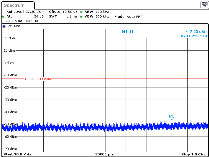
80MHz_30kHz_3500MHz_DFT-s-OFDM QPSK_RB1@0 -47.05 dBm
