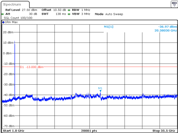
40MHz_30kHz_3530MHz_DFT-s-OFDM QPSK_RB1@0 -36.97 dBm
