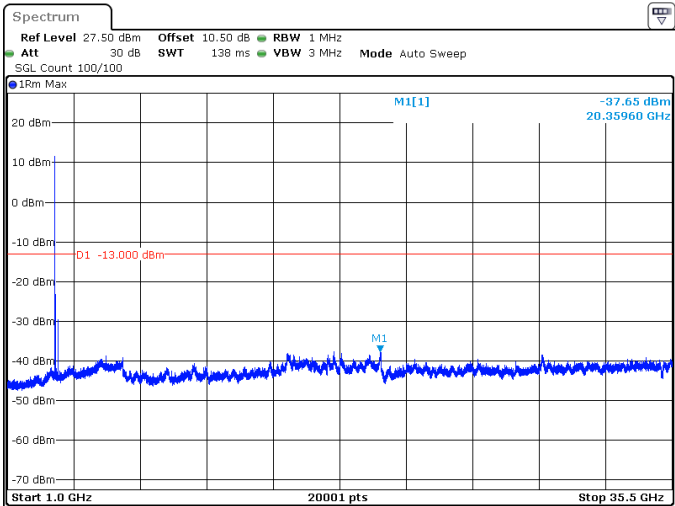
70MHz_30kHz_3500MHz_DFT-s-OFDM QPSK_RB1@0 -37.65 dBm
