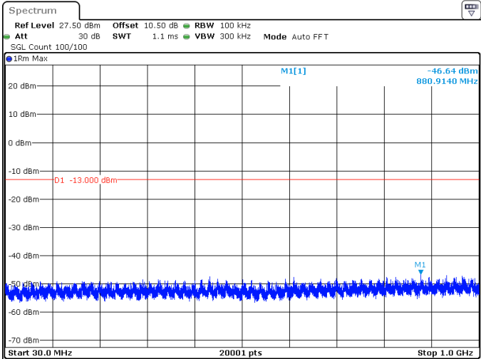
100MHz_30kHz_3500MHz_DFT-s-OFDM QPSK_RB1@0 -46.64 dBm
