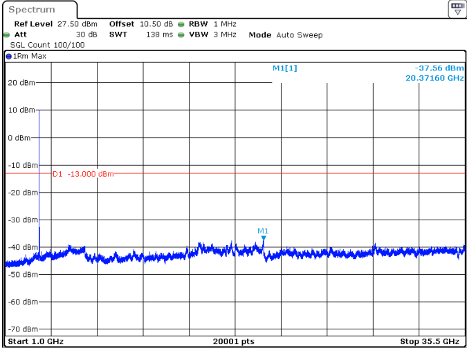
60MHz_30kHz_3520MHz_DFT-s-OFDM QPSK_RB1@161 -37.56 dBm
