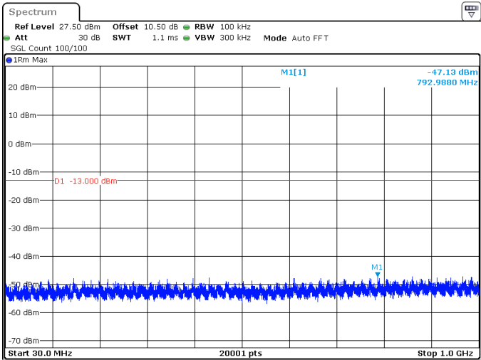
90MHz_30kHz_3505MHz_DFT-s-OFDM QPSK_RB243@0 -47.13 dBm
