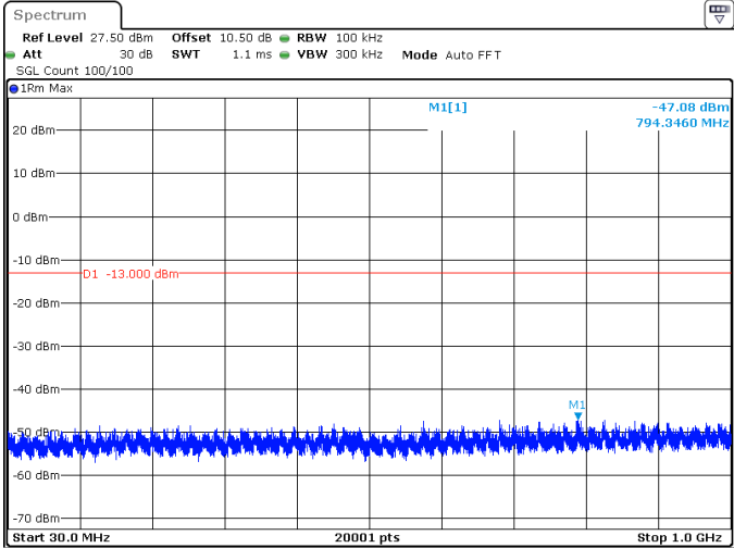
20MHz_15kHz_3710MHz_DFT-s-OFDM QPSK_RB1@105 -47.08 dBm
