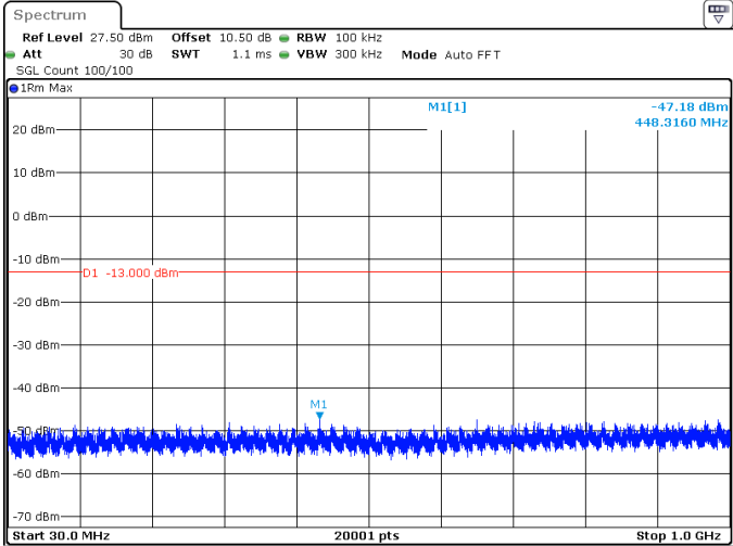
10MHz_30kHz_3840MHz_DFT-s-OFDM QPSK_RB24@0 -47.18 dBm
