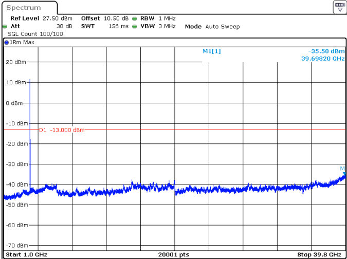
10MHz_15kHz_3975MHz_DFT-s-OFDM QPSK_RB1@0 -35.50 dBm
