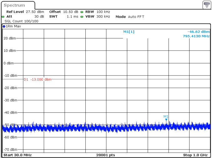
90MHz_30kHz_3500MHz_DFT-s-OFDM QPSK_RB243@0 -46.62 dBm
