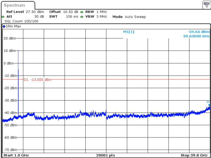
10MHz_30kHz_3975MHz_DFT-s-OFDM QPSK_RB1@0 -34.65 dBm
