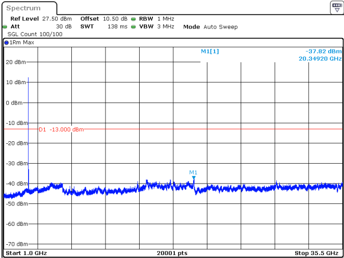
20MHz_30kHz_3500MHz_DFT-s-OFDM QPSK_RB1@50 -37.82 dBm
