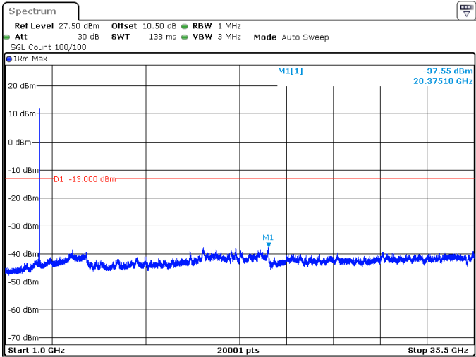
70MHz_30kHz_3485MHz_DFT-s-OFDM QPSK_RB1@188 -37.55 dBm
