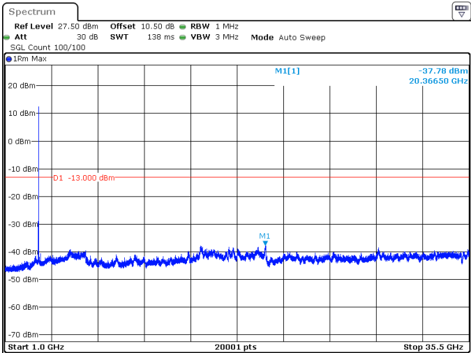
80MHz_30kHz_3510MHz_DFT-s-OFDM QPSK_RB1@0 -37.78 dBm
