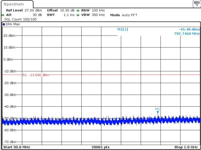
60MHz_30kHz_3480MHz_DFT-s-OFDM QPSK_RB1@161 -45.48 dBm
