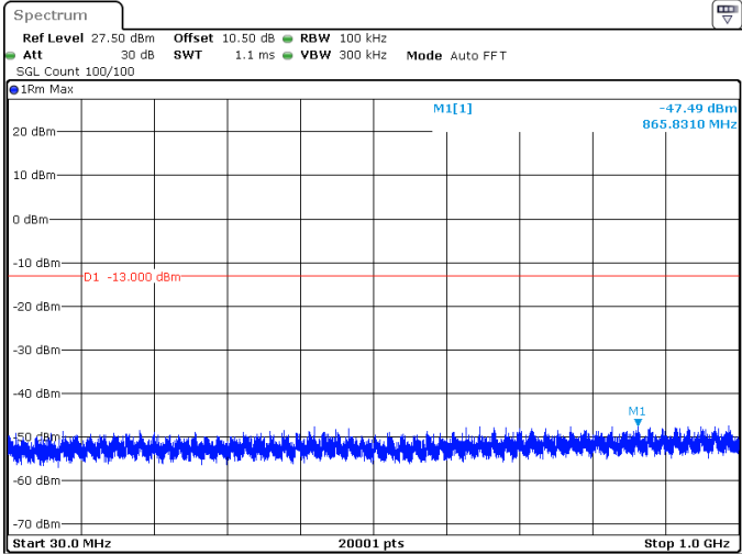
60MHz_30kHz_3500MHz_DFT-s-OFDM QPSK_RB1@161 -47.49 dBm
