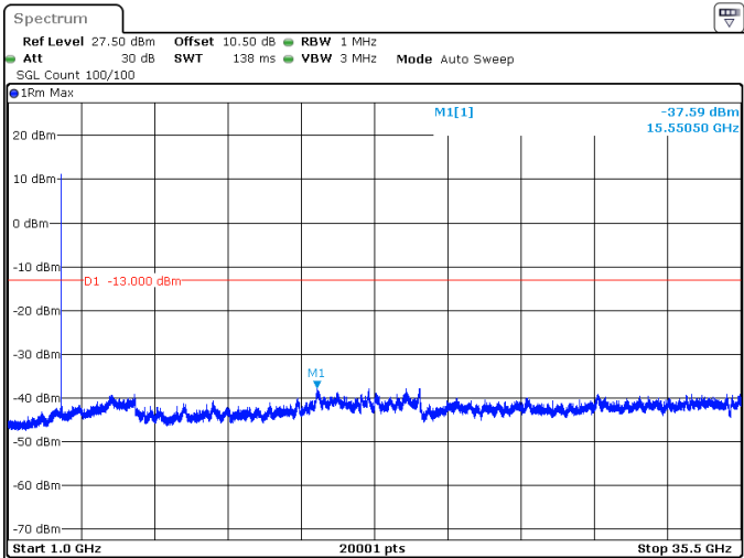
20MHz_30kHz_3500MHz_DFT-s-OFDM QPSK_RB1@0 -37.59 dBm
