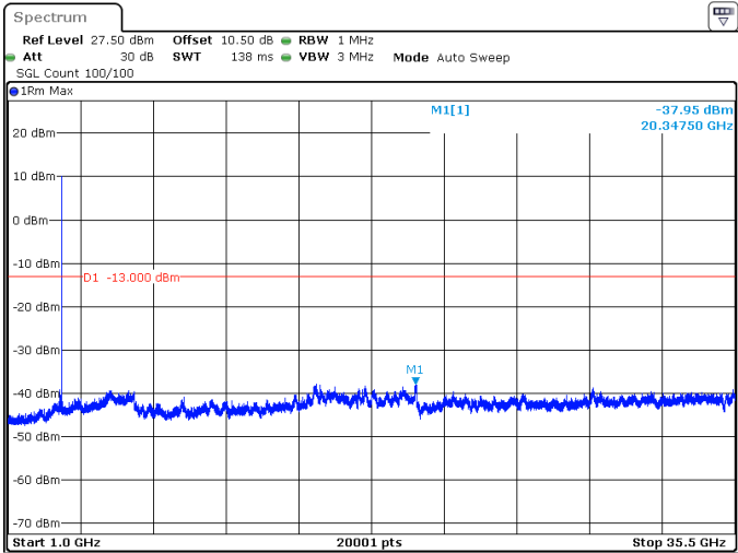
80MHz_30kHz_3500MHz_DFT-s-OFDM QPSK_RB1@216 -37.95 dBm
