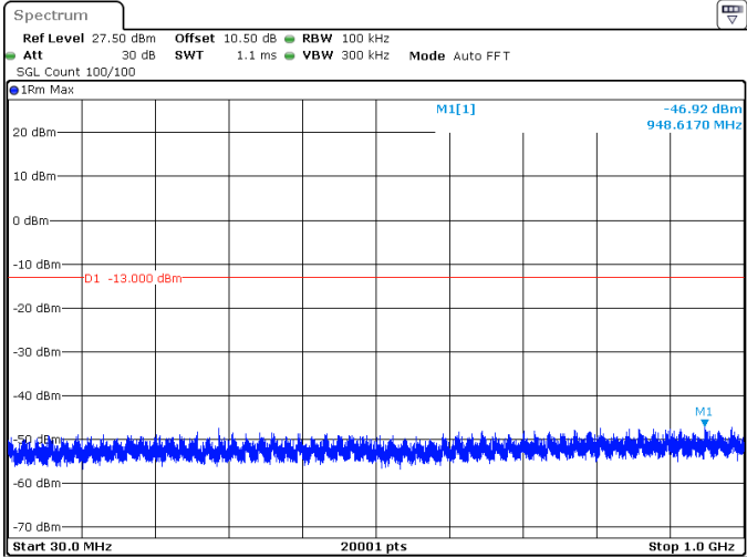
10MHz_15kHz_3975MHz_DFT-s-OFDM QPSK_RB50@0 -46.92 dBm
