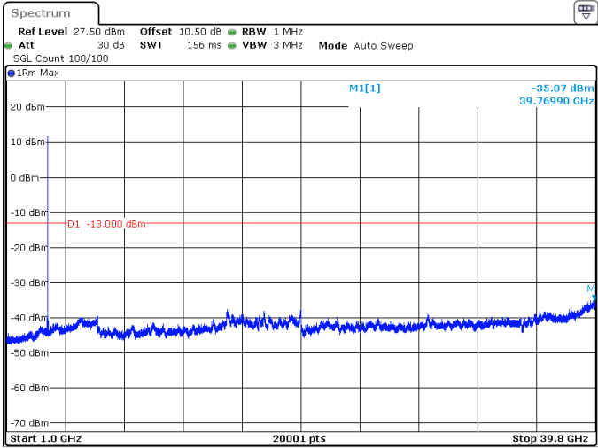
10MHz_15kHz_3705MHz_DFT-s-OFDM QPSK_RB1@0 -35.07 dBm
