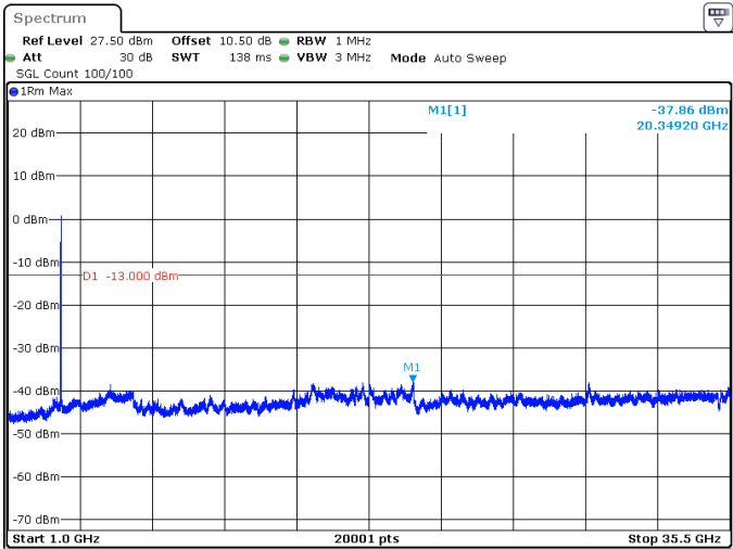
40MHz_30kHz_3530MHz_DFT-s-OFDM QPSK_RB100@0 -37.86 dBm
