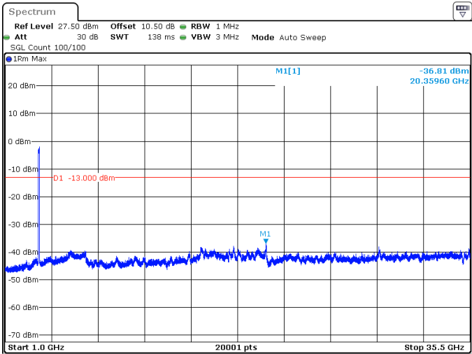
80MHz_30kHz_3490MHz_DFT-s-OFDM QPSK_RB216@0 -36.81 dBm
