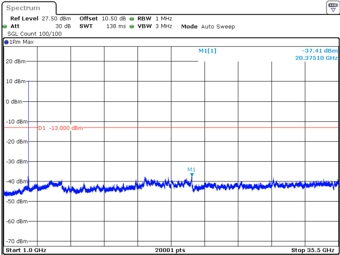
80MHz_30kHz_3510MHz_DFT-s-OFDM QPSK_RB1@216 -37.41 dBm
