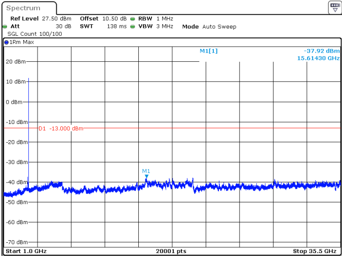
80MHz_30kHz_3490MHz_DFT-s-OFDM QPSK_RB1@216 -37.92 dBm
