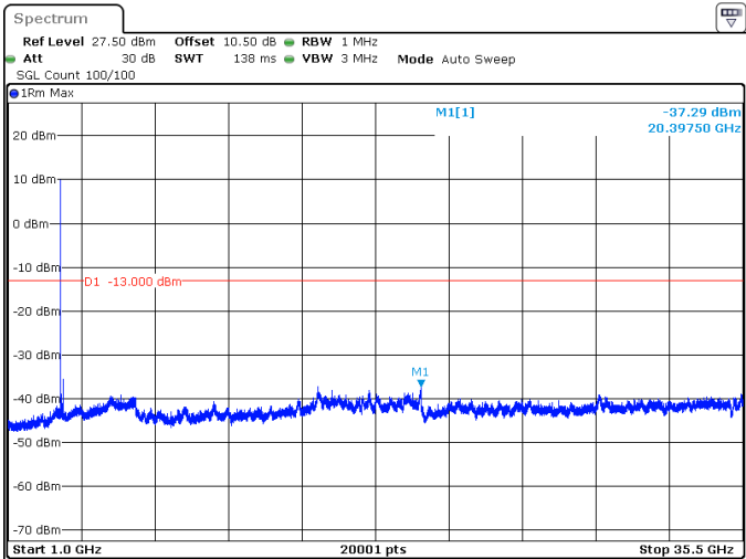
70MHz_30kHz_3485MHz_DFT-s-OFDM QPSK_RB1@0 -37.29 dBm
