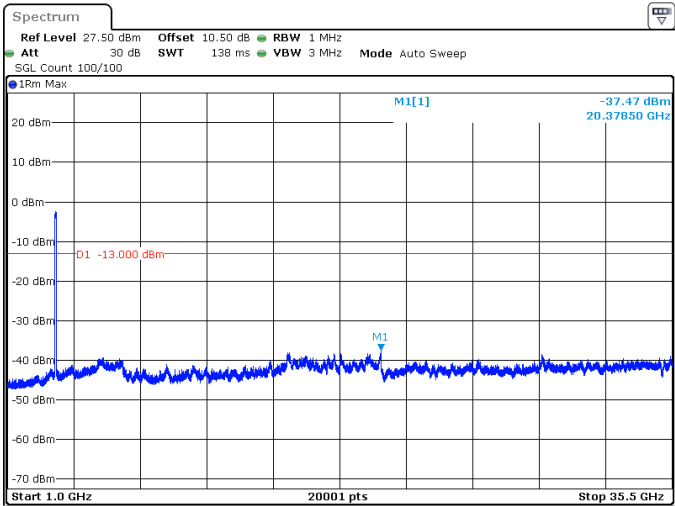
80MHz_30kHz_3500MHz_DFT-s-OFDM QPSK_RB216@0 -37.47 dBm
