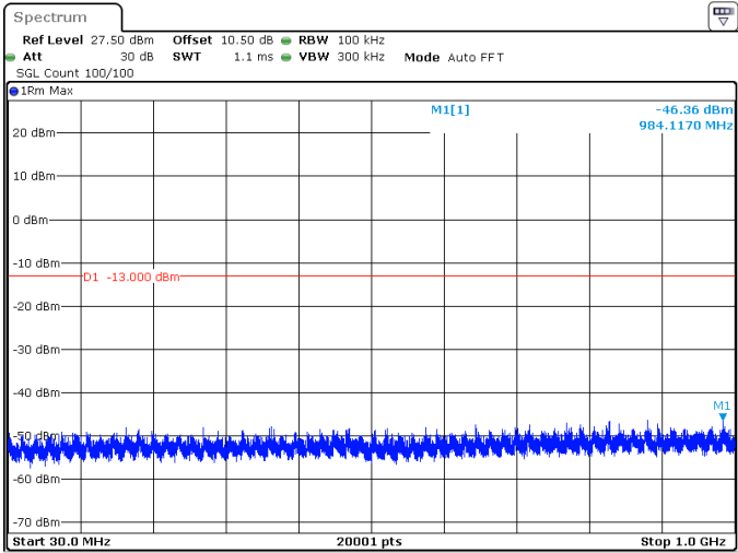
10MHz_15kHz_3705MHz_DFT-s-OFDM QPSK_RB50@0 -46.36 dBm
