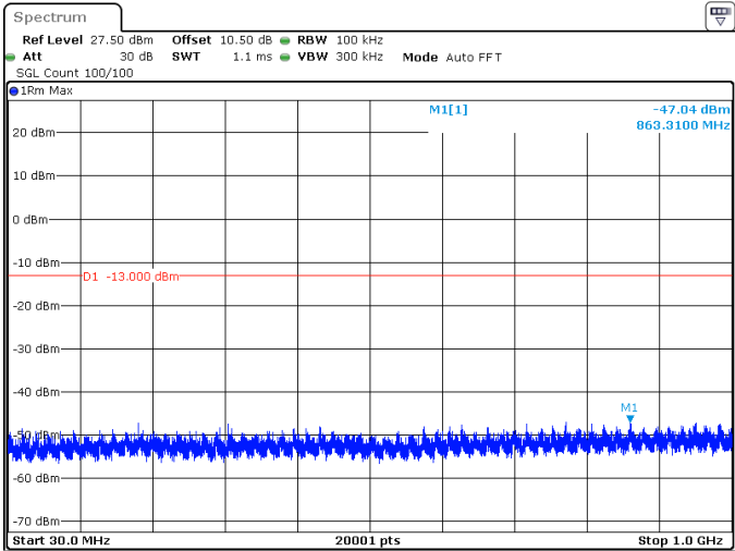
20MHz_30kHz_3540MHz_DFT-s-OFDM QPSK_RB1@50 -47.04 dBm
