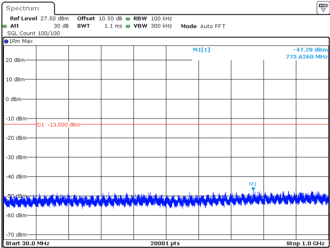
10MHz_15kHz_3840MHz_DFT-s-OFDM QPSK_RB50@0 -47.28 dBm
