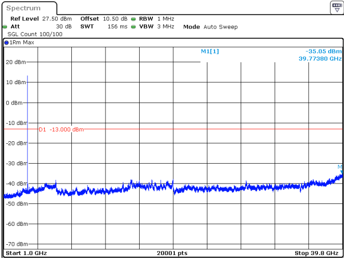
10MHz_15kHz_3705MHz_DFT-s-OFDM QPSK_RB1@51 -35.05 dBm
