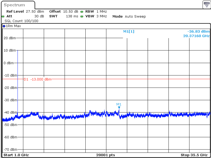
90MHz_30kHz_3495MHz_DFT-s-OFDM QPSK_RB1@244 -36.83 dBm
