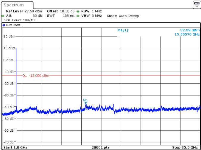
80MHz_30kHz_3490MHz_DFT-s-OFDM QPSK_RB1@0 -37.39 dBm
