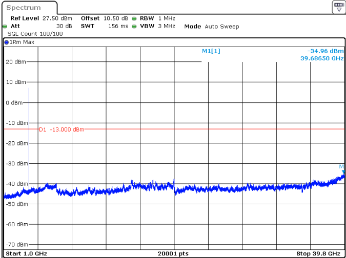
10MHz_30kHz_3840MHz_DFT-s-OFDM QPSK_RB1@0 -34.96 dBm
