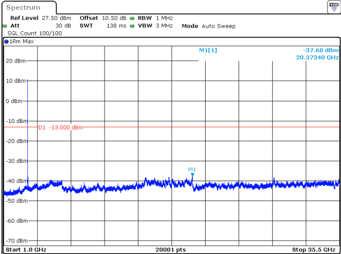
20MHz_30kHz_3460MHz_DFT-s-OFDM QPSK_RB1@0 -37.60 dBm
