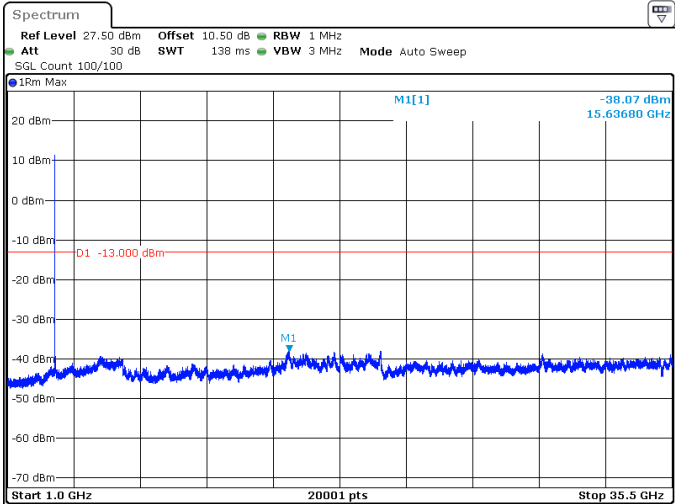
60MHz_30kHz_3480MHz_DFT-s-OFDM QPSK_RB1@0 -38.07 dBm
