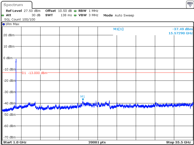
70MHz_30kHz_3500MHz_DFT-s-OFDM QPSK_RB180@0 -37.49 dBm
