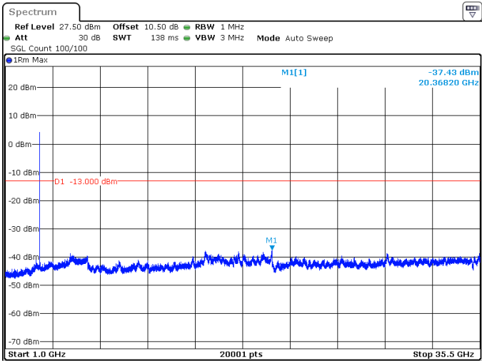
20MHz_30kHz_3500MHz_DFT-s-OFDM QPSK_RB50@0 -37.43 dBm
