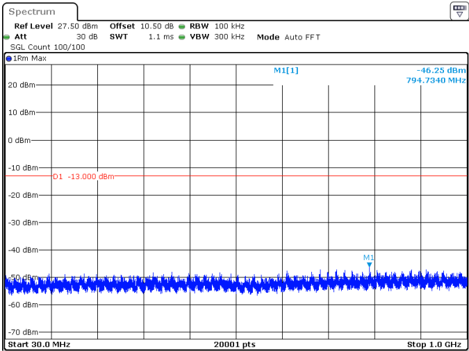
20MHz_30kHz_3540MHz_DFT-s-OFDM QPSK_RB50@0 -46.25 dBm
