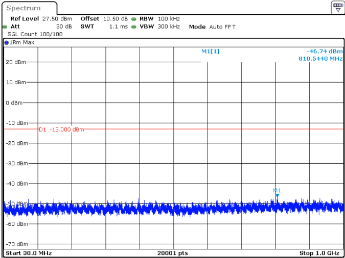
10MHz_30kHz_3975MHz_DFT-s-OFDM QPSK_RB1@23 -46.74 dBm
