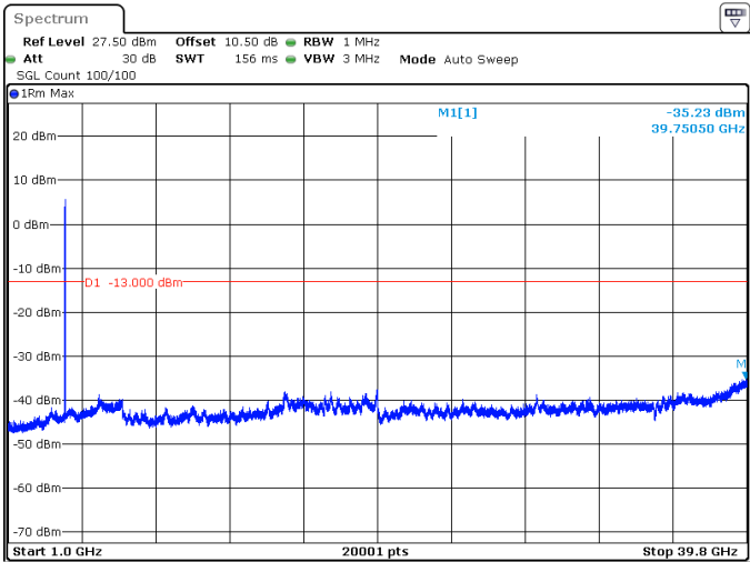
10MHz_30kHz_3975MHz_DFT-s-OFDM QPSK_RB24@0 -35.23 dBm
