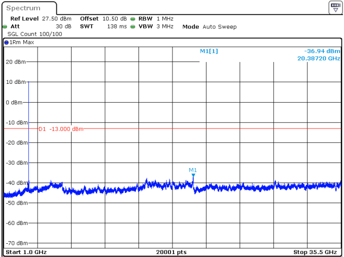
90MHz_30kHz_3500MHz_DFT-s-OFDM QPSK_RB1@244 -36.94 dBm
