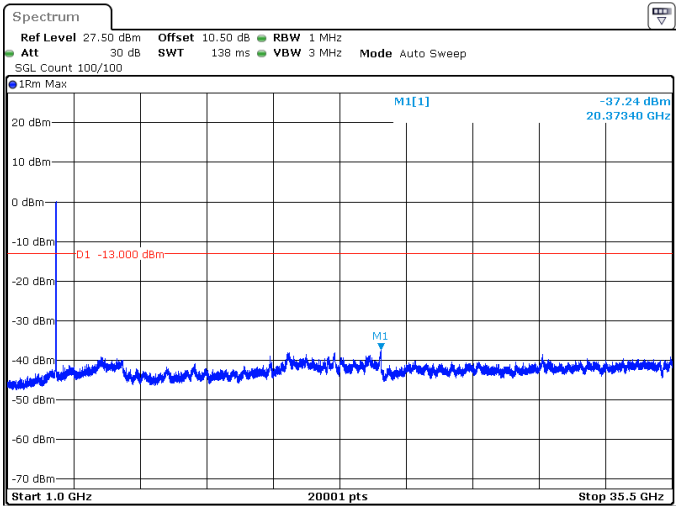
50MHz_30kHz_3500MHz_DFT-s-OFDM QPSK_RB128@0 -37.24 dBm
