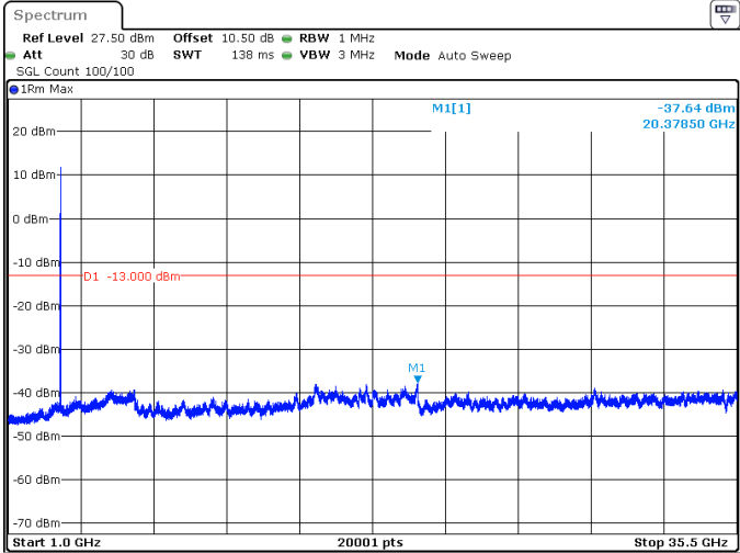
20MHz_30kHz_3460MHz_DFT-s-OFDM QPSK_RB1@50 -37.64 dBm
