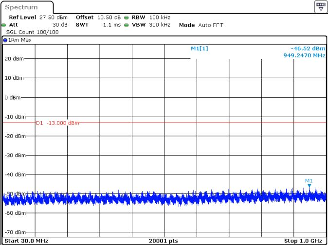
40MHz_30kHz_3470MHz_DFT-s-OFDM QPSK_RB1@0 -46.52 dBm
