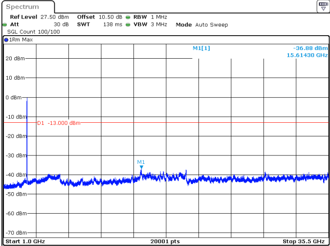
60MHz_30kHz_3480MHz_DFT-s-OFDM QPSK_RB162@0 -36.88 dBm
