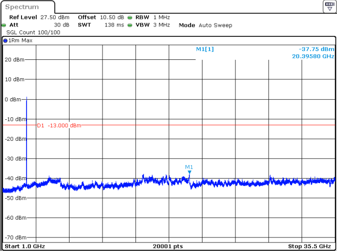
40MHz_30kHz_3470MHz_DFT-s-OFDM QPSK_RB100@0 -37.75 dBm
