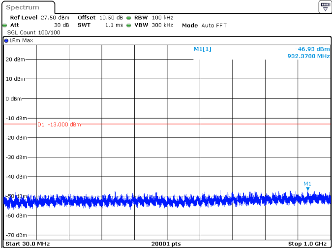
60MHz_30kHz_3520MHz_DFT-s-OFDM QPSK_RB1@0 -46.93 dBm
