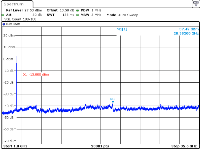
20MHz_30kHz_3460MHz_DFT-s-OFDM QPSK_RB50@0 -37.49 dBm
