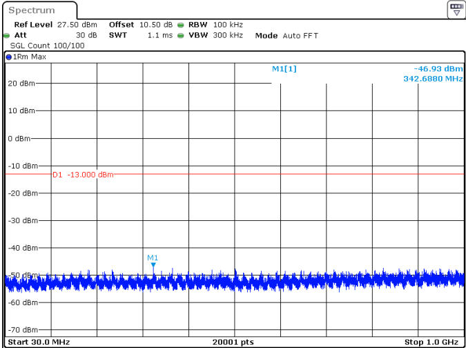
60MHz_30kHz_3500MHz_DFT-s-OFDM QPSK_RB1@0 -46.93 dBm
