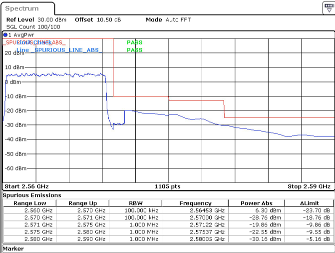
10MHz_15kHz_2565MHz_DFT-s-OFDM QPSK_RB50@0 -30.16 dBm
