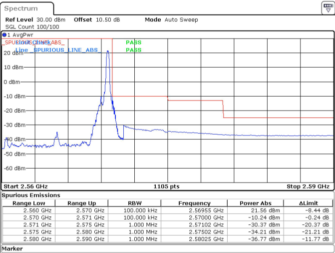
10MHz_15kHz_2565MHz_DFT-s-OFDM QPSK_RB1@51 -10.24 dBm
