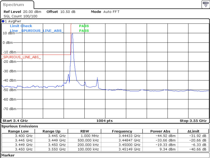
20MHz_30kHz_3460MHz_DFT-s-OFDM QPSK_RB1@0 -19.33 dBm
