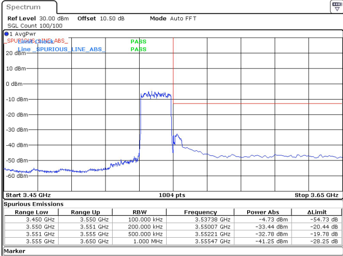
20MHz_30kHz_3540MHz_DFT-s-OFDM QPSK_RB50@0 -32.78 dBm
