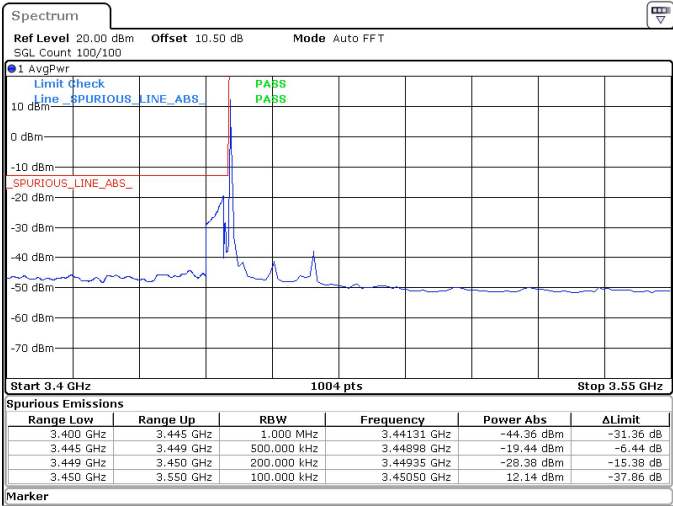
20MHz_15kHz_3460MHz_DFT-s-OFDM QPSK_RB1@0 -19.44 dBm
