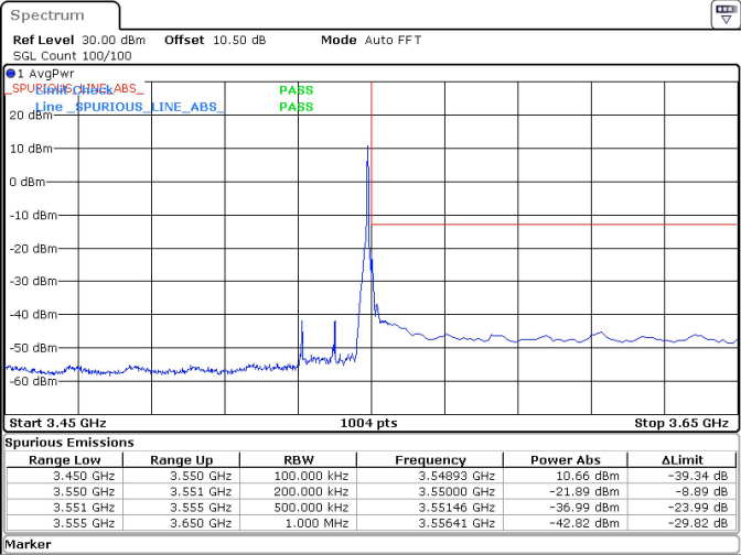
20MHz_30kHz_3540MHz_DFT-s-OFDM QPSK_RB1@50 -21.89 dBm
