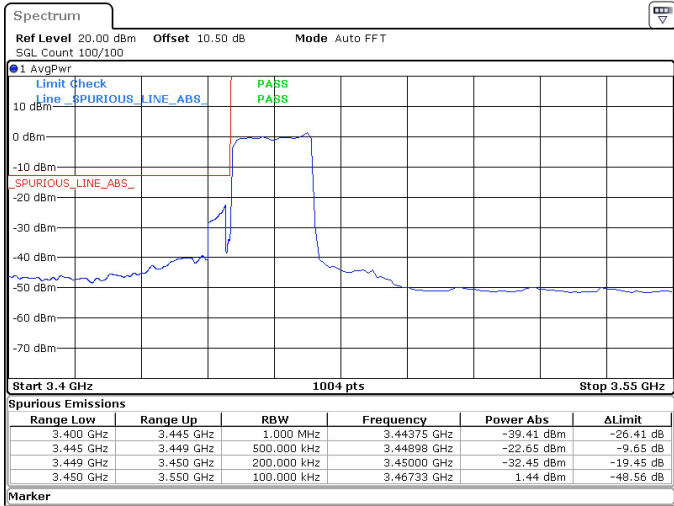
20MHz_15kHz_3460MHz_DFT-s-OFDM QPSK_RB100@0 -22.65 dBm
