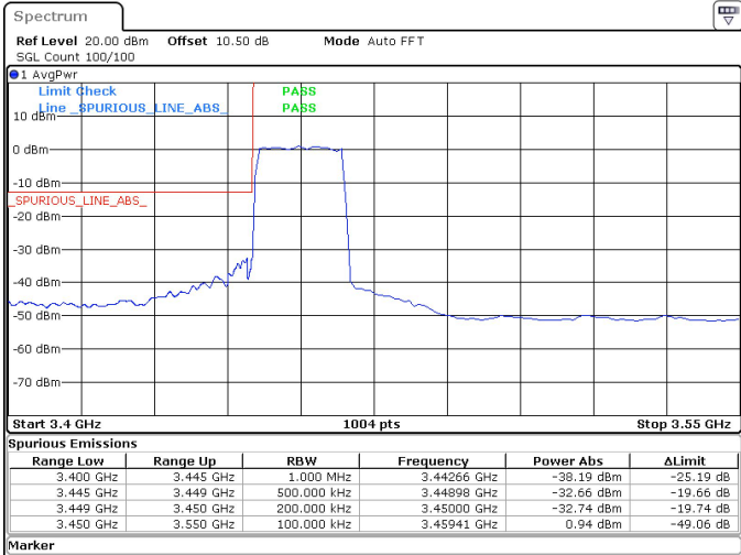
20MHz_30kHz_3460MHz_DFT-s-OFDM QPSK_RB50@0 -32.66 dBm
