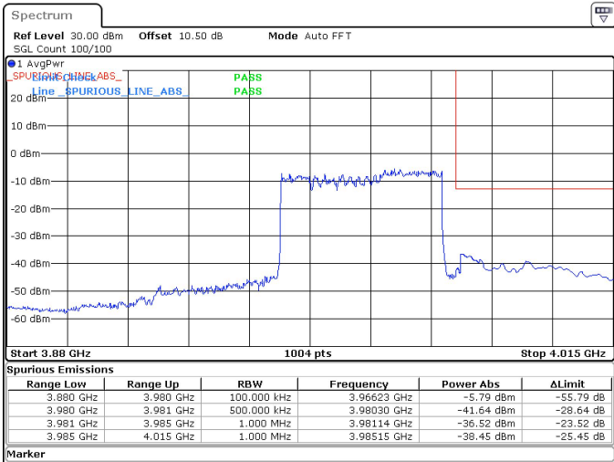
40MHz_30kHz_3960MHz_DFT-s-OFDM QPSK_RB100@0 -36.52 dBm
