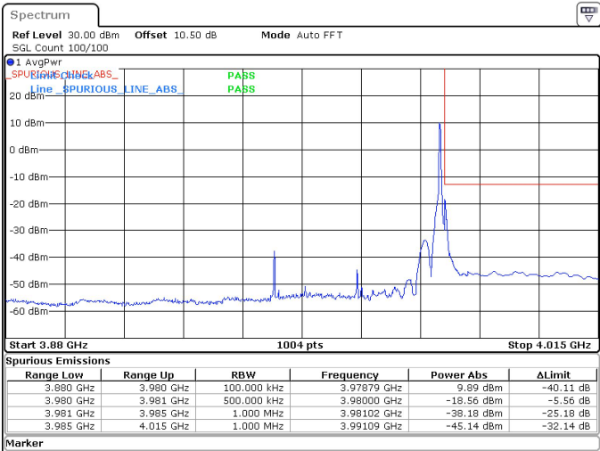
40MHz_30kHz_3960MHz_DFT-s-OFDM QPSK_RB1@105 -18.56 dBm
