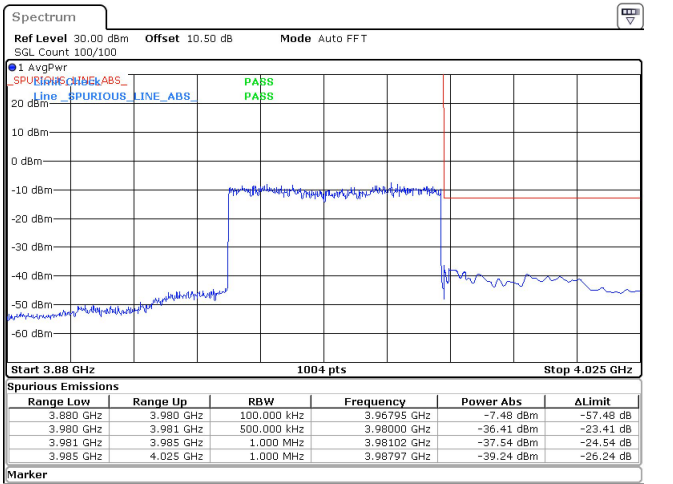
50MHz_15kHz_3955MHz_DFT-s-OFDM QPSK_RB270@0 -36.41 dBm
