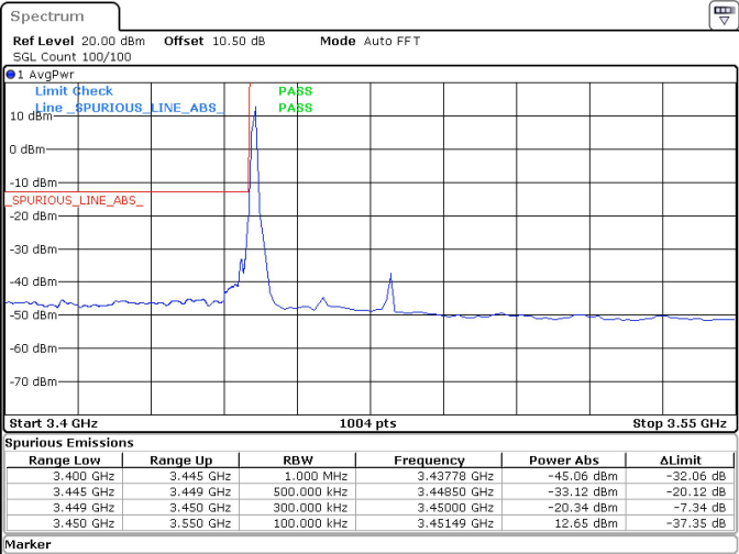
30MHz_30kHz_3465MHz_DFT-s-OFDM QPSK_RB1@0 -20.34 dBm
