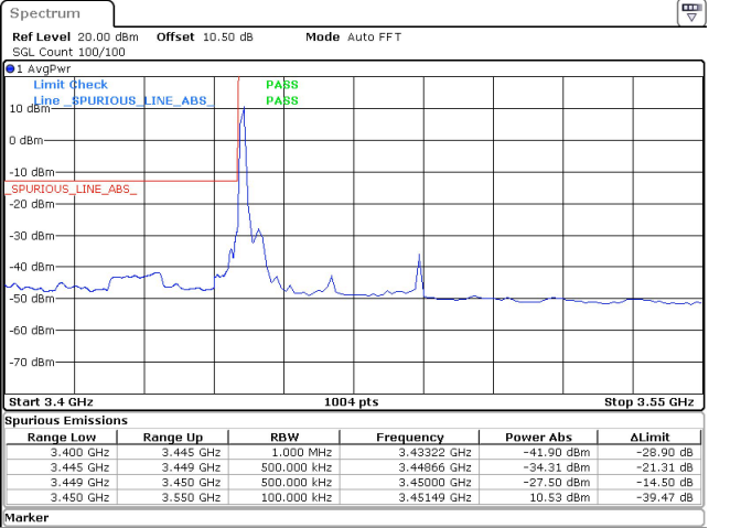
40MHz_30kHz_3470MHz_DFT-s-OFDM QPSK_RB1@0 -27.50 dBm
