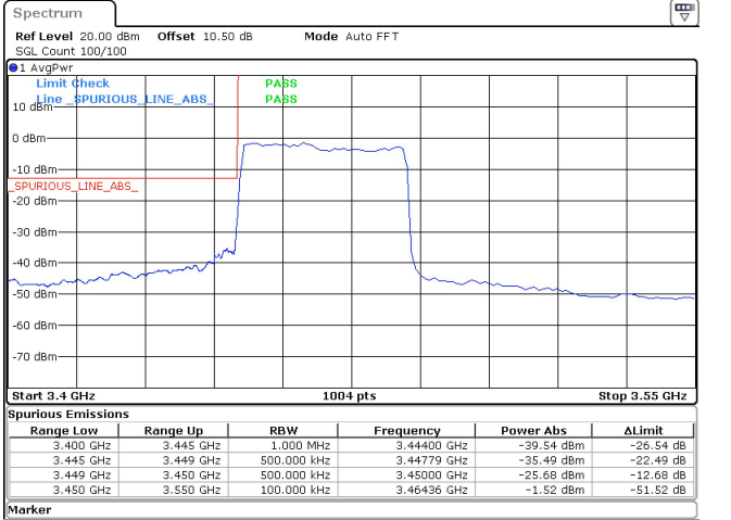
40MHz_30kHz_3470MHz_DFT-s-OFDM QPSK_RB100@0 -25.68 dBm
