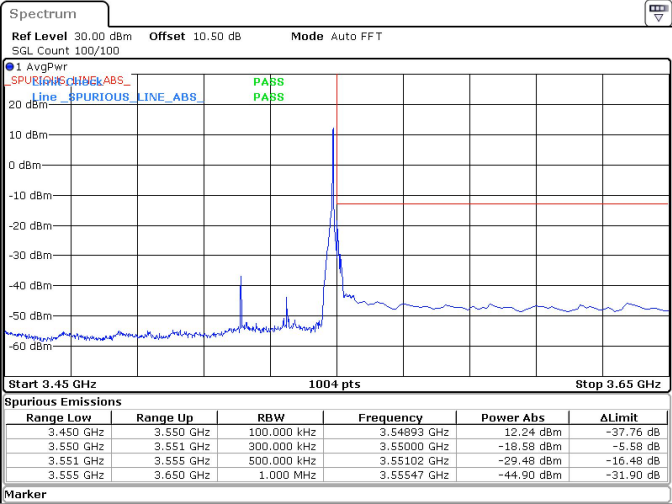
30MHz_30kHz_3535MHz_DFT-s-OFDM QPSK_RB1@77 -18.58 dBm
