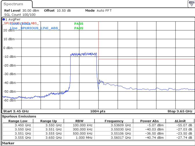
30MHz_30kHz_3535MHz_DFT-s-OFDM QPSK_RB75@0 -36.50 dBm
