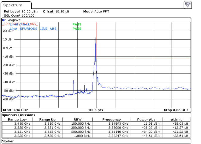
25MHz_30kHz_3537.5MHz_DFT-s-OFDM QPSK_RB1@64 -25.27 dBm
