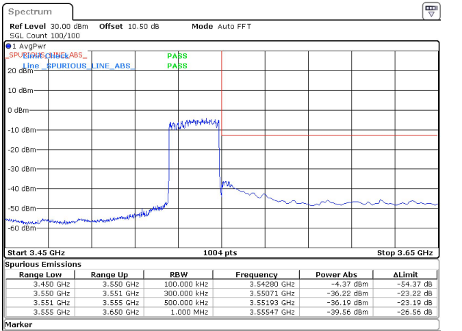
25MHz_30kHz_3537.5MHz_DFT-s-OFDM QPSK_RB64@0 -36.19 dBm
