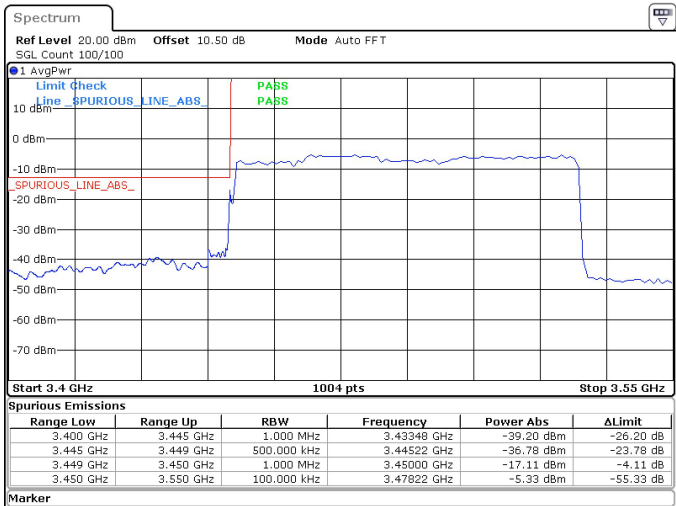
80MHz_30kHz_3490MHz_DFT-s-OFDM QPSK_RB216@0 -17.11 dBm
