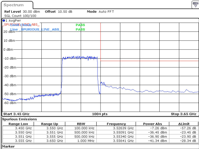
40MHz_30kHz_3530MHz_DFT-s-OFDM QPSK_RB100@0 -36.45 dBm
