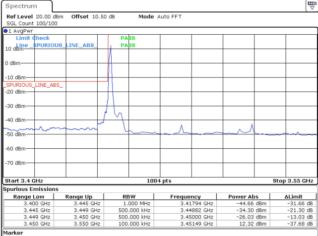
70MHz_30kHz_3485MHz_DFT-s-OFDM QPSK_RB1@0 -26.03 dBm
