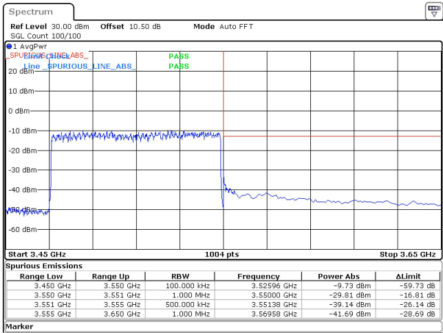
80MHz_30kHz_3510MHz_DFT-s-OFDM QPSK_RB216@0 -29.81 dBm
