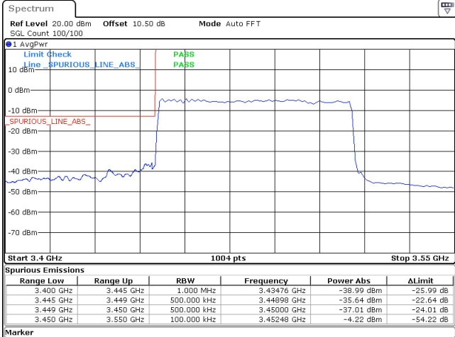
70MHz_30kHz_3485MHz_DFT-s-OFDM QPSK_RB180@0 -35.64 dBm
