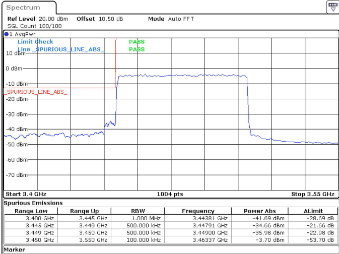
60MHz_30kHz_3480MHz_DFT-s-OFDM QPSK_RB162@0 -34.66 dBm
