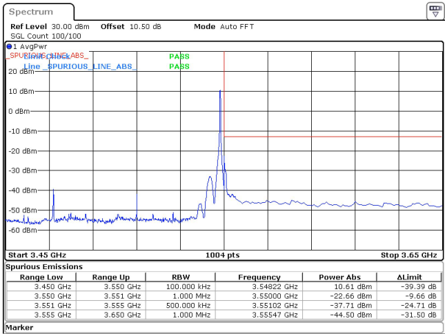
80MHz_30kHz_3510MHz_DFT-s-OFDM QPSK_RB1@216 -22.66 dBm
