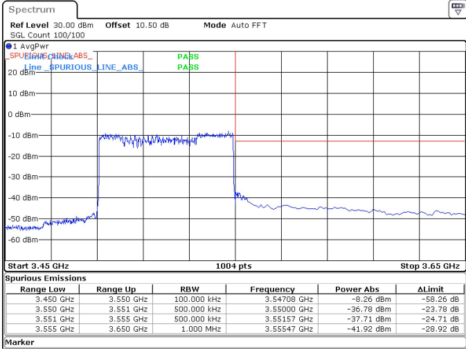
60MHz_30kHz_3520MHz_DFT-s-OFDM QPSK_RB162@0 -36.78 dBm
