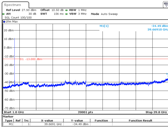
40MHz_30kHz_3720MHz_DFT-s-OFDM QPSK_RB1@0&amp;-34.49 dBm
