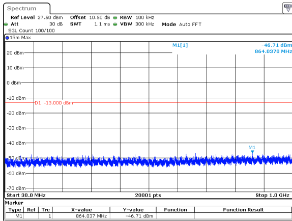
60MHz_30kHz_3730MHz_DFT-s-OFDM QPSK_RB1@0&amp;-46.71 dBm
