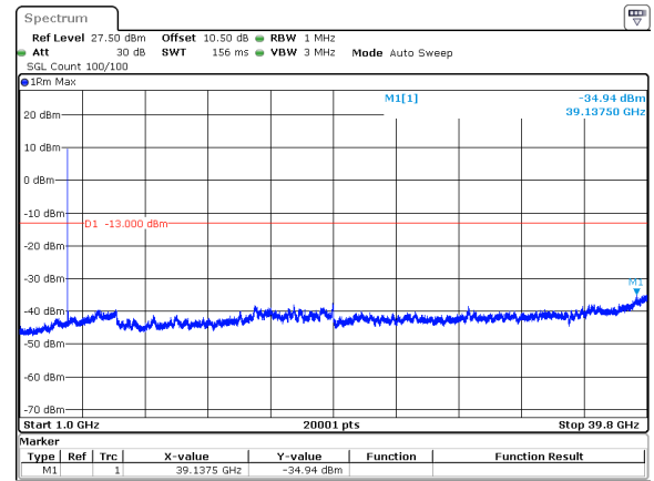
20MHz_30kHz_3970MHz_DFT-s-OFDM QPSK_RB1@0&amp;-34.94 dBm
