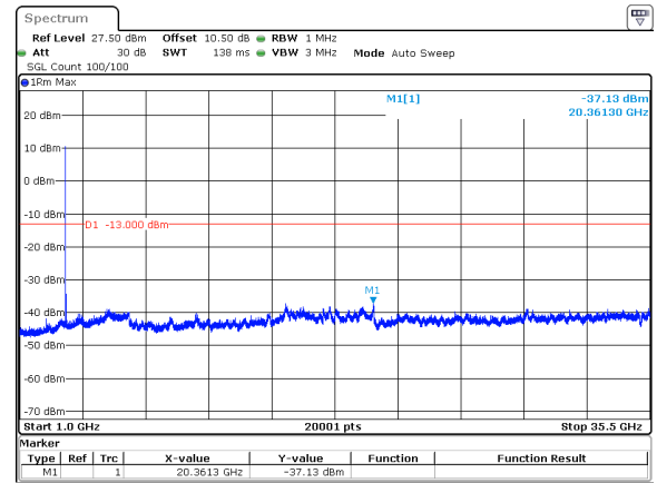
10MHz_30kHz_3500MHz_DFT-s-OFDM QPSK_RB1@0&amp;-37.13 dBm
