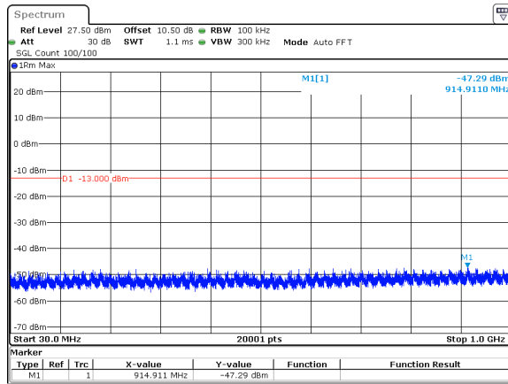
40MHz_30kHz_3960MHz_DFT-s-OFDM QPSK_RB1@0&amp;-47.29 dBm
