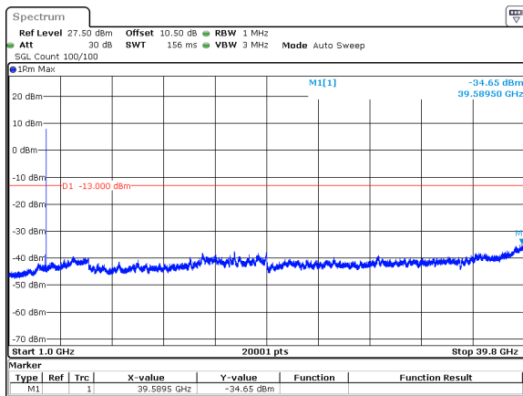
100MHz_30kHz_3750MHz_DFT-s-OFDM QPSK_RB1@272&amp;-34.65 dBm
