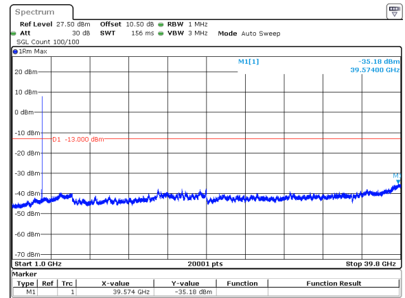
60MHz_30kHz_3950MHz_DFT-s-OFDM QPSK_RB1@161&amp;-35.18 dBm
