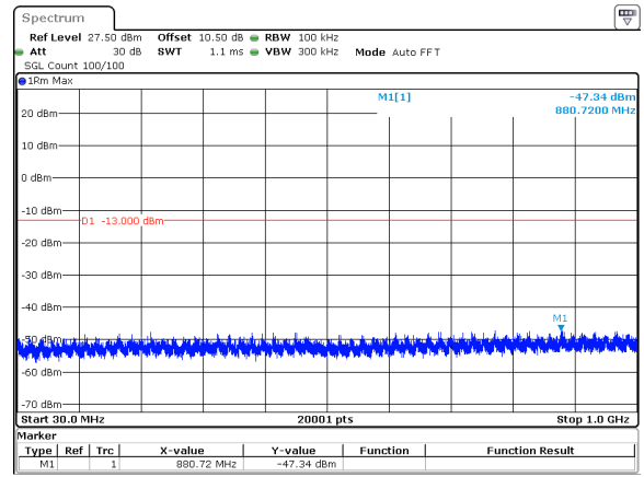
80MHz_30kHz_3940MHz_DFT-s-OFDM QPSK_RB1@0&amp;-47.34 dBm
