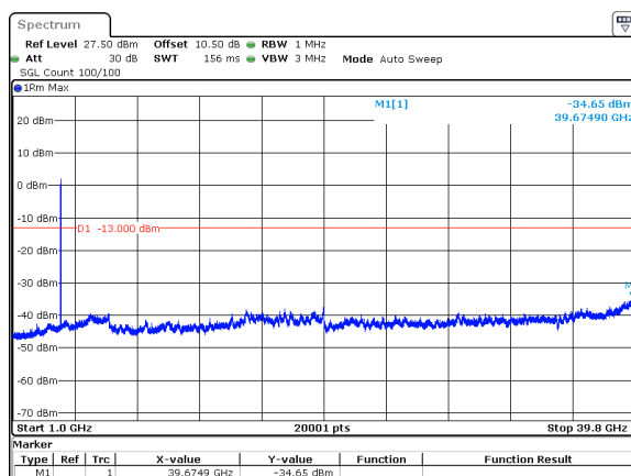
20MHz_30kHz_3970MHz_DFT-s-OFDM QPSK_RB50@0&amp;-34.65 dBm
