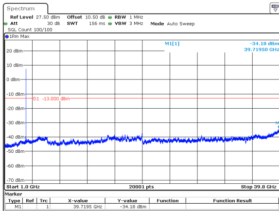
80MHz_30kHz_3940MHz_DFT-s-OFDM QPSK_RB1@216&amp;-34.18 dBm
