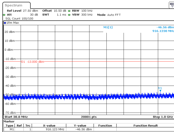
40MHz_15kHz_3720MHz_DFT-s-OFDM QPSK_RB1@215&amp;-46.56 dBm
