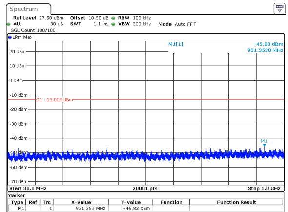
100MHz_30kHz_3750MHz_DFT-s-OFDM QPSK_RB1@272&amp;-45.83 dBm
