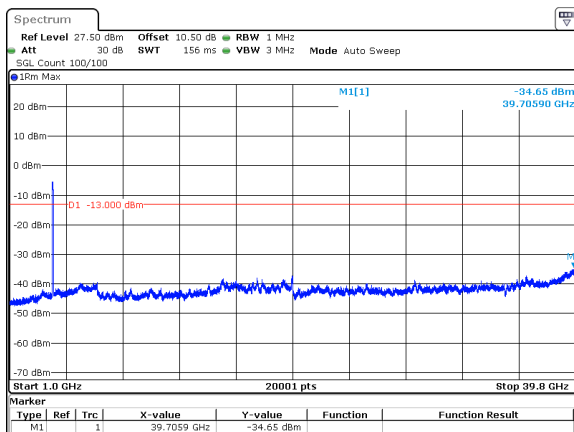
80MHz_30kHz_3940MHz_DFT-s-OFDM QPSK_RB216@0&amp;-34.65 dBm
