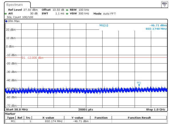
40MHz_15kHz_3960MHz_DFT-s-OFDM QPSK_RB1@0&amp;-46.71 dBm
