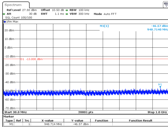
20MHz_30kHz_3970MHz_DFT-s-OFDM QPSK_RB1@0&amp;-46.57 dBm
