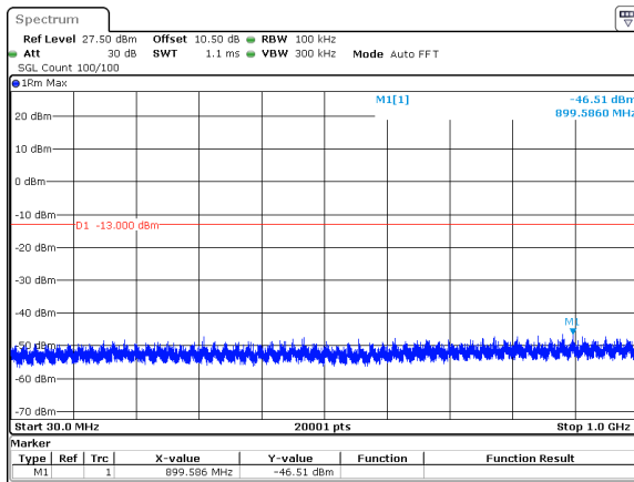
20MHz_30kHz_3840MHz_DFT-s-OFDM QPSK_RB1@50&amp;-46.51 dBm
