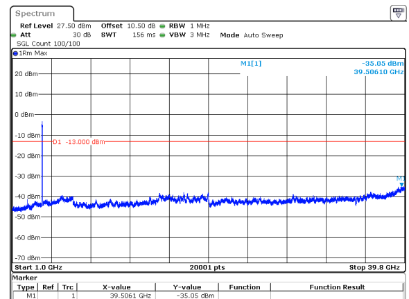
60MHz_30kHz_3950MHz_DFT-s-OFDM QPSK_RB162@0&amp;-35.05 dBm
