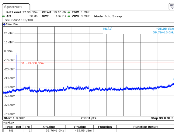
50MHz_15kHz_3955MHz_DFT-s-OFDM QPSK_RB270@0&amp;-35.08 dBm
