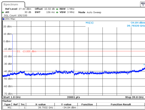
100MHz_30kHz_3750MHz_DFT-s-OFDM QPSK_RB1@0&amp;-34.84 dBm
