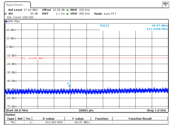
90MHz_30kHz_3745MHz_DFT-s-OFDM QPSK_RB1@0&amp;-46.97 dBm
