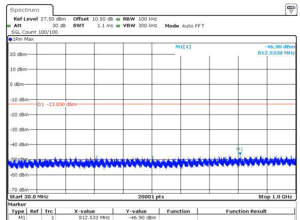
90MHz_30kHz_3935MHz_DFT-s-OFDM QPSK_RB243@0&amp;-46.90 dBm
