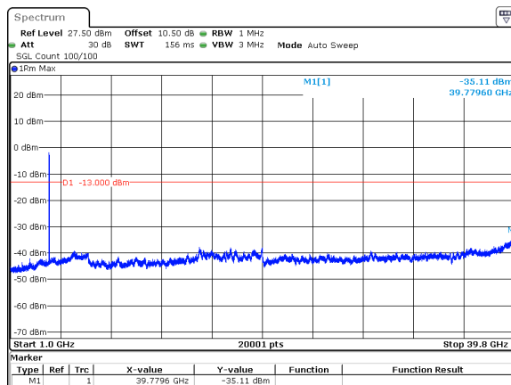
40MHz_30kHz_3960MHz_DFT-s-OFDM QPSK_RB100@0&amp;-35.11 dBm
