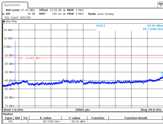
90MHz_30kHz_3935MHz_DFT-s-OFDM QPSK_RB1@244&amp;-35.01 dBm
