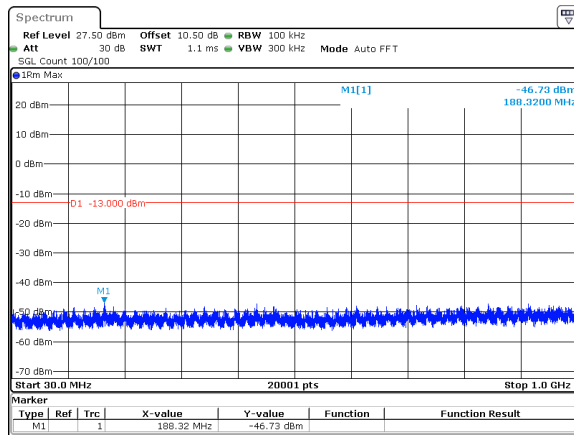
10MHz_30kHz_3500MHz_DFT-s-OFDM QPSK_RB1@23&amp;-46.73 dBm
