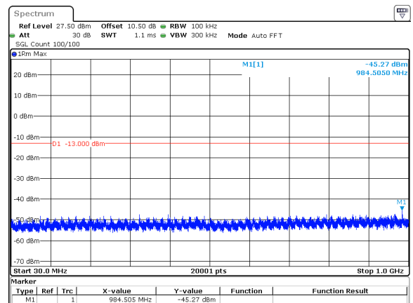
80MHz_30kHz_3940MHz_DFT-s-OFDM QPSK_RB216@0&amp;-45.27 dBm
