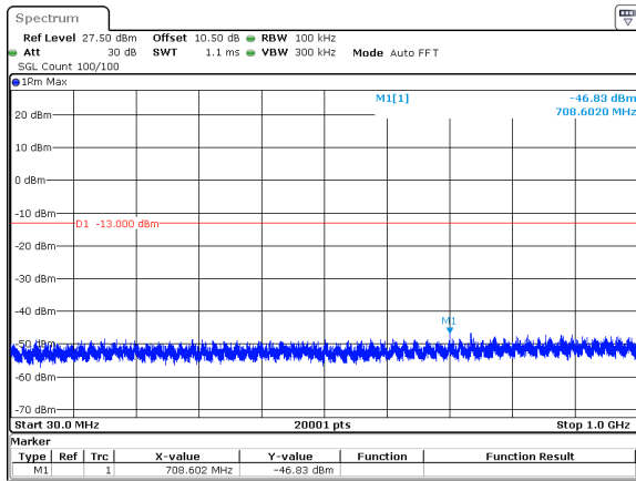
50MHz_30kHz_3955MHz_DFT-s-OFDM QPSK_RB1@0&amp;-46.83 dBm
