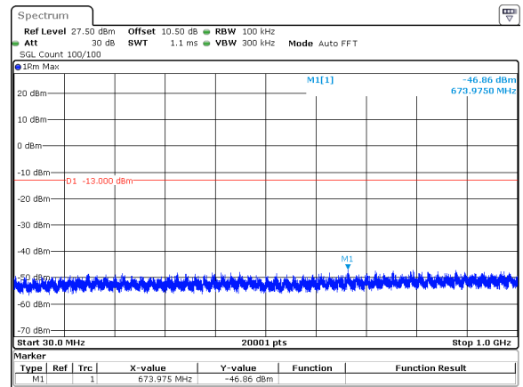
80MHz_30kHz_3940MHz_DFT-s-OFDM QPSK_RB1@216&amp;-46.86 dBm
