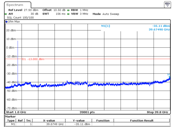
40MHz_30kHz_3960MHz_DFT-s-OFDM QPSK_RB1@0&amp;-35.11 dBm
