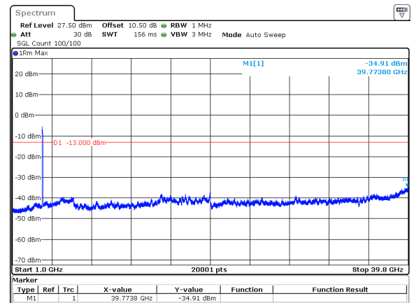
100MHz_30kHz_3930MHz_DFT-s-OFDM QPSK_RB270@0&amp;-34.91 dBm
