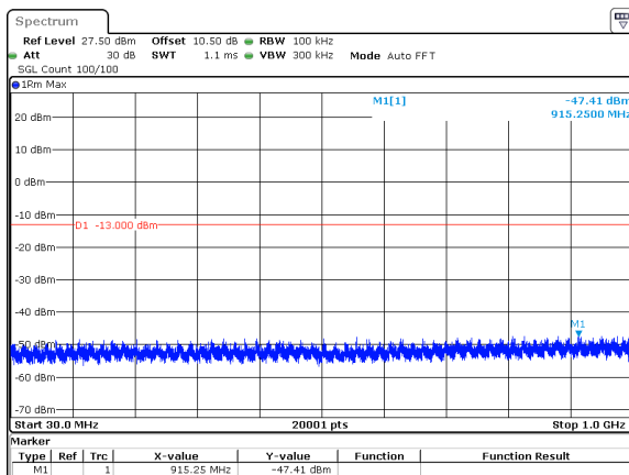
60MHz_30kHz_3950MHz_DFT-s-OFDM QPSK_RB162@0&amp;-47.41 dBm
