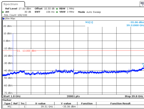
20MHz_30kHz_3840MHz_DFT-s-OFDM QPSK_RB1@0&amp;-35.06 dBm
