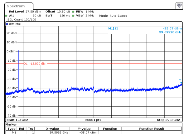
20MHz_30kHz_3840MHz_DFT-s-OFDM QPSK_RB50@0&amp;-35.07 dBm
