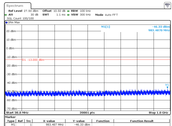
90MHz_30kHz_3745MHz_DFT-s-OFDM QPSK_RB243@0&amp;-46.33 dBm
