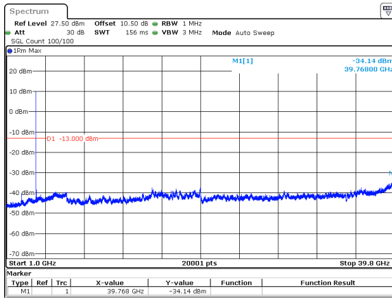
60MHz_30kHz_3950MHz_DFT-s-OFDM QPSK_RB1@0&amp;-34.14 dBm
