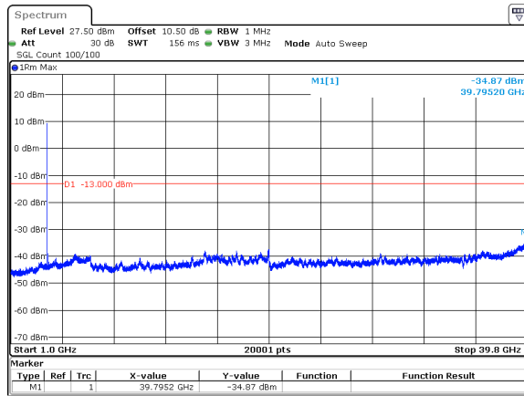
90MHz_30kHz_3745MHz_DFT-s-OFDM QPSK_RB1@0&amp;-34.87 dBm
