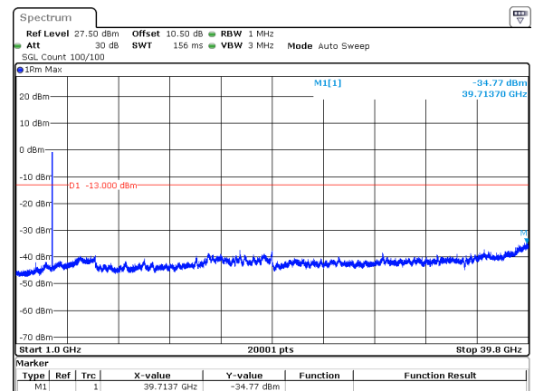
40MHz_30kHz_3720MHz_DFT-s-OFDM QPSK_RB100@0&amp;-34.77 dBm
