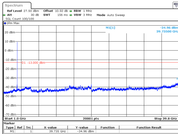
40MHz_15kHz_3960MHz_DFT-s-OFDM QPSK_RB1@215&amp;-34.96 dBm
