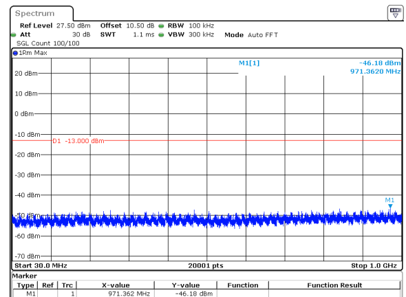
40MHz_30kHz_3960MHz_DFT-s-OFDM QPSK_RB100@0&amp;-46.18 dBm
