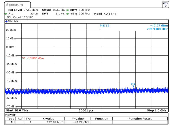
40MHz_30kHz_3720MHz_DFT-s-OFDM QPSK_RB1@0&amp;-47.27 dBm
