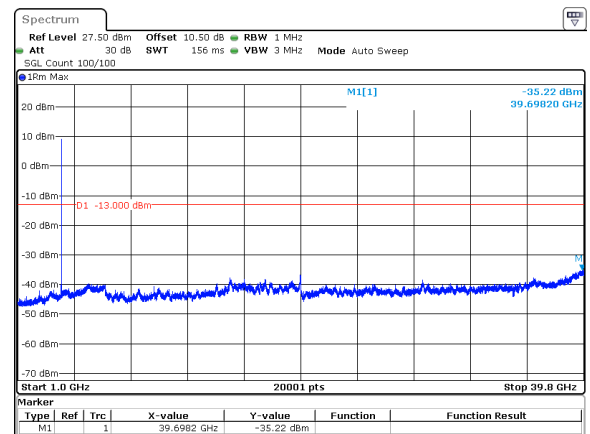
20MHz_30kHz_3970MHz_DFT-s-OFDM QPSK_RB1@50&amp;-35.22 dBm
