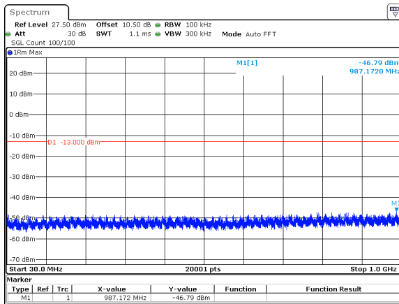
60MHz_30kHz_3950MHz_DFT-s-OFDM QPSK_RB1@161&amp;-46.79 dBm
