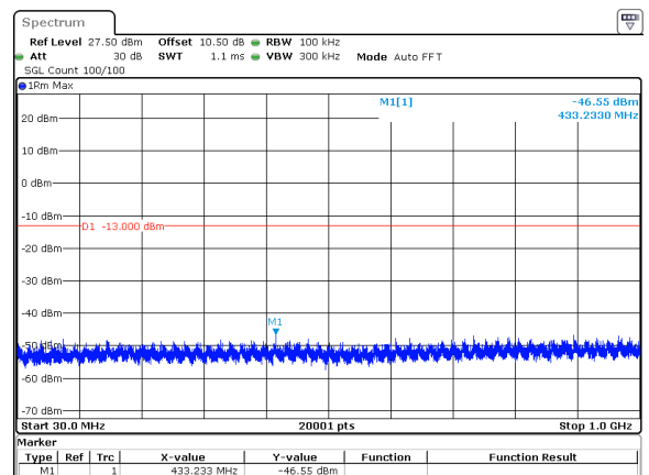
100MHz_30kHz_3750MHz_DFT-s-OFDM QPSK_RB270@0&amp;-46.55 dBm
