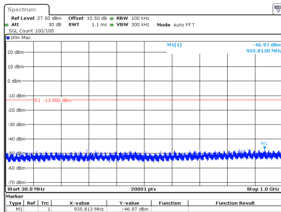
20MHz_30kHz_3970MHz_DFT-s-OFDM QPSK_RB1@50&amp;-46.97 dBm
