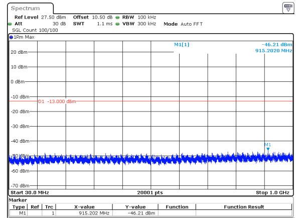
20MHz_30kHz_3840MHz_DFT-s-OFDM QPSK_RB1@0&amp;-46.21 dBm
