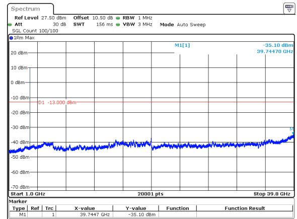
20MHz_30kHz_3840MHz_DFT-s-OFDM QPSK_RB1@50&amp;-35.10 dBm
