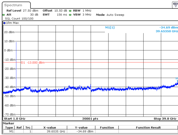
80MHz_30kHz_3940MHz_DFT-s-OFDM QPSK_RB1@0&amp;-34.69 dBm
