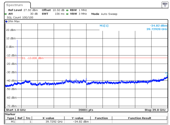
100MHz_30kHz_3930MHz_DFT-s-OFDM QPSK_RB1@0&amp;-34.82 dBm
