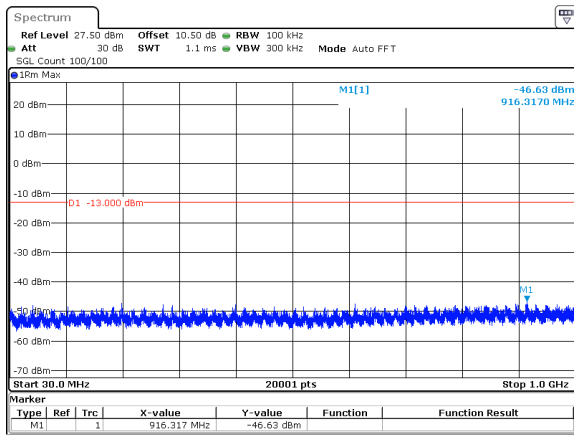
100MHz_30kHz_3930MHz_DFT-s-OFDM QPSK_RB1@0&amp;-46.63 dBm
