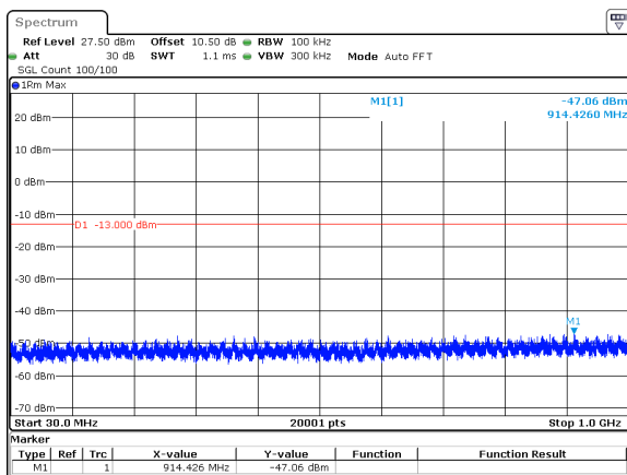
100MHz_30kHz_3840MHz_DFT-s-OFDM QPSK_RB270@0&amp;-47.06 dBm
