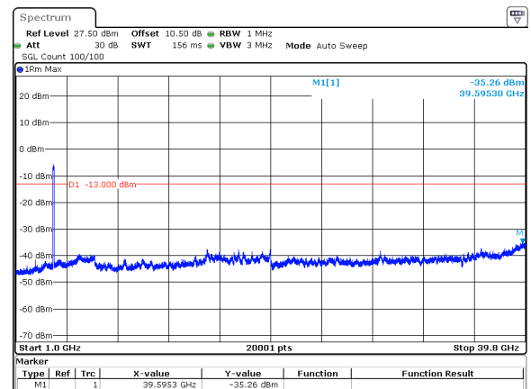
90MHz_30kHz_3840MHz_DFT-s-OFDM QPSK_RB243@0&amp;-35.26 dBm
