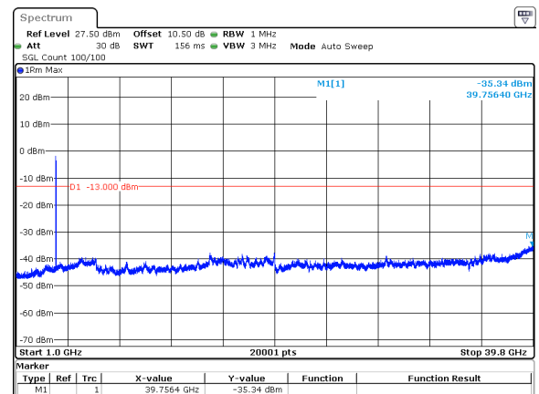
40MHz_15kHz_3960MHz_DFT-s-OFDM QPSK_RB216@0&amp;-35.34 dBm
