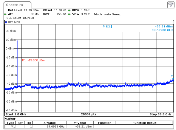
90MHz_30kHz_3935MHz_DFT-s-OFDM QPSK_RB1@0&amp;-35.21 dBm
