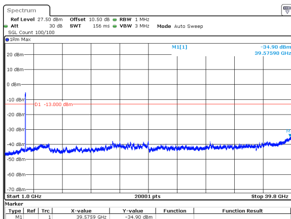
100MHz_30kHz_3750MHz_DFT-s-OFDM QPSK_RB270@0&amp;-34.90 dBm
