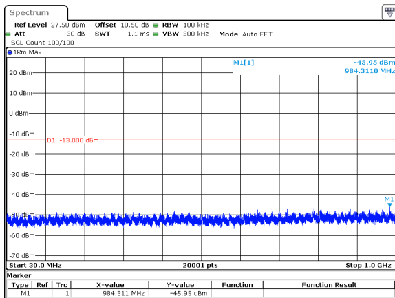
100MHz_30kHz_3930MHz_DFT-s-OFDM QPSK_RB270@0&amp;-45.95 dBm
