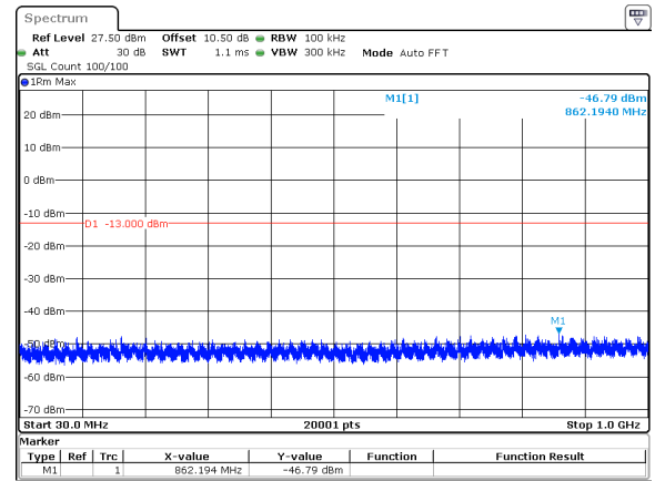
60MHz_30kHz_3950MHz_DFT-s-OFDM QPSK_RB1@0&amp;-46.79 dBm
