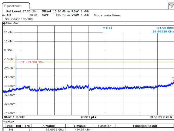
90MHz_30kHz_3935MHz_DFT-s-OFDM QPSK_RB243@0&amp;-34.98 dBm
