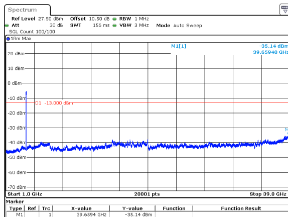
90MHz_30kHz_3745MHz_DFT-s-OFDM QPSK_RB243@0&amp;-35.14 dBm
