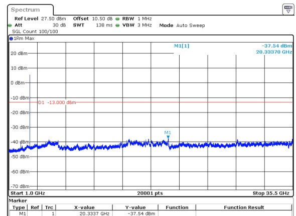
10MHz_30kHz_3545MHz_DFT-s-OFDM QPSK_RB24@0&amp;-37.54 dBm
