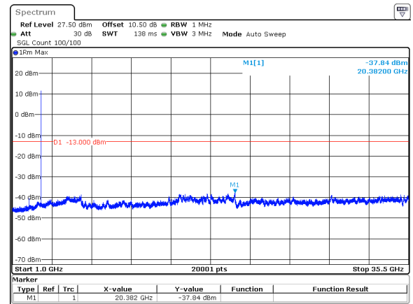
10MHz_30kHz_3500MHz_DFT-s-OFDM QPSK_RB1@23&amp;-37.84 dBm
