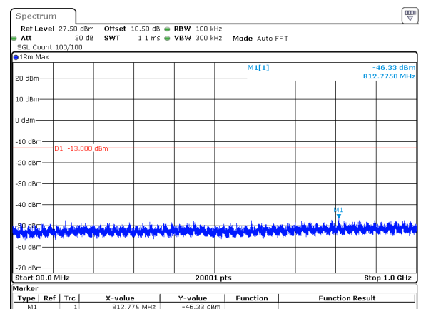
20MHz_30kHz_3970MHz_DFT-s-OFDM QPSK_RB50@0&amp;-46.33 dBm
