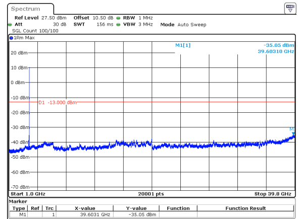
40MHz_15kHz_3720MHz_DFT-s-OFDM QPSK_RB1@215&amp;-35.05 dBm
