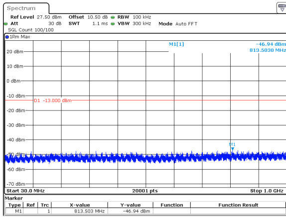
90MHz_30kHz_3935MHz_DFT-s-OFDM QPSK_RB1@0&amp;-46.94 dBm
