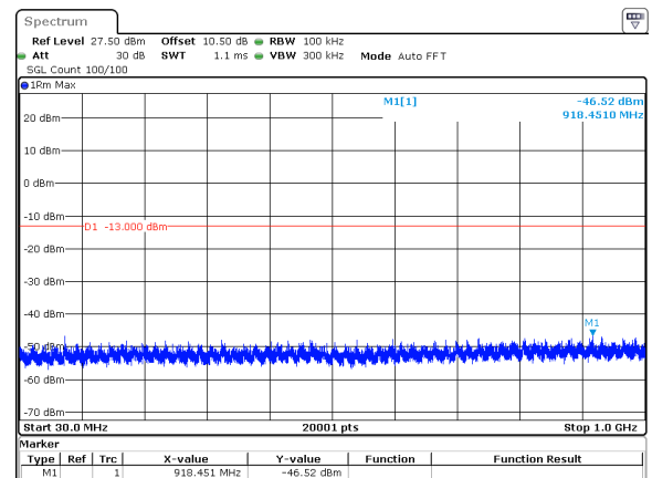
10MHz_30kHz_3500MHz_DFT-s-OFDM QPSK_RB24@0&amp;-46.52 dBm
