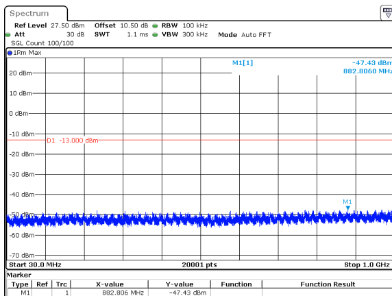
20MHz_30kHz_3840MHz_DFT-s-OFDM QPSK_RB50@0&amp;-47.43 dBm
