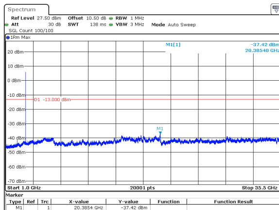
10MHz_30kHz_3500MHz_DFT-s-OFDM QPSK_RB24@0&amp;-37.42 dBm
