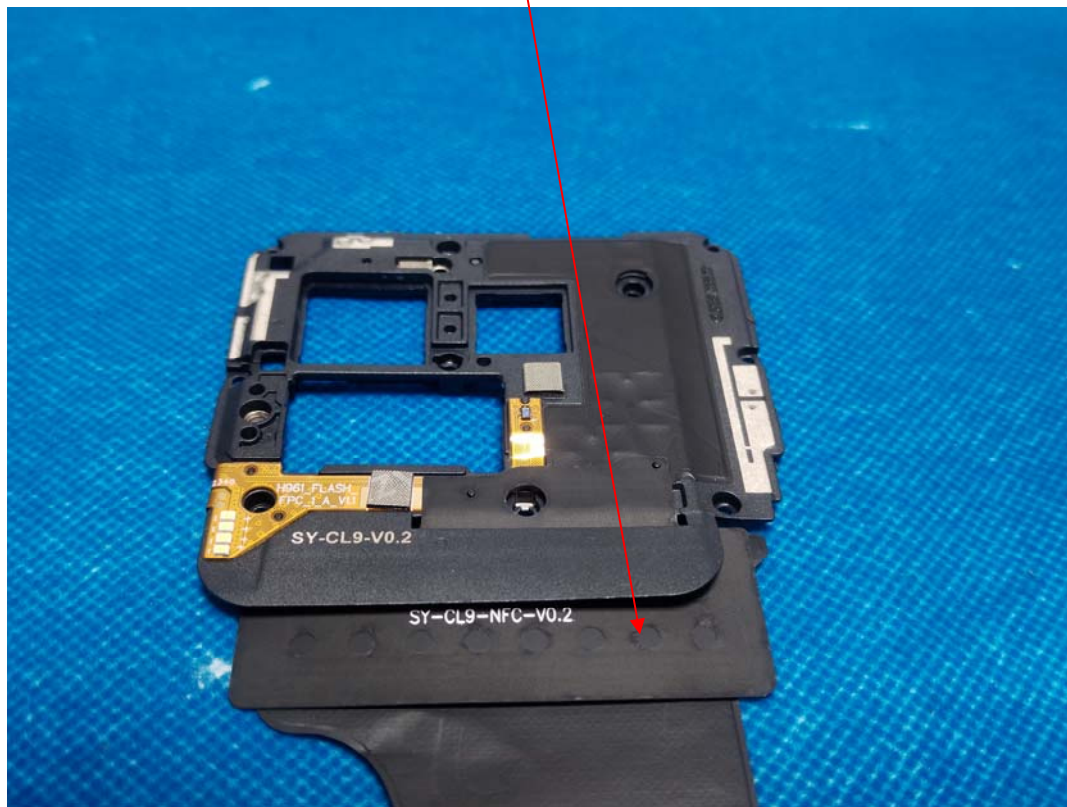
NFC Antenna
