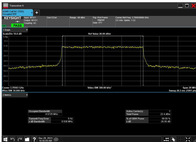
10MHz_30kHz_3705MHz_DFT-s-OFDM QPSK_RB24@0 8.573 MHz
