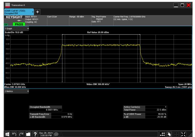
10MHz_30kHz_3975MHz_DFT-s-OFDM PI/2 BPSK_RB24@0 8.568 MHz
