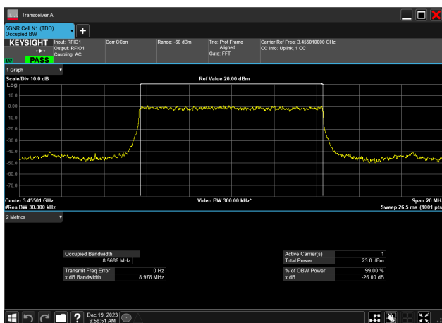
10MHz_30kHz_3455MHz_DFT-s-OFDM PI/2 BPSK_RB24@0 8.569 MHz
