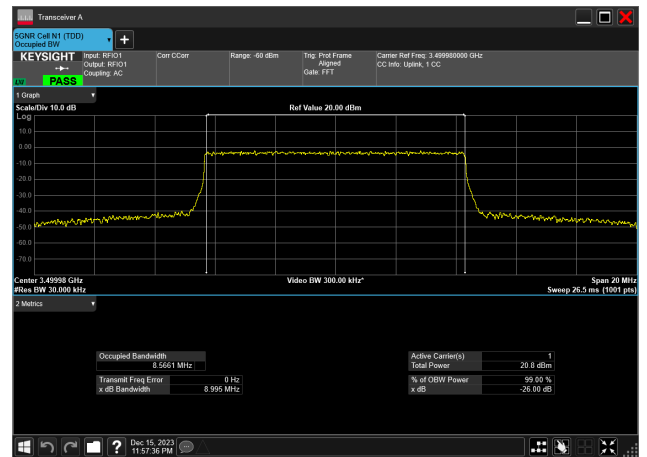
10MHz_30kHz_3500MHz_CP-OFDM QPSK_RB24@0 8.566 MHz
