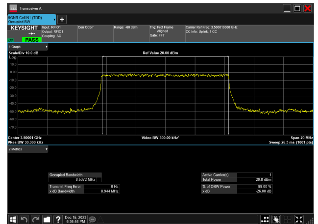
10MHz_30kHz_3500MHz_DFT-s-OFDM PI/2 BPSK_RB24@0 8.537 MHz
