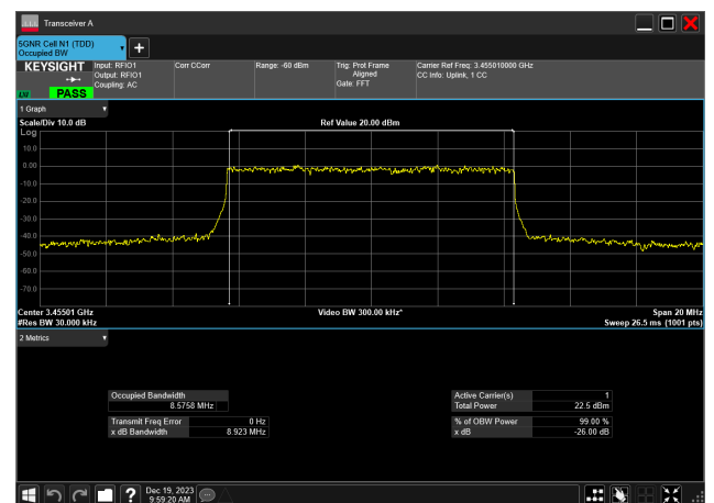
10MHz_30kHz_3455MHz_DFT-s-OFDM QPSK_RB24@0 8.576 MHz
