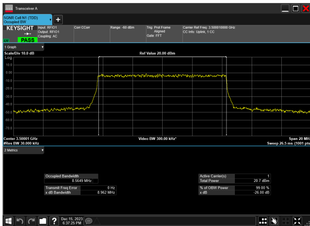
10MHz_30kHz_3500MHz_DFT-s-OFDM QPSK_RB24@0 8.565 MHz
