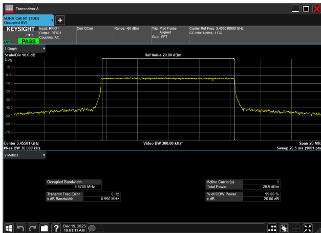
10MHz_30kHz_3455MHz_CP-OFDM QPSK_RB24@0 8.570 MHz
