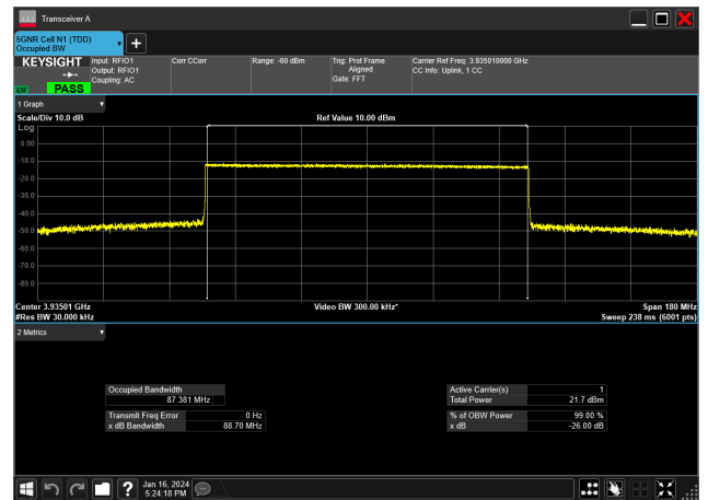
90MHz_30kHz_3935MHz_CP-OFDM QPSK_RB245@0 87.381 MHz
