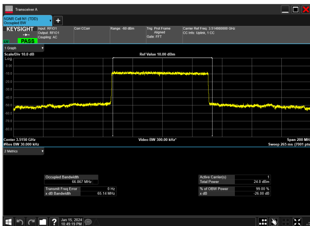
70MHz_30kHz_3515MHz_DFT-s-OFDM QPSK_RB180@0 66.867 MHz
