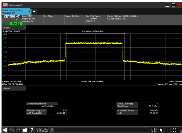
70MHz_30kHz_3485MHz_DFT-s-OFDM QPSK_RB180@0 66.748 MHz
