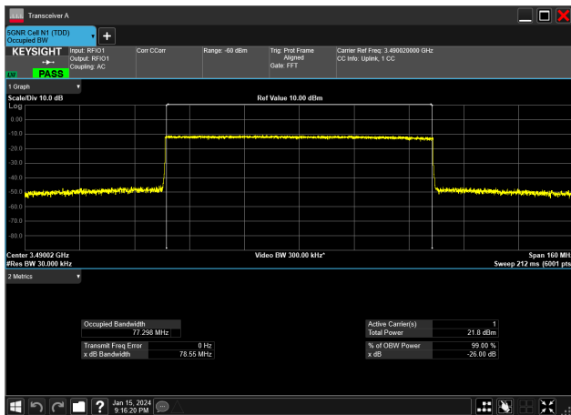
80MHz_30kHz_3490MHz_CP-OFDM QPSK_RB217@0 77.298 MHz
