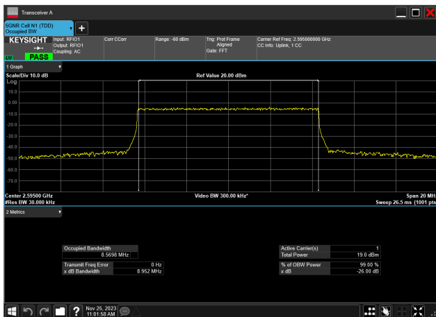
10MHz_30kHz_2595MHz_CP-OFDM QPSK_RB24@0 8.570 MHz
