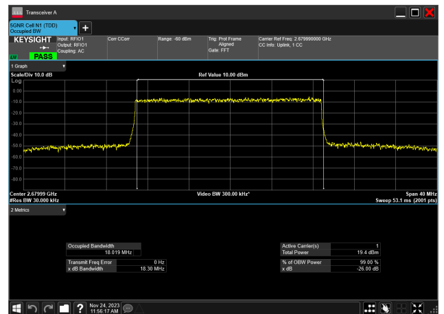
20MHz_30kHz_2679.99MHz_DFT-s-OFDM 64 QAM_RB50@0 18.019 MHz
