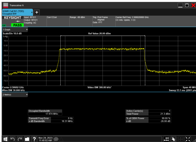
20MHz_30kHz_2506.02MHz_DFT-s-OFDM PI/2 BPSK_RB50@0 17.974 MHz
