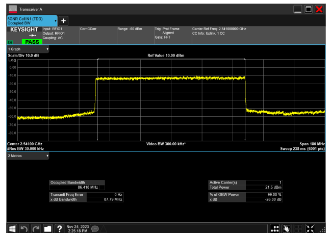
90MHz_30kHz_2541MHz_DFT-s-OFDM PI/2 BPSK_RB243@0 86.418 MHz
