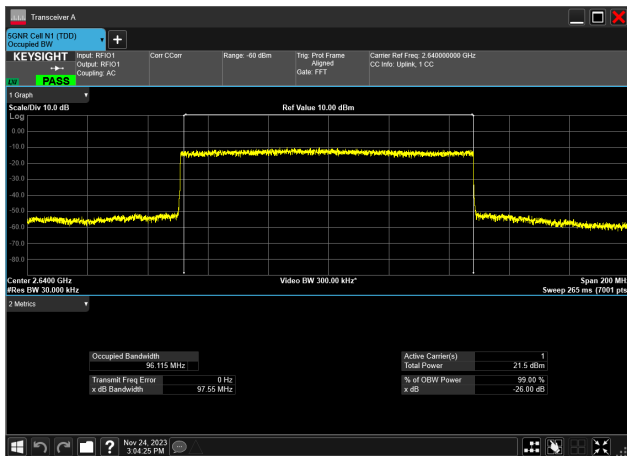
100MHz_30kHz_2640MHz_DFT-s-OFDM PI/2 BPSK_RB270@0 96.115 MHz
