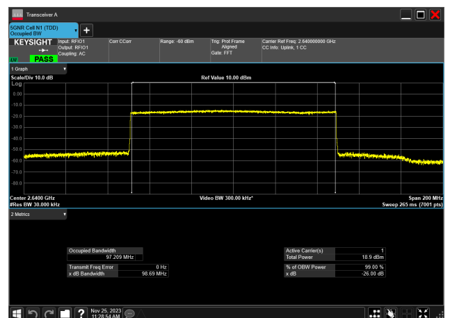
100MHz_30kHz_2640MHz_CP-OFDM QPSK_RB273@0 97.209 MHz
