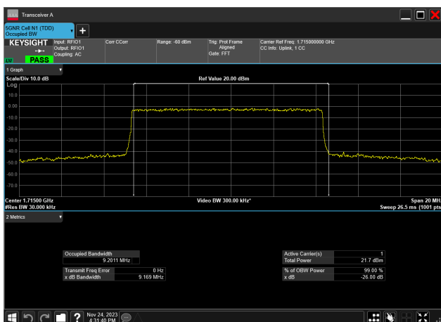
10MHz_15kHz_1715MHz_DFT-s-OFDM QPSK_RB50@0 9.201 MHz
