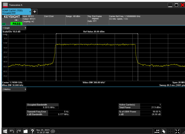
10MHz_15kHz_1745MHz_DFT-s-OFDM PI/2 BPSK_RB50@0 9.201 MHz
