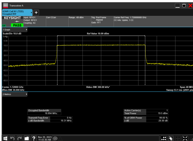
20MHz_15kHz_1720MHz_CP-OFDM QPSK_RB106@0 18.894 MHz
