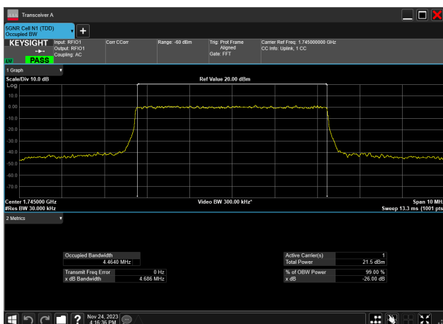
5MHz_15kHz_1745MHz_DFT-s-OFDM QPSK_RB25@0 4.464 MHz
