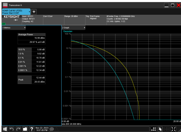
20MHz_15kHz_2535MHz_CP-OFDM QPSK_RB106@0 10.70 dB
