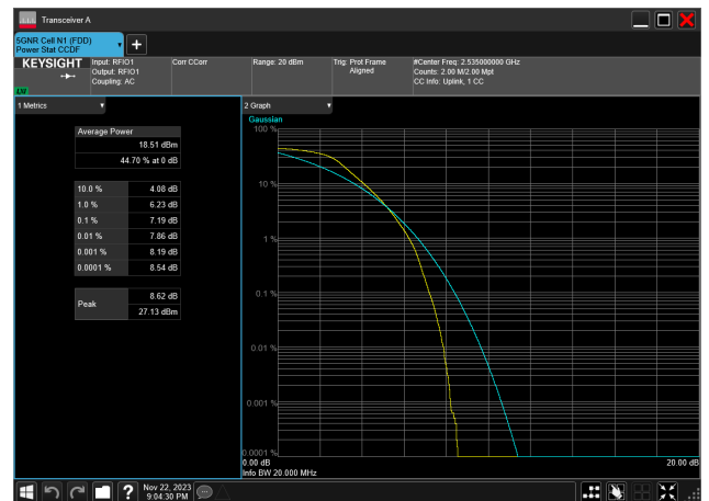
20MHz_15kHz_2535MHz_DFT-s-OFDM PI/2 BPSK_RB100@0 7.19 dB
