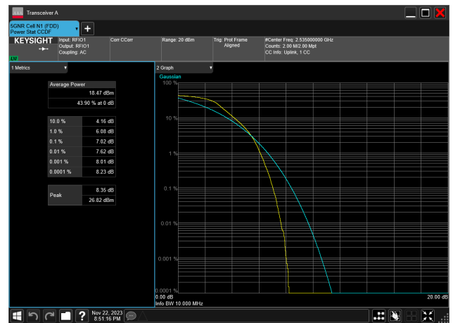
10MHz_15kHz_2535MHz_DFT-s-OFDM PI/2 BPSK_RB50@0 7.02 dB
