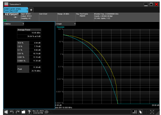
10MHz_15kHz_2535MHz_DFT-s-OFDM 256 QAM_RB50@0 9.56 dB
