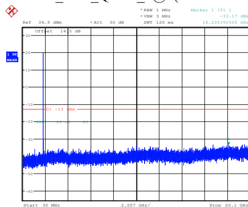
20MHz Low QPSK 1@0(30MHz~20.1GHz)
