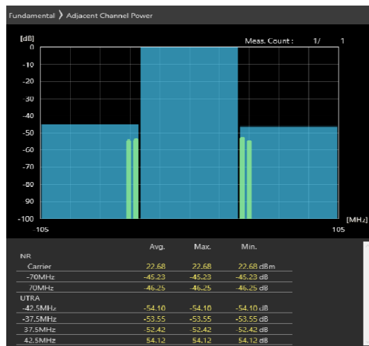
70MHz_30kHz_3665MHz-OFDM QPSK_RB90@45 -45.23,-46.25dB
