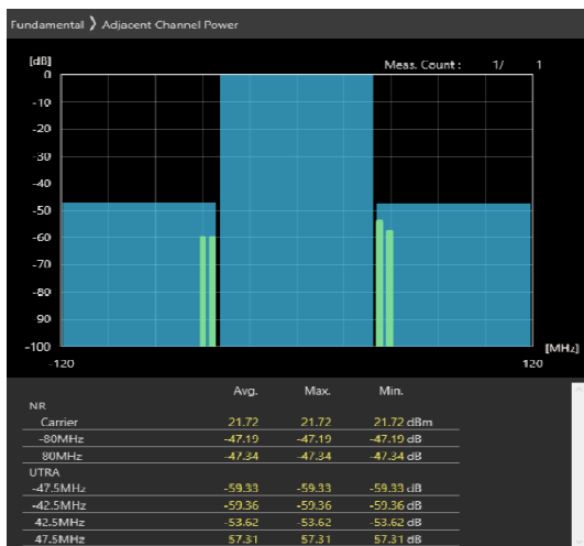
80MHz_30kHz_3660MHz-OFDM QPSK_RB1@216 -47.19,-47.34dB
