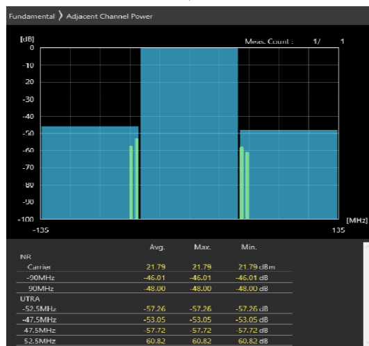
90MHz_30kHz_3655MHz-OFDM QPSK_RB120@60 -45.66,-45.79dB
