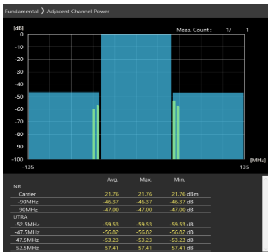
90MHz_30kHz_3655MHz-OFDM QPSK_RB1@244 -46.37,-47dB
