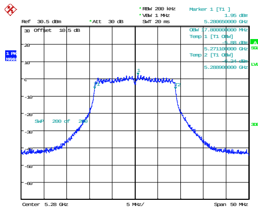
802.11n20_5280MHz_Chain 1 17.800MHz
