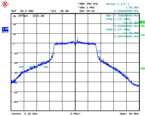
802.11a_5320MHz_Chain 0 17.750MHz
