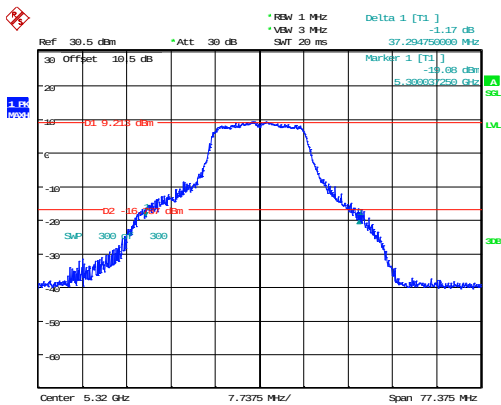
802.11a_5320MHz_Chain 1 37.295MHz
