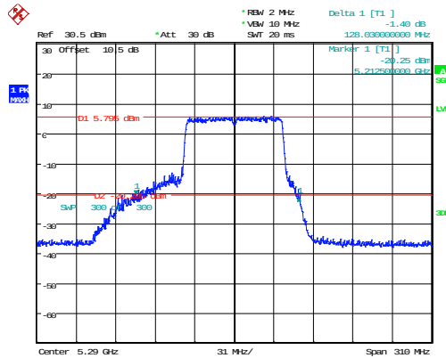
802.11ac80_5290MHz_Chain 0 128.030MHz
