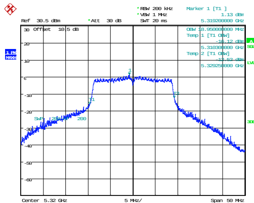
802.11n20_5320MHz_Chain 0 18.950MHz
