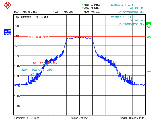
802.11n20_5200MHz_Chain 0 46.058MHz
