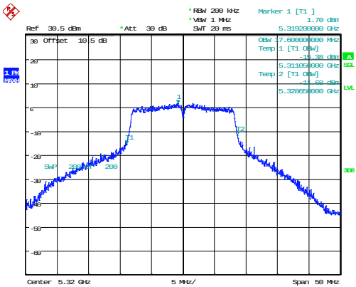
802.11a_5320MHz_Chain 1 17.600MHz
