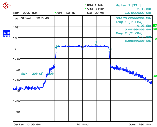
802.11ac80_5530MHz_Chain 0 76.600MHz
