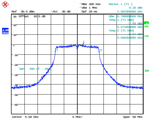
802.11a_5580MHz_Chain 1 16.700MHz
