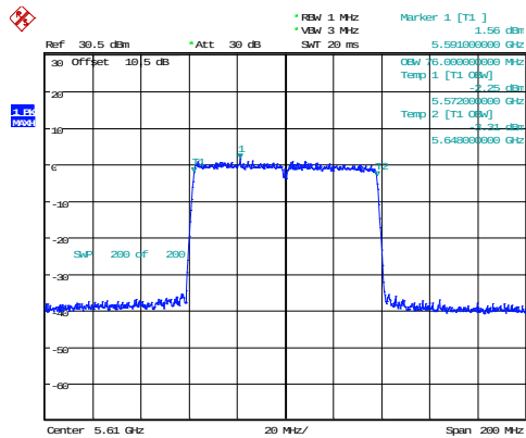
802.11ac80_5610MHz_Chain 1 76MHz
