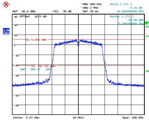
802.11n40_5270MHz_Chain 1 40.500MHz
