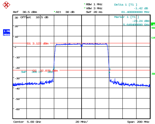
802.11ac80_5690MHz_Chain 0 81.400MHz
