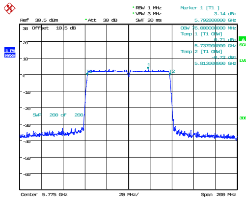
802.11ac80_5775MHz_Chain 0 76MHz
