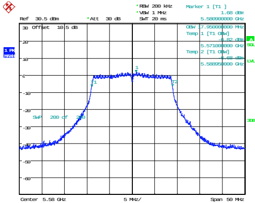
802.11n20_5580MHz_Chain 0 17.950MHz
