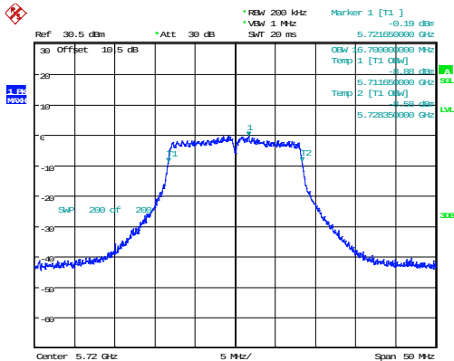
802.11a_5720MHz_Chain 1 16.700MHz
