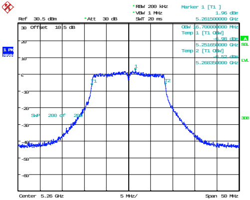
802.11a_5260MHz_Chain 1 16.700MHz
