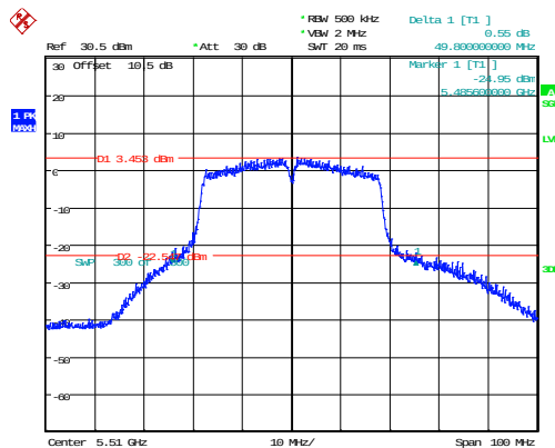
802.11n40_5510MHz_Chain 1 49.800MHz
