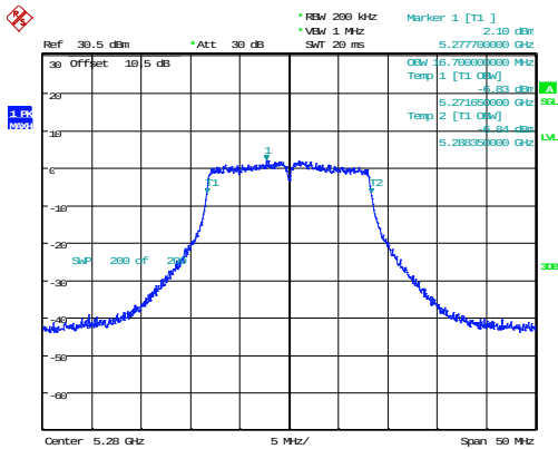
802.11a_5280MHz_Chain 1 16.700MHz
