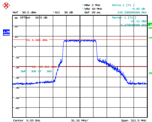
802.11ac80_5530MHz_Chain 0 128.338MHz
