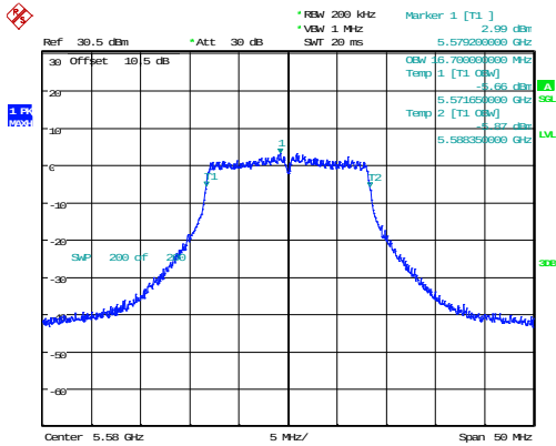
802.11a_5580MHz_Chain 0 16.700MHz
