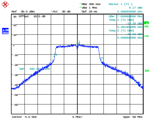
802.11a_5500MHz_Chain 1 17.650MHz
