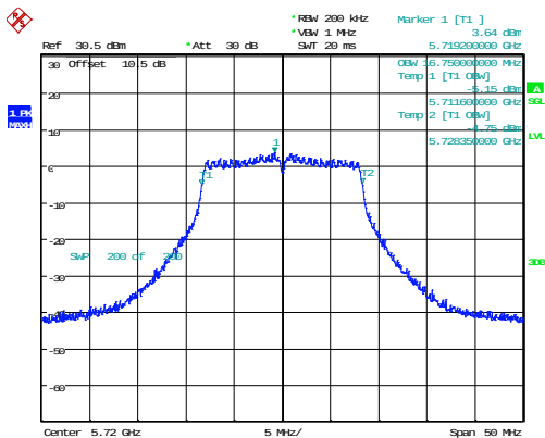
802.11a_5720MHz_Chain 0 16.750MHz
