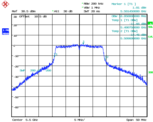
802.11n20_5500MHz_Chain 0 18.850MHz
