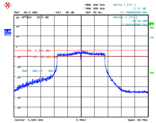
802.11n20_5825MHz_Chain 1 17.700MHz
