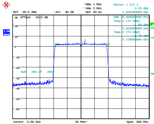
802.11ac80_5690MHz_Chain 0 76MHz
