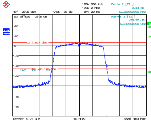
802.11n40_5270MHz_Chain 0 41.200MHz
