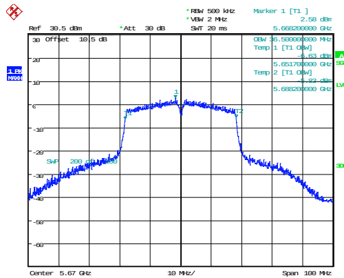
802.11n40_5670MHz_Chain 1 36.500MHz
