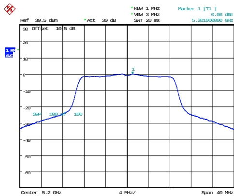
802.11n20_5200MHz_Chain 1
