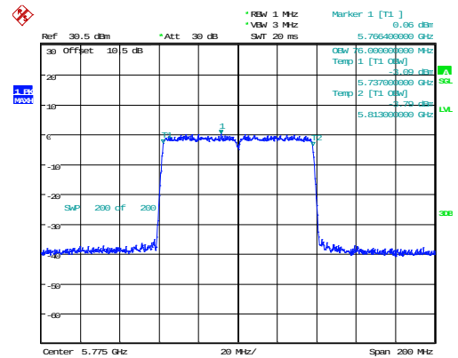
802.11ac80_5775MHz_Chain 1 76MHz
