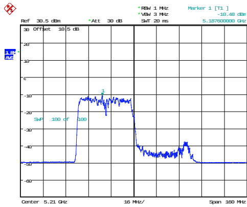
802.11ax80_5210MHz_RU_484/65_Chain 0
