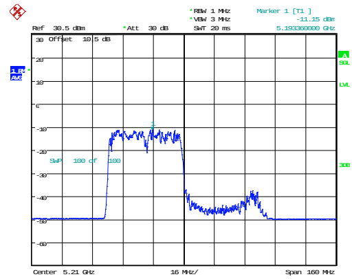
802.11ax80_5210MHz_RU_484/65_Chain 1
