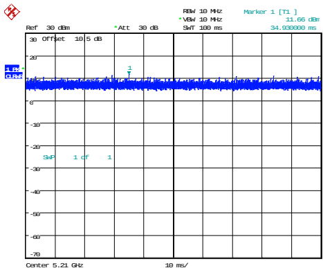
802.11ac80_5210MHz_Chain 0 100ms,100ms
