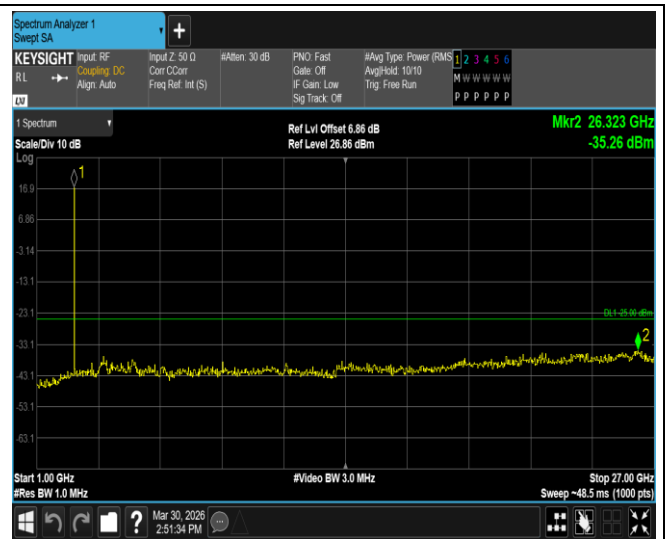
Band41-5MHz-16QAM-41565-1RB#0-Range2:1000~27000MHz
