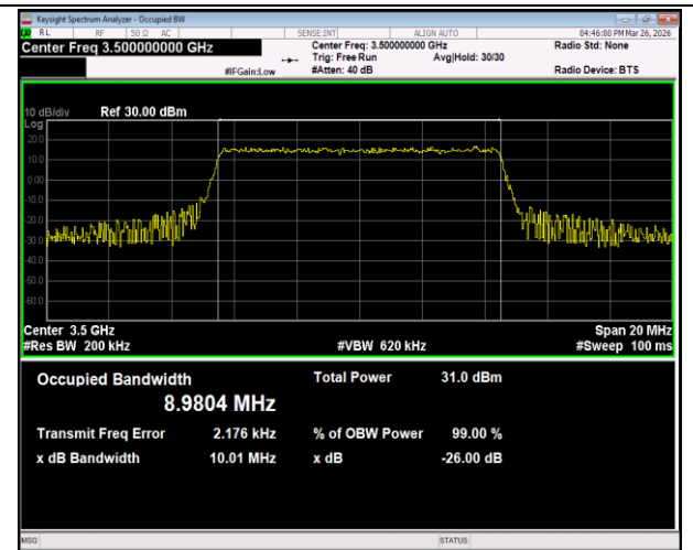
Band42(3450-3550)-10MHz-QPSK-43040-50RB#0-PASS
