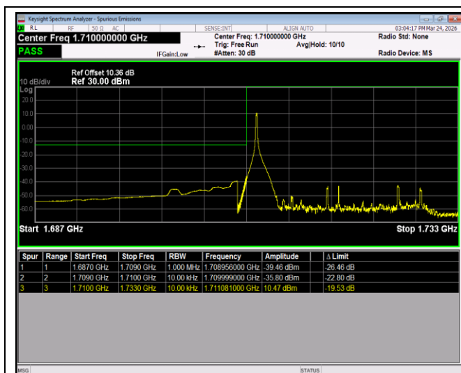
Band4-20MHz-QPSK-20050-100RB#0
