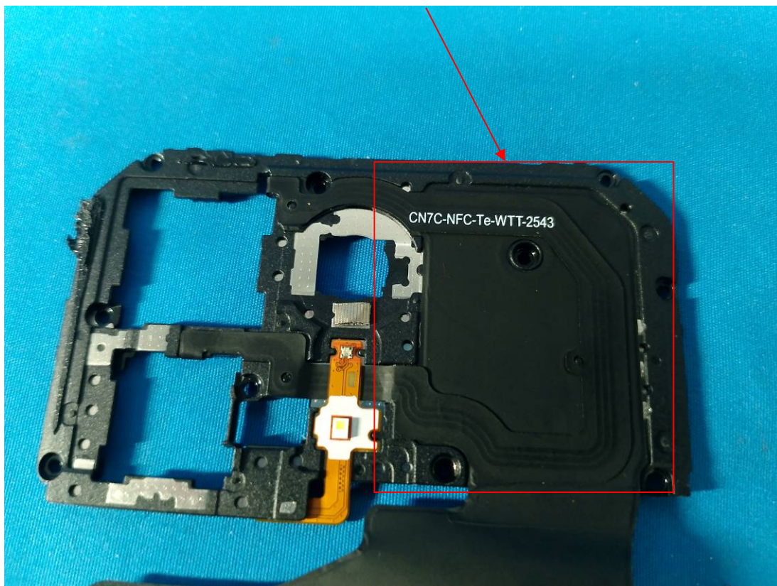
NFC Antenna
