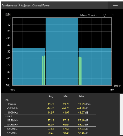
100MHz_30kHz_3650MHz-OFDM QPSK_RB135@67 -44.7,-44.97dB
