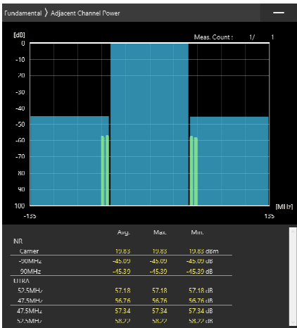
90MHz_30kHz_3655MHz-OFDM QPSK_RB120@60 -45.09,-45.39dB
