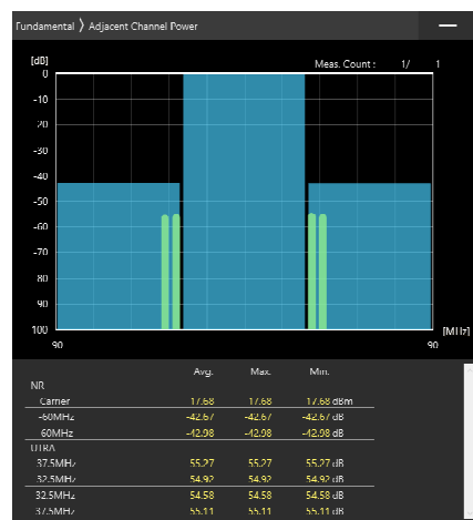
60MHz_30kHz_3670MHz-OFDM QPSK_RB162@0 -42.67,-42.98dB
