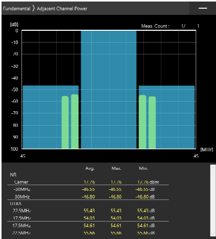
30MHz_30kHz_3685MHz-OFDM QPSK_RB75@0 -46.55,-46.8dB
