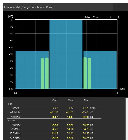
40MHz_30kHz_3680MHz-OFDM QPSK_RB100@0 -45.83,-45.67dB
