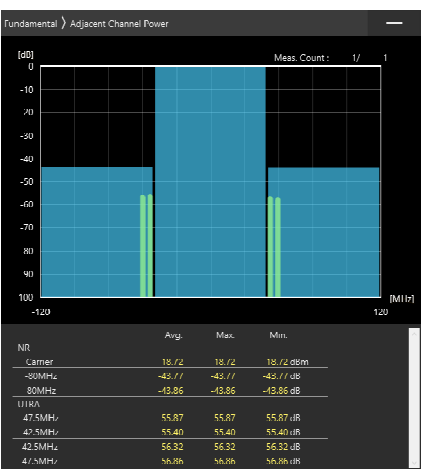
80MHz_30kHz_3660MHz-OFDM QPSK_RB216@0 -43.77,-43.86dB
