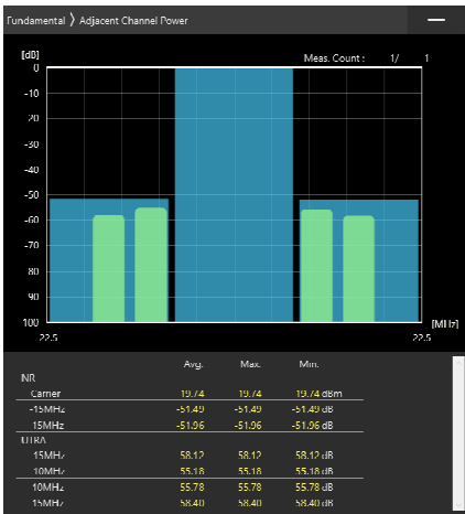
15MHz_30kHz_3692.5MHz-OFDM QPSK_RB18@9 -51.49,-51.96dB
