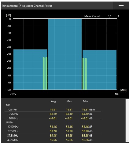
70MHz_30kHz_3665MHz-OFDM QPSK_RB180@0 -43.19,-44.01dB
