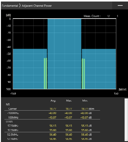
100MHz_30kHz_3650MHz-OFDM QPSK_RB270@0 -43,-43.07dB
