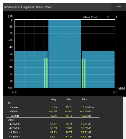
80MHz_30kHz_3660MHz-OFDM QPSK_RB108@54 -45.48,-45.76dB
