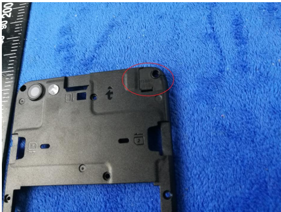
BT/WIFI/BLE/GPS - Antenna View
