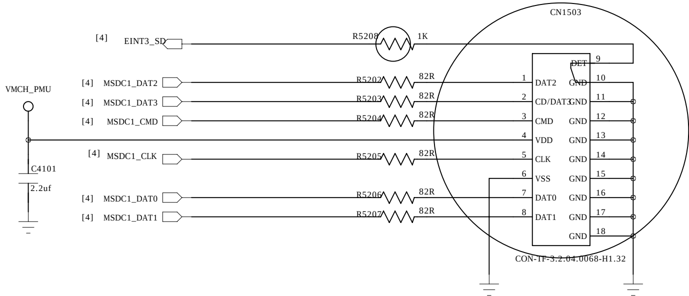
T_FLASH
