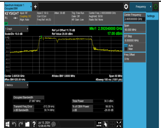
41(2555-2655)-41(2555-2655)-10MHz-20MHz-16QAM-16 QAM-40646-40790-50RB#0-100RB#0-PASS
