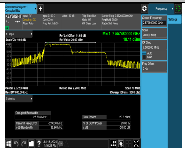
41(2555-2655)-41(2555-2655)-15MHz-20MHz-QPSK-QPS K-40318-40489-75RB#0-100RB#0-PASS
