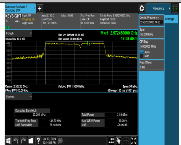
41(2555-2655)-41(2555-2655)-15MHz-10MHz-QPSK-QPS K-40315-40435-75RB#0-50RB#0-PASS
