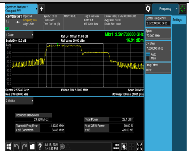
41(2555-2655)-41(2555-2655)-20MHz-15MHz-QPSK-QPS K-40340-40511-100RB#0-75RB#0-PASS
