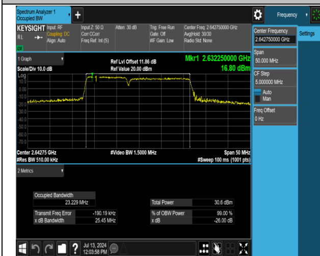
41(2555-2655)-41(2555-2655)-10MHz-15MHz-16QAM-16 QAM-41045-41165-50RB#0-75RB#0-PASS
