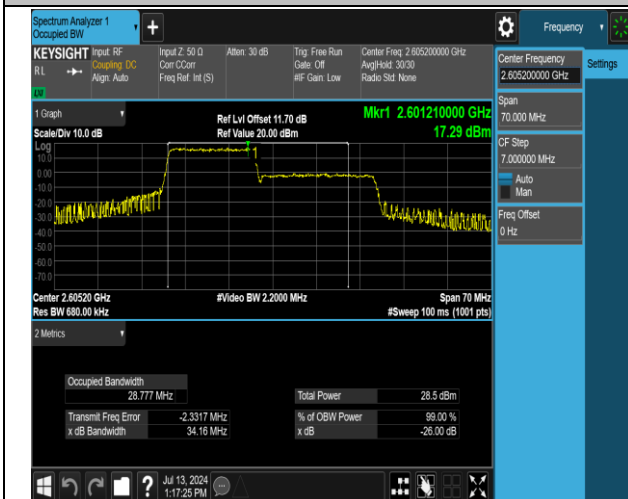
41(2555-2655)-41(2555-2655)-15MHz-20MHz-QPSK-QPS K-40644-40815-75RB#0-100RB#0-PASS
