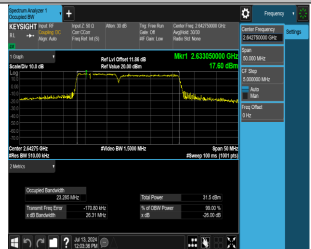
41(2555-2655)-41(2555-2655)-10MHz-15MHz-QPSK-QPS K-41045-41165-50RB#0-75RB#0-PASS
