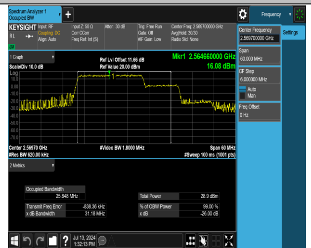
41(2555-2655)-41(2555-2655)-20MHz-10MHz-QPSK-QPS K-40340-40484-100RB#0-50RB#0-PASS
