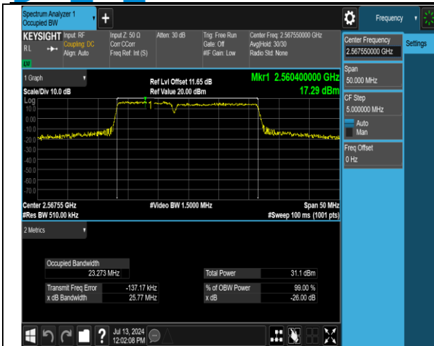
41(2555-2655)-41(2555-2655)-10MHz-15MHz-16QAM-16 QAM-40293-40413-50RB#0-75RB#0-PASS
