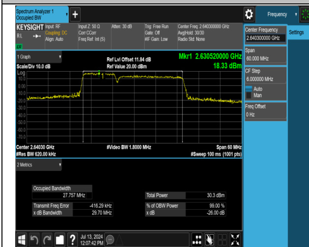
41(2555-2655)-41(2555-2655)-10MHz-20MHz-16QAM-16 QAM-40996-41140-50RB#0-100RB#0-PASS
