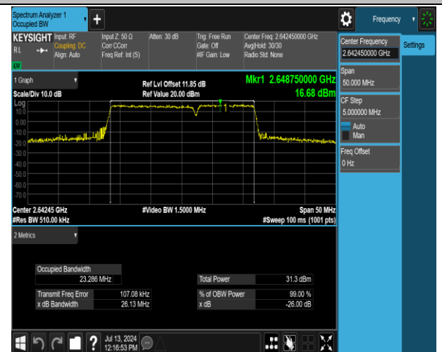
41(2555-2655)-41(2555-2655)-15MHz-10MHz-QPSK-QPS K-41067-41187-75RB#0-50RB#0-PASS
