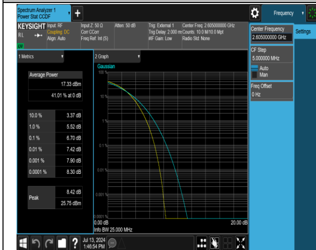
41(2555-2655)-41(2555-2655)-20MHz-20MHz-16QAM-16QAM-40641-40839-100RB#0-100RB#0-PASS
