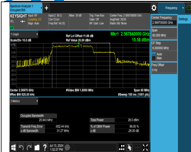
41(2555-2655)-41(2555-2655)-20MHz-10MHz-16QAM-16 QAM-40340-40484-100RB#0-50RB#0-PASS
