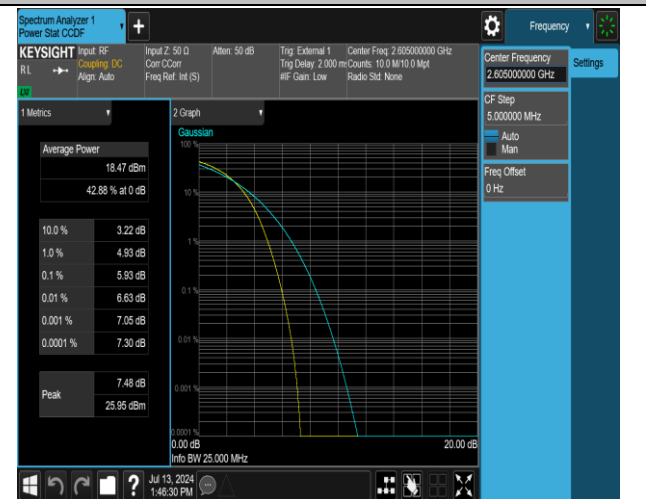
41(2555-2655)-41(2555-2655)-20MHz-20MHz-QPSK-QPSK-40641-40839-100RB#0-100RB#0-PASS
