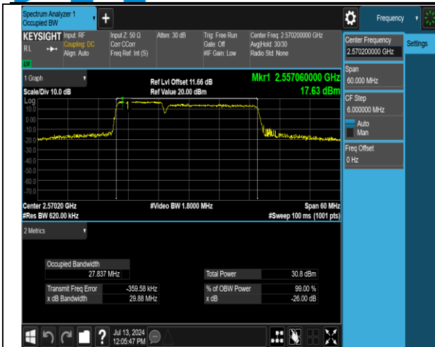
41(2555-2655)-41(2555-2655)-10MHz-20MHz-16QAM-16 QAM-40295-40439-50RB#0-100RB#0-PASS
