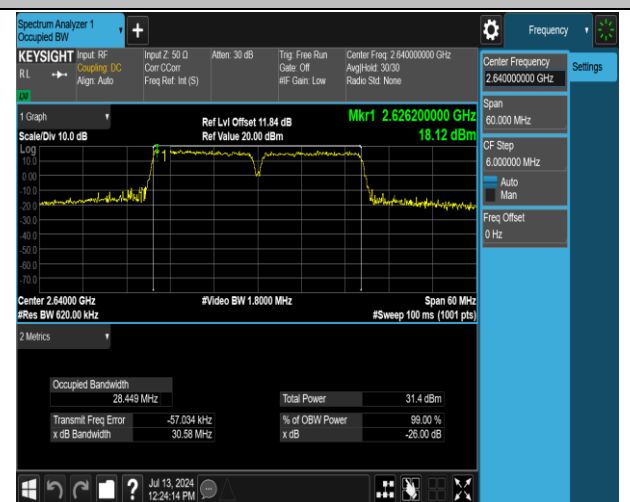
41(2555-2655)-41(2555-2655)-15MHz-15MHz-QPSK-QPS K-41015-41165-75RB#0-75RB#0-PASS
