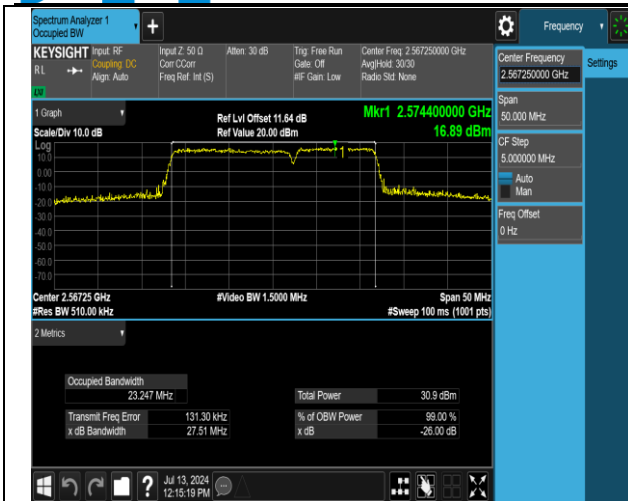
41(2555-2655)-41(2555-2655)-15MHz-10MHz-16QAM-16 QAM-40315-40435-75RB#0-50RB#0-PASS
