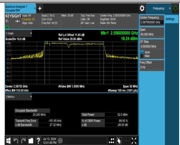
41(2555-2655)-41(2555-2655)-10MHz-15MHz-QPSK-QPS K-40293-40413-50RB#0-75RB#0-PASS
