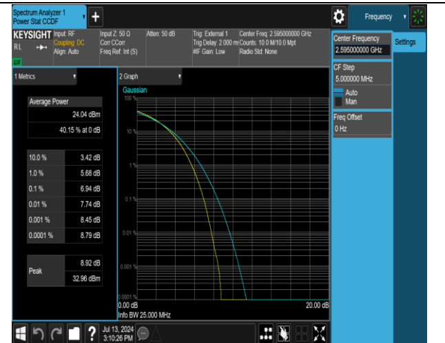
38-38-20MHz-20MHz-QPSK-QPSK-37901-38099-100RB#0-100RB#0-PASS
