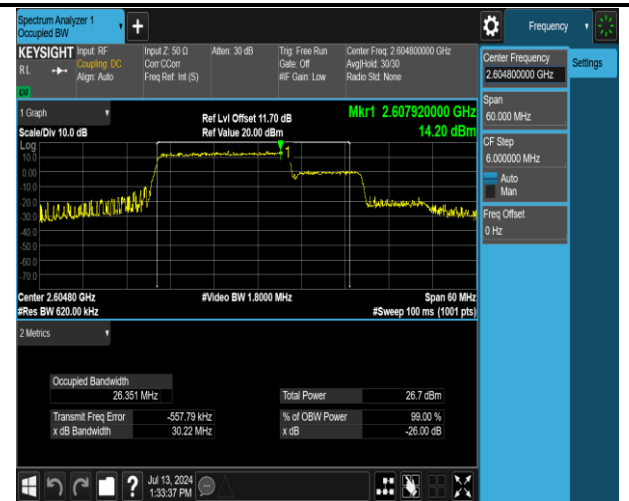
41(2555-2655)-41(2555-2655)-20MHz-10MHz-16QAM-16 QAM-40691-40835-100RB#0-50RB#0-PASS
