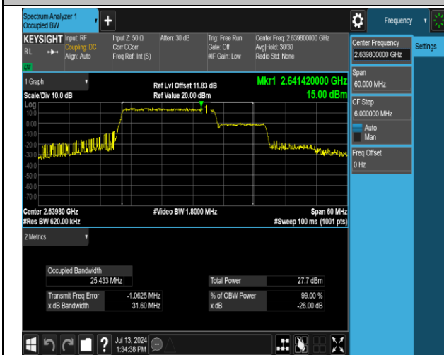
41(2555-2655)-41(2555-2655)-20MHz-10MHz-16QAM-16 QAM-41041-41185-100RB#0-50RB#0-PASS
