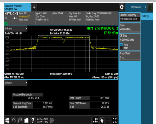
41(2555-2655)-41(2555-2655)-15MHz-15MHz-QPSK-QPS K-40315-40465-75RB#0-75RB#0-PASS
