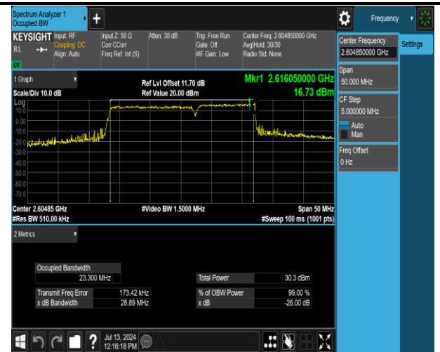
41(2555-2655)-41(2555-2655)-15MHz-10MHz-16QAM-16 QAM-40691-40811-75RB#0-50RB#0-PASS
