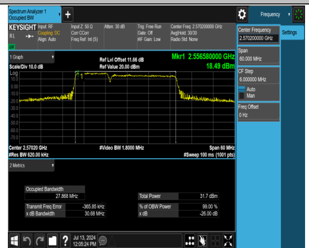
41(2555-2655)-41(2555-2655)-10MHz-20MHz-QPSK-QPS K-40295-40439-50RB#0-100RB#0-PASS
