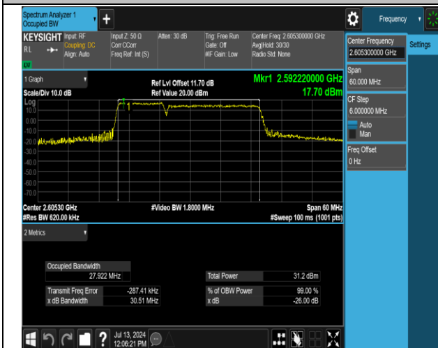
41(2555-2655)-41(2555-2655)-10MHz-20MHz-QPSK-QPS K-40646-40790-50RB#0-100RB#0-PASS
