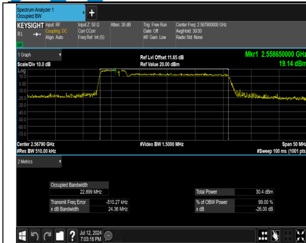
41(2555-2655)-41(2555-2655)-5MHz-20MHz-16QAM-16Q AM-40273-40390-25RB#0-100RB#0-PASS
