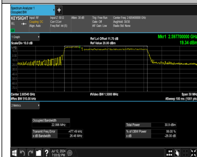
41(2555-2655)-41(2555-2655)-5MHz-20MHz-QPSK-QPSK -40648-40765-25RB#0-100RB#0-PASS
