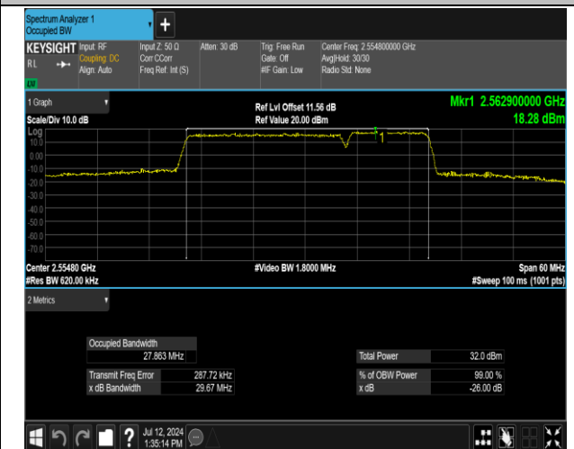
7-7-20MHz-10MHz-QPSK-QPSK-21251-21395-100RB#0- 50RB#0-PASS
