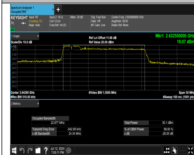
41(2555-2655)-41(2555-2655)-5MHz-20MHz-16QAM-16Q AM-41023-41140-25RB#0-100RB#0-PASS
