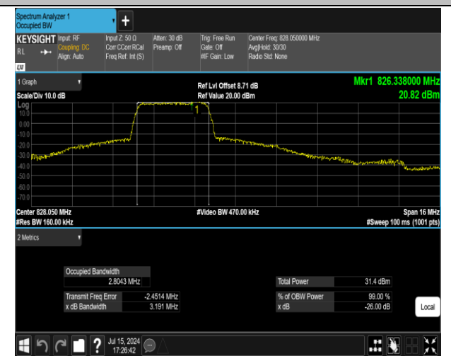
5-5-3MHz-5MHz-QPSK-QPSK-20416-20455-15RB#0-25R B#0-PASS
