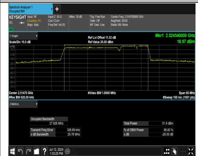
7-7-20MHz-10MHz-QPSK-QPSK-20850-20994-100RB#0- 50RB#0-PASS
