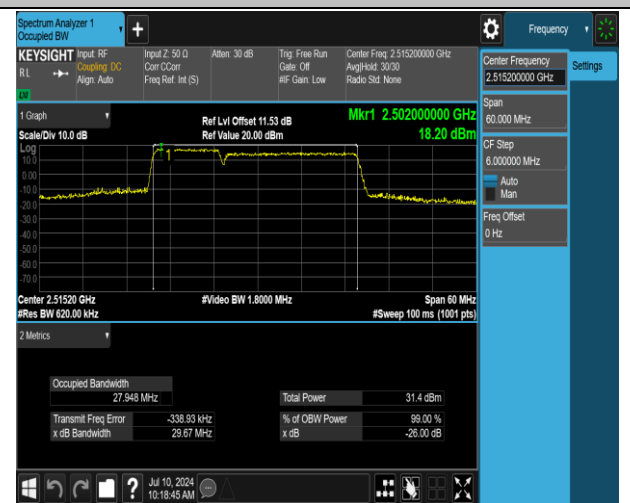
7-7-10MHz-20MHz-QPSK-QPSK-20805-20949-50RB#0-1 00RB#0-PASS
