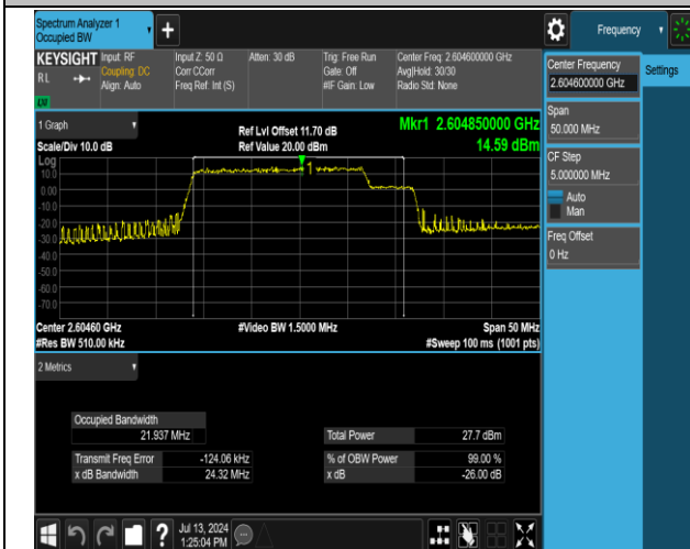
41(2555-2655)-41(2555-2655)-20MHz-5MHz-QPSK-QPSK -40715-40832-100RB#0-25RB#0-PASS
