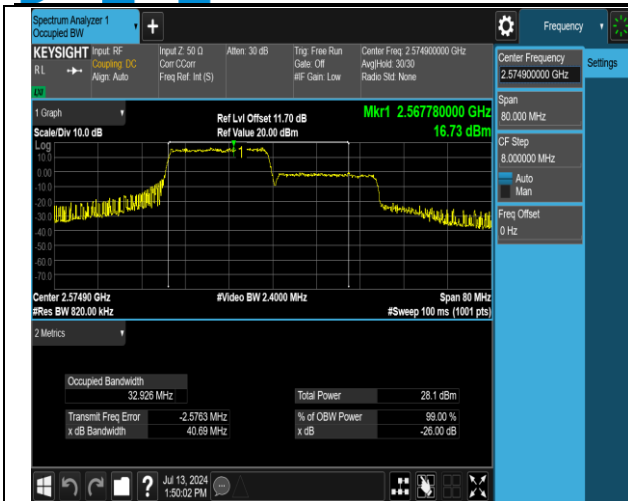
41(2555-2655)-41(2555-2655)-20MHz-20MHz-16QAM-16 QAM-40340-40538-100RB#0-100RB#0-PASS
