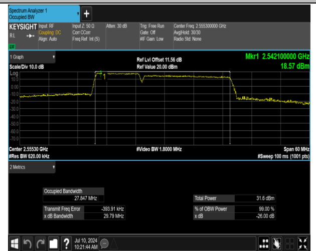
7-7-10MHz-20MHz-QPSK-QPSK-21206-21350-50RB#0-1 00RB#0-PASS
