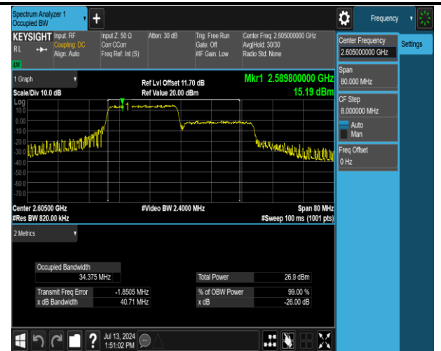
41(2555-2655)-41(2555-2655)-20MHz-20MHz-16QAM-16 QAM-40641-40839-100RB#0-100RB#0-PASS
