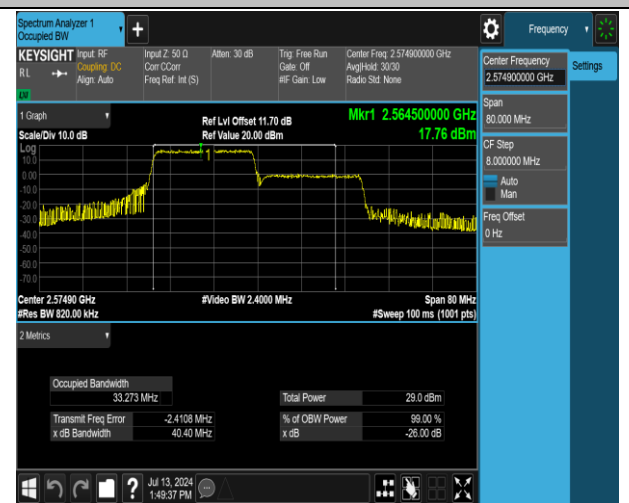
41(2555-2655)-41(2555-2655)-20MHz-20MHz-QPSK-QPS K-40340-40538-100RB#0-100RB#0-PASS
