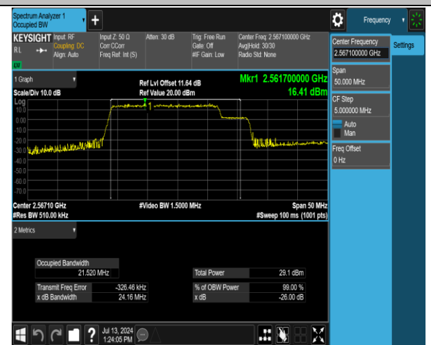
41(2555-2655)-41(2555-2655)-20MHz-5MHz-QPSK-QPSK -40340-40457-100RB#0-25RB#0-PASS
