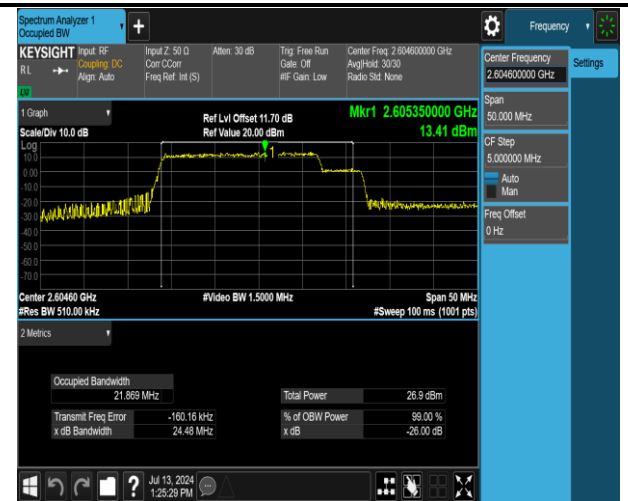
41(2555-2655)-41(2555-2655)-20MHz-5MHz-16QAM-16Q AM-40715-40832-100RB#0-25RB#0-PASS
