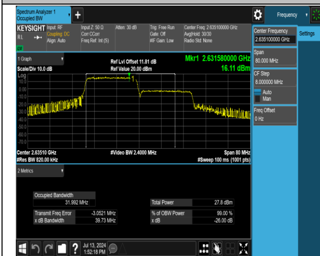
41(2555-2655)-41(2555-2655)-20MHz-20MHz-16QAM-16 QAM-40942-41140-100RB#0-100RB#0-PASS
