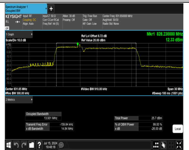
5-5-5MHz-10MHz-QPSK-QPSK-20428-20500-25RB#0-50RB#0-PASS
