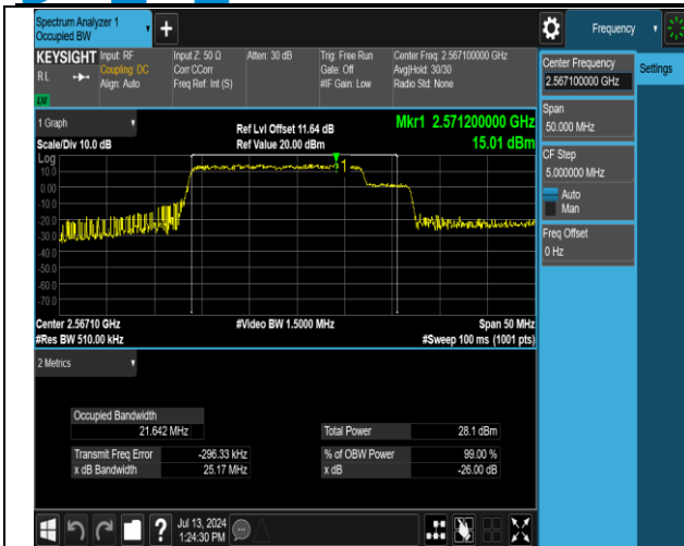
41(2555-2655)-41(2555-2655)-20MHz-5MHz-16QAM-16Q AM-40340-40457-100RB#0-25RB#0-PASS
