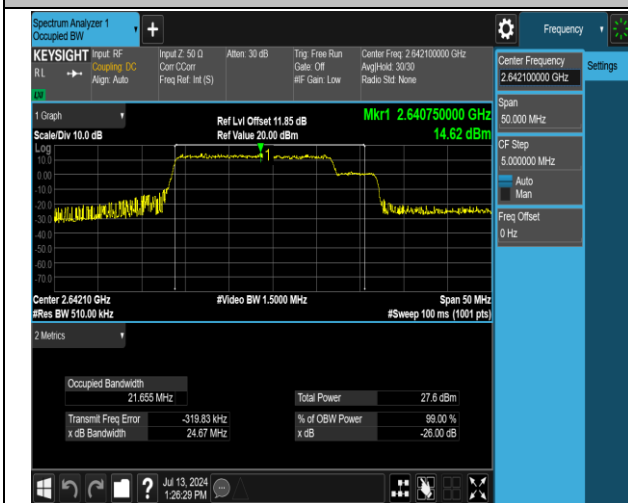
41(2555-2655)-41(2555-2655)-20MHz-5MHz-16QAM-16Q AM-41090-41207-100RB#0-25RB#0-PASS
