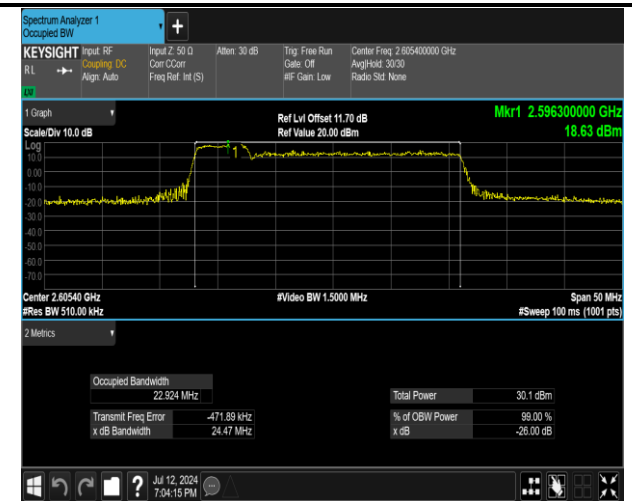
41(2555-2655)-41(2555-2655)-5MHz-20MHz-16QAM-16Q AM-40648-40765-25RB#0-100RB#0-PASS
