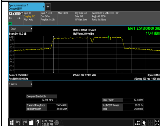
7-7-20MHz-15MHz-QPSK-QPSK-21026-21197-100RB#0- 75RB#0-PASS
