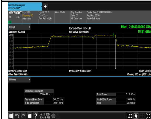
7-7-20MHz-10MHz-QPSK-QPSK-21051-21195-100RB#0- 50RB#0-PASS
