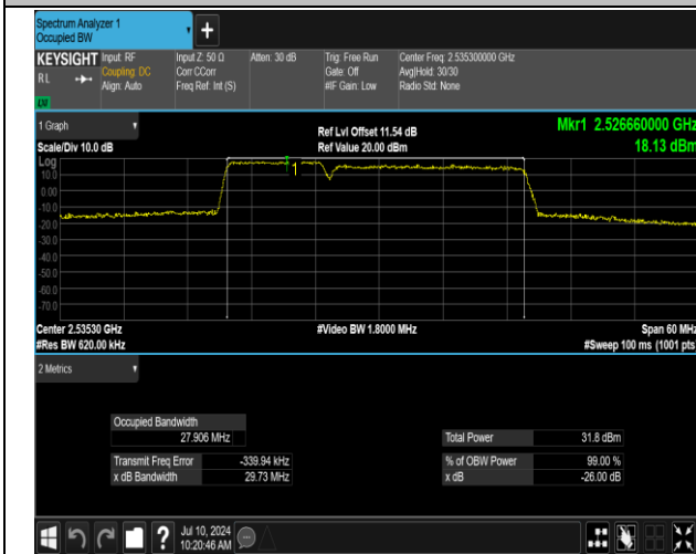
7-7-10MHz-20MHz-QPSK-QPSK-21006-21150-50RB#0-1 00RB#0-PASS
