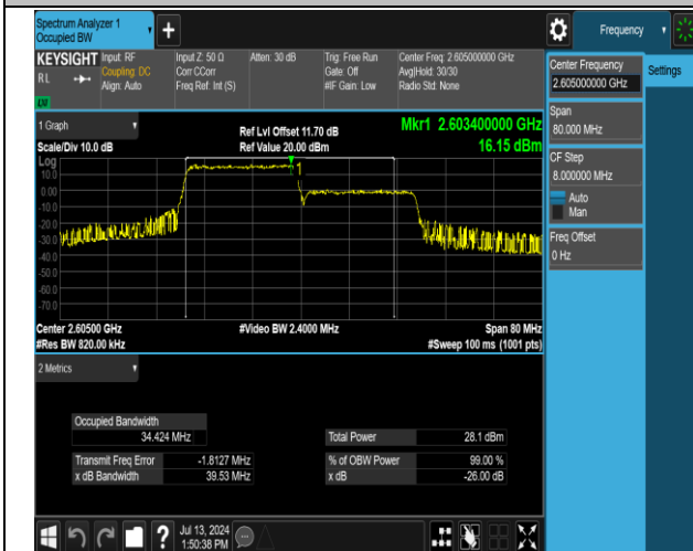
41(2555-2655)-41(2555-2655)-20MHz-20MHz-QPSK-QPS K-40641-40839-100RB#0-100RB#0-PASS
