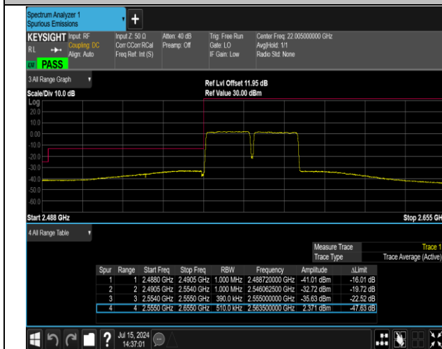
41(2555-2655)-41(2555-2655)-20MHz-20MHz-16QAM@16
