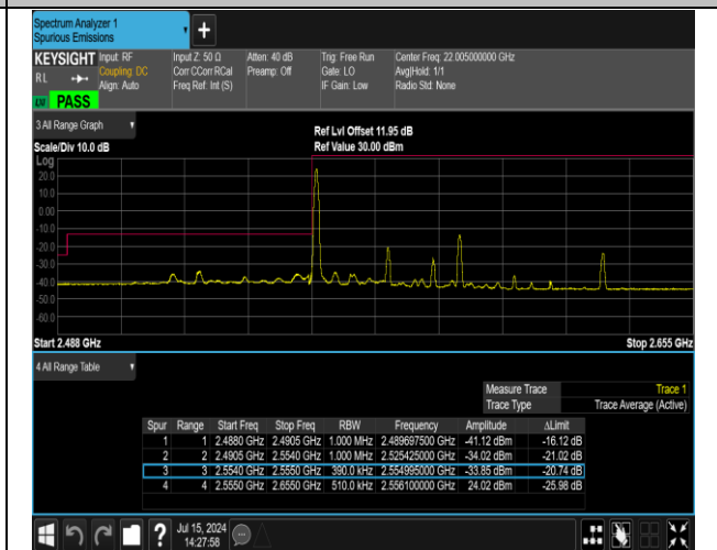
41(2555-2655)-41(2555-2655)-20MHz-20MHz-16QAM@1
