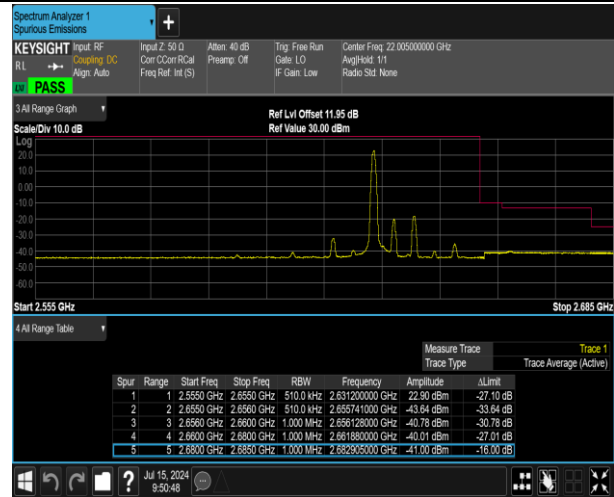
0RB#0@100RB#0-PASS
