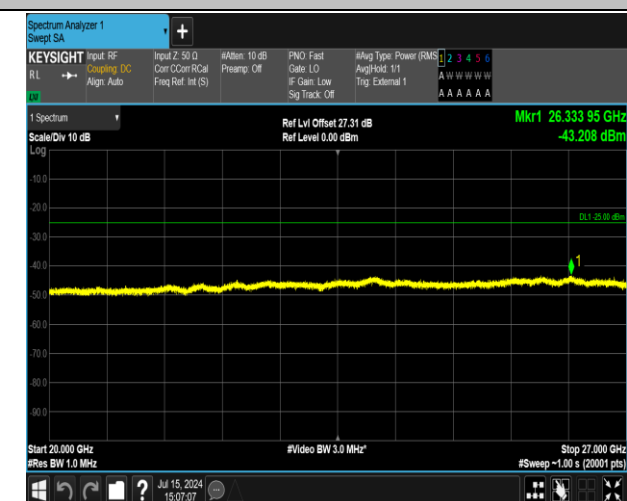
41(2555-2655)-41(2555-2655)-20MHz-20MHz-16QAM-16 QAM-40340-40538-100RB#0-100RB#0-20000~27000MHz
