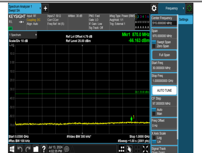
38-38-20MHz-20MHz-QPSK-QPSK-37901-38099-1RB#99-ORB#0-30~1000MHz-PASS
