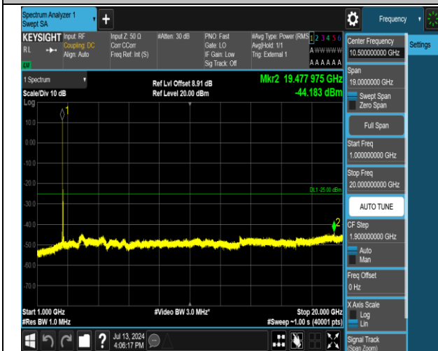
38-38-20MHz-20MHz-QPSK-QPSK-37901-38099-1RB#0- 1RB#99-1000~20000MHz-PASS
