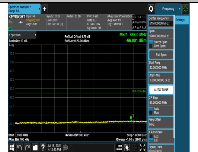
38-38-20MHz-20MHz-QPSK-QPSK-37952-38150-1RB#0- RB#0-30~1000MHz-PASS
