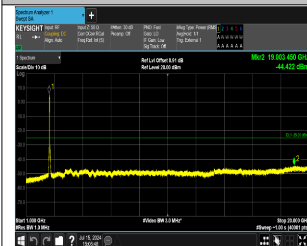
41(2555-2655)-41(2555-2655)-20MHz-20MHz-16QAM-16 QAM-40340-40538-100RB#0-100RB#0-1000~20000MHz-
