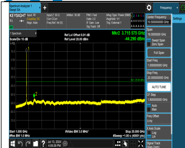
38-38-20MHz-20MHz-QPSK-QPSK-37901-38099-100RB# 0-100RB#0-1000~20000MHz-PASS
