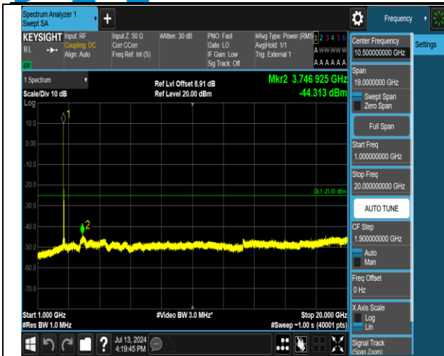
38-38-20MHz-20MHz-QPSK-QPSK-37952-38150-1RB#0- 1RB#99-1000~20000MHz-PASS
