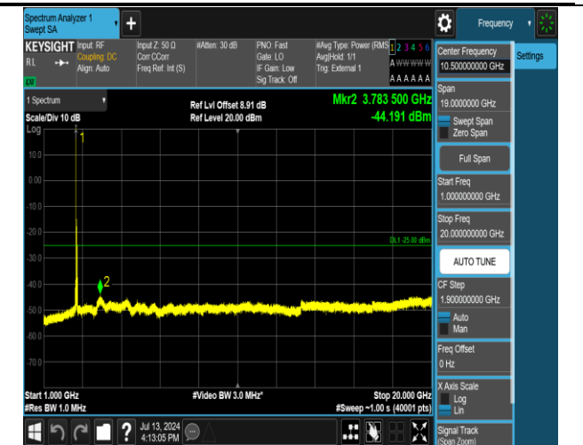
38-38-20MHz-20MHz-QPSK-QPSK-37952-38150-1RB#0- RB#0-1000~20000MHz-PASS
