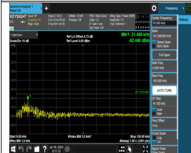
38-38-20MHz-20MHz-QPSK-QPSK-37952-38150-1RB#0- 1RB#99-0.009~0.15MHz-PASS
