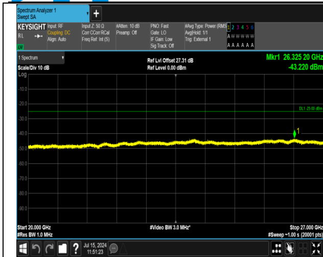
41(2555-2655)-41(2555-2655)-20MHz-5MHz-16QAM-16Q AM-40340-40457-1RB#0-ORB#0-20000~27000MHz-PASS
