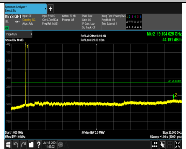
41(2555-2655)-41(2555-2655)-20MHz-5MHz-QPSK-QPSK -40340-40457-1RB#99-0RB#0-1000~20000MHz-PASS
