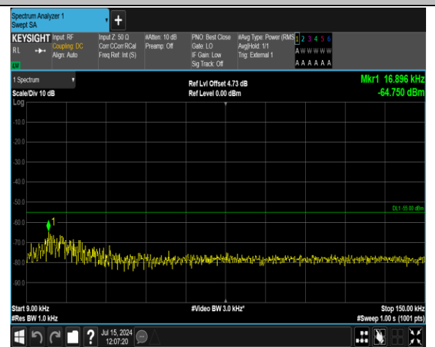
41(2555-2655)-41(2555-2655)-20MHz-5MHz-QPSK-QPSK -40715-40832-1RB#99-0RB#0-0.009~0.15MHz-PASS
