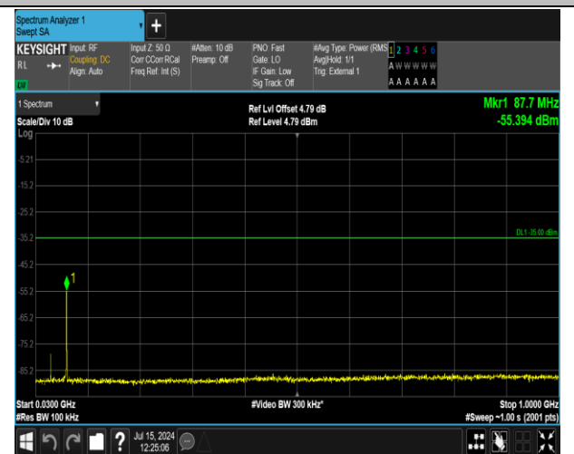
41(2555-2655)-41(2555-2655)-20MHz-5MHz-16QAM-16Q AM-41090-41207-1RB#99-ORB#0-30~1000MHz-PASS
