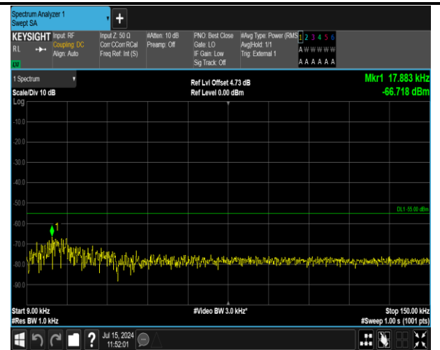
41(2555-2655)-41(2555-2655)-20MHz-5MHz-QPSK-QPSK -40340-40457-1RB#99-0RB#0-0.009~0.15MHz-PASS
