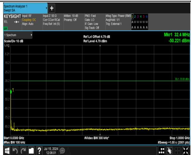
41(2555-2655)-41(2555-2655)-20MHz-5MHz-16QAM-16Q AM-40715-40832-1RB#0-0RB#0-30~1000MHz-PASS
