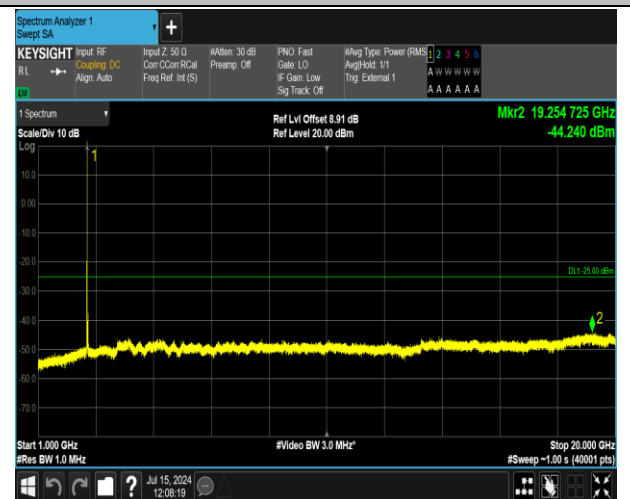
41(2555-2655)-41(2555-2655)-20MHz-5MHz-QPSK-QPSK -40715-40832-1RB#99-0RB#0-1000~20000MHz-PASS
