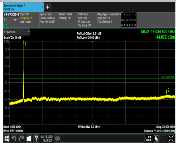
41(2555-2655)-41(2555-2655)-20MHz-5MHz-16QAM-16Q AM-40715-40832-1RB#0-0RB#0-1000~20000MHz-PASS
