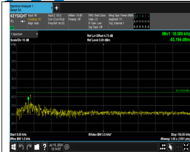
41(2555-2655)-41(2555-2655)-20MHz-5MHz-QPSK-QPS K-40715-40832-100RB#0-25RB#0-0.009~0.15MHz-PASS
