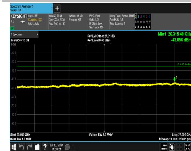
41(2555-2655)-41(2555-2655)-20MHz-5MHz-QPSK-QPS K-40340-40457-1RB#99-0RB#0-20000~27000MHz-PASS
