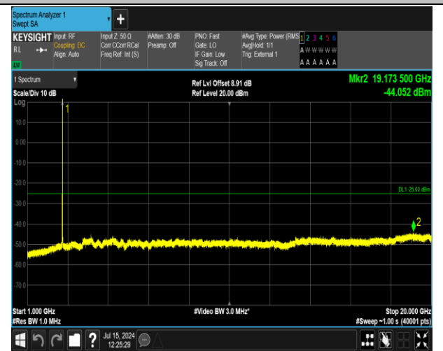
41(2555-2655)-41(2555-2655)-20MHz-5MHz-16QAM-16Q AM-41090-41207-1RB#99-ORB#0-1000~20000MHz-PASS
