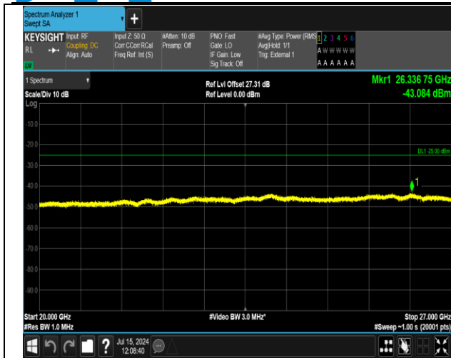
41(2555-2655)-41(2555-2655)-20MHz-5MHz-QPSK-QPS K-40715-40832-1RB#99-0RB#0-20000~27000MHz-PASS
