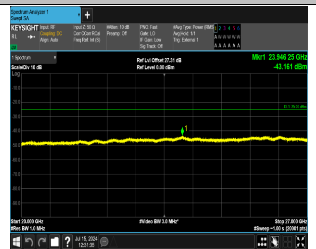
41(2555-2655)-41(2555-2655)-20MHz-5MHz-QPSK-QPSK -41090-41207-100RB#0-25RB#0-20000~27000MHz-PASS
