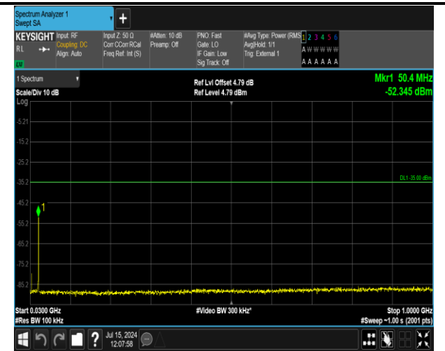
41(2555-2655)-41(2555-2655)-20MHz-5MHz-QPSK-QPSK -40715-40832-1RB#99-0RB#0-30~1000MHz-PASS
