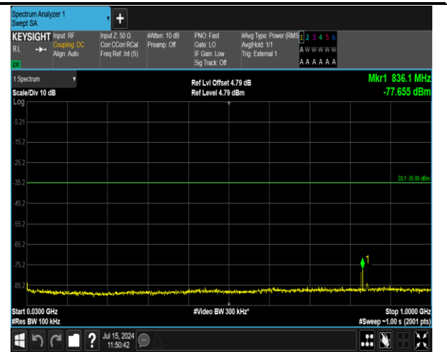
41(2555-2655)-41(2555-2655)-20MHz-5MHz-16QAM-16Q AM-40340-40457-1RB#0-ORB#0-30~1000MHz-PASS
