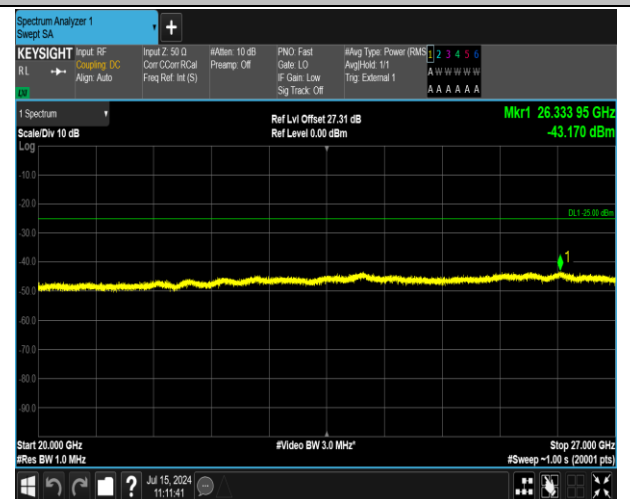
41(2555-2655)-41(2555-2655)-5MHz-20MHz-QPSK-QPSK -41023-41140-1RB#24-0RB#0-20000~27000MHz-PASS
