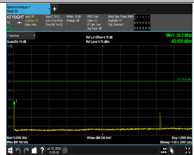
41(2555-2655)-41(2555-2655)-5MHz-20MHz-QPSK-QPSK -40648-40765-25RB#0-100RB#0-30~1000MHz-PASS
