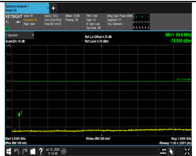
41(2555-2655)-41(2555-2655)-5MHz-20MHz-QPSK-QPSK -41023-41140-1RB#0-1RB#99-30~1000MHz-PASS
