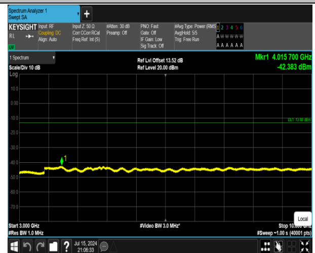
5-5-10MHz-10MHz-QPSK-QPSK-20501-20600-50RB#0-50 RB#0-3000~10000MHz-PASS
