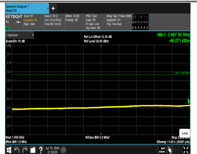
5-5-10MHz-10MHz-QPSK-QPSK-20501-20600-1RB#0-1R B#49-1000~3000MHz-PASS
