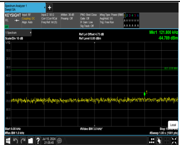
5-5-10MHz-10MHz-QPSK-QPSK-20501-20600-50RB#0-50 RB#0-0.009~0.15MHz-PASS
