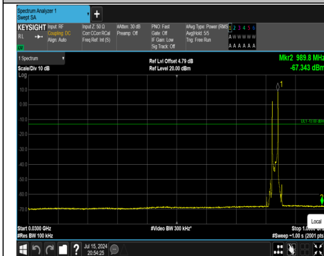
5-5-10MHz-10MHz-QPSK-QPSK-20476-20575-1RB#0-1R B#49-30~1000MHz-PASS
