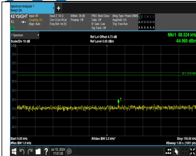
5-5-3MHz-5MHz-QPSK-QPSK-20416-20455-15RB#0-25R B#0-0.009~0.15MHz-PASS
