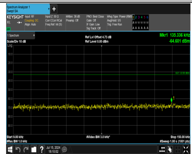
5-5-3MHz-5MHz-QPSK-QPSK-20586-20625-1RB#0-0RB# 0-0.009~0.15MHz-PASS
