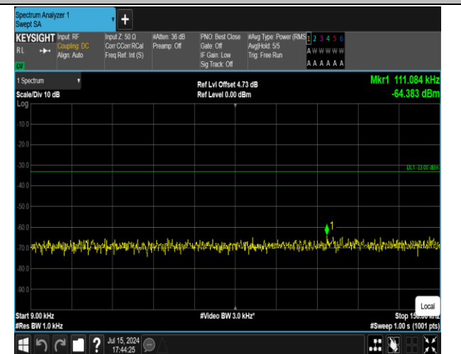
5-5-3MHz-5MHz-QPSK-QPSK-20416-20455-1RB#0-0RB# 0-0.009~0.15MHz-PASS
