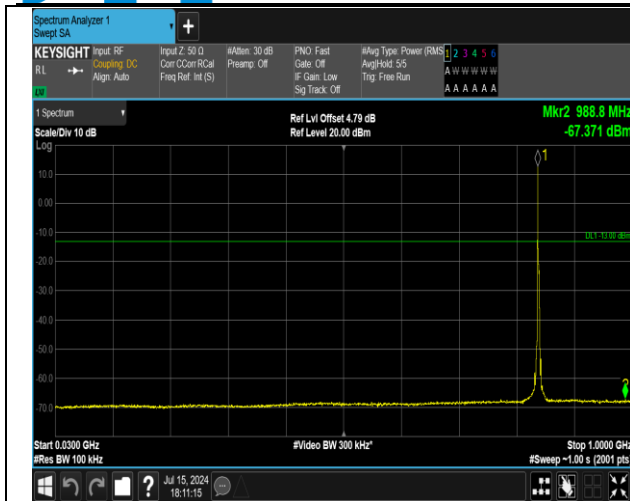
5-5-3MHz-5MHz-QPSK-QPSK-20586-20625-1RB#0-0RB# 0-30~1000MHz-PASS
