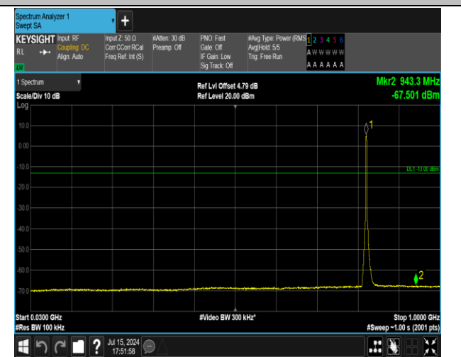
5-5-3MHz-5MHz-QPSK-QPSK-20416-20455-15RB#0-25R B#0-30~1000MHz-PASS
