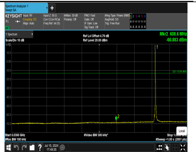
5-5-3MHz-5MHz-QPSK-QPSK-20416-20455-1RB#0-1RB# 24-30~1000MHz-PASS
