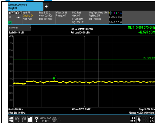
5-5-3MHz-5MHz-QPSK-QPSK-20501-20540-15RB#0-25R# B#0-3000~10000MHz-PASS
