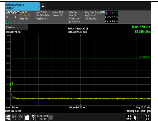
5-5-3MHz-5MHz-QPSK-QPSK-20416-20455-15RB#0-25R B#0-0.15~30MHz-PASS
