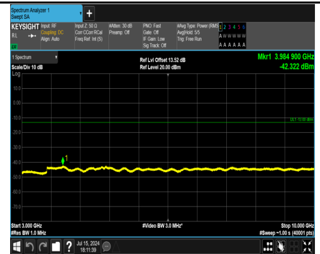
5-5-3MHz-5MHz-QPSK-QPSK-20586-20625-1RB#0-0RB# 0-3000~10000MHz-PASS
