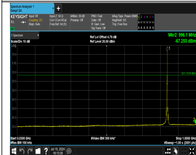
5-5-3MHz-5MHz-QPSK-QPSK-20586-20625-1RB#14-0RB #0-30~1000MHz-PASS
