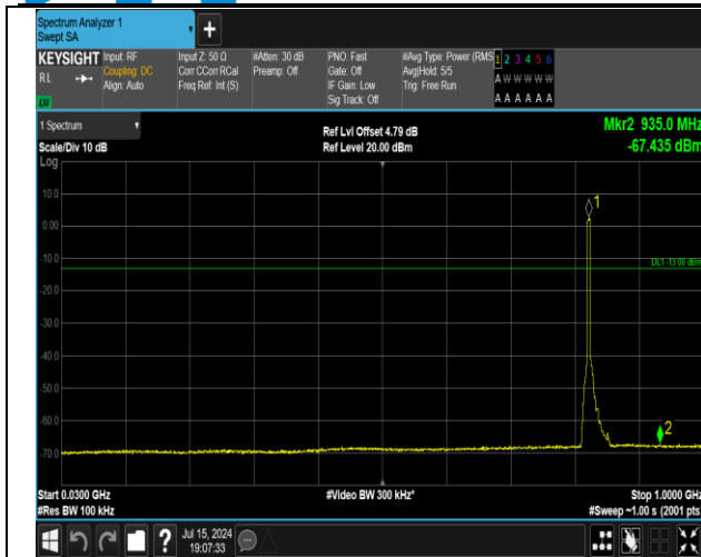
5-5-5MHz-3MHz-QPSK-QPSK-20425-20464-25RB#0-15R B#0-30~1000MHz-PASS
