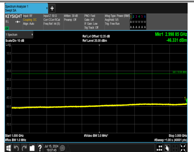
5-5-5MHz-3MHz-QPSK-QPSK-20425-20464-25RB#0-15R B#0-1000~3000MHz-PASS
