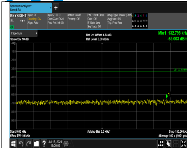
5-5-5MHz-3MHz-QPSK-QPSK-20425-20464-1RB#0-0RB# 0-0.009~0.15MHz-PASS
