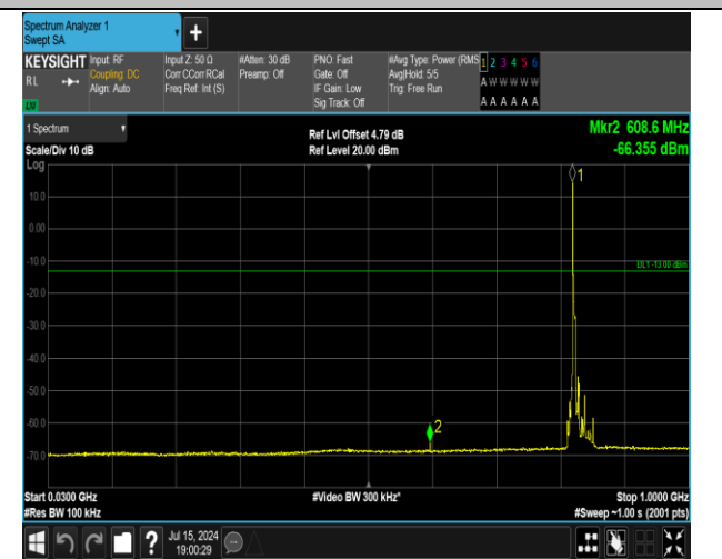
5-5-5MHz-3MHz-QPSK-QPSK-20425-20464-1RB#0-0RB# 0-30~1000MHz-PASS
