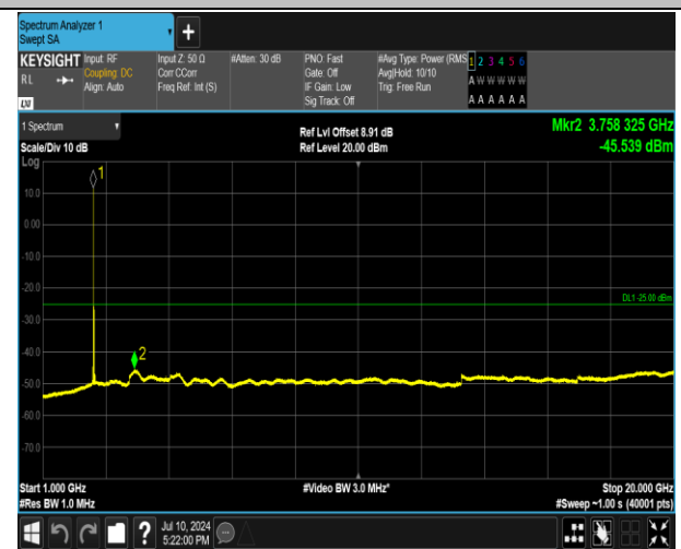
7-7-15MHz-10MHz-QPSK-QPSK-21051-21171-1RB#0-1R B#49-1000~20000MHz-PASS
