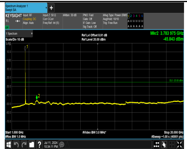
7-7-15MHz-20MHz-QPSK-QPSK-20828-20999-1RB#0-1R B#99-1000~20000MHz-PASS
