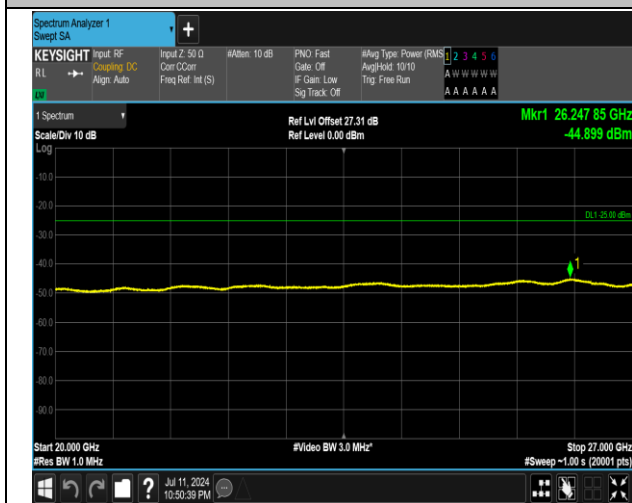
7-7-15MHz-20MHz-QPSK-QPSK-21003-21174-75RB#0-1 00RB#0-20000~27000MHz-PASS
