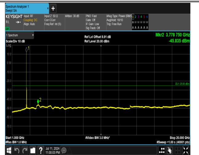
7-7-15MHz-20MHz-QPSK-QPSK-21179-21350-1RB#0-1R B#99-1000~20000MHz-PASS
