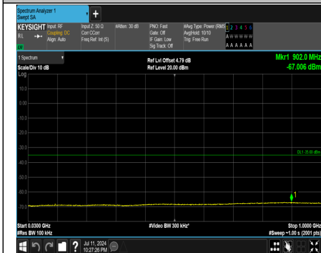
7-7-15MHz-20MHz-QPSK-QPSK-20828-20999-1RB#0-0R B#0-30~1000MHz-PASS
