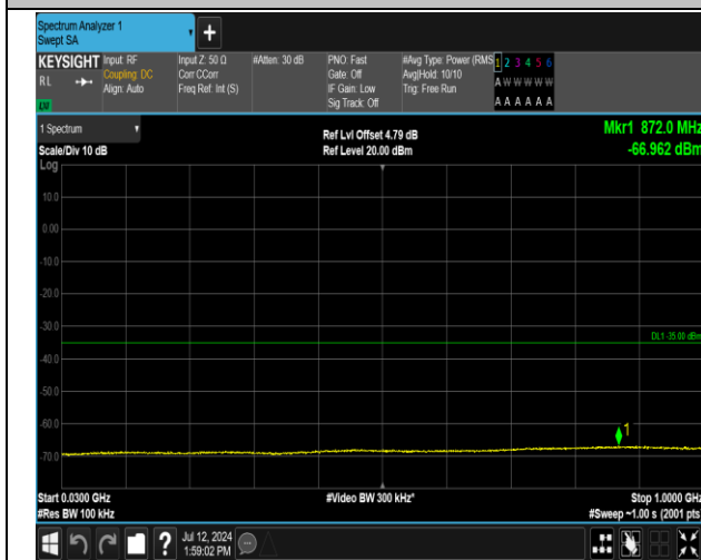
7-7-20MHz-10MHz-QPSK-QPSK-20850-20994-1RB#0-1R B#49-30~1000MHz-PASS
