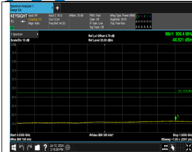
7-7-20MHz-10MHz-QPSK-QPSK-21051-21195-100RB#0-50RB#0-30~1000MHz-PASS
