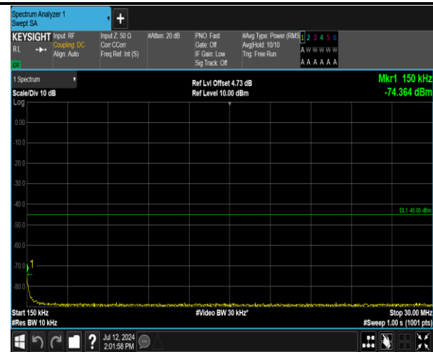
7-7-20MHz-10MHz-QPSK-QPSK-20850-20994-100RB#0-50RB#0-0.15~30MHz-PASS
