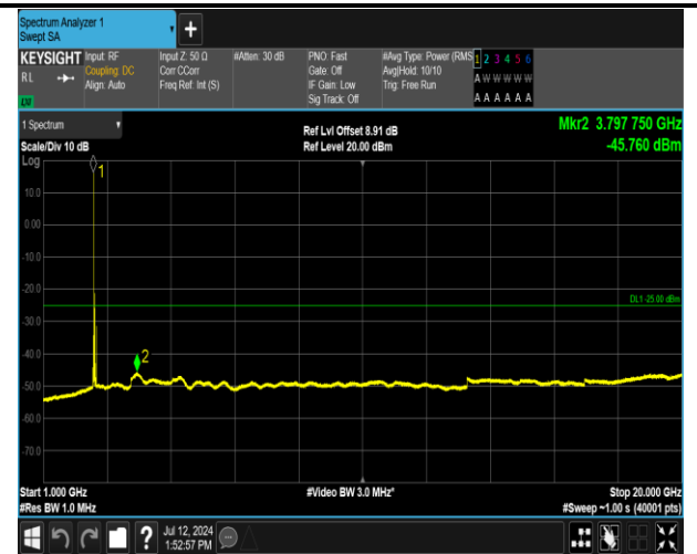
7-7-20MHz-10MHz-QPSK-QPSK-20850-20994-1RB#0-0R B#0-1000~20000MHz-PASS
