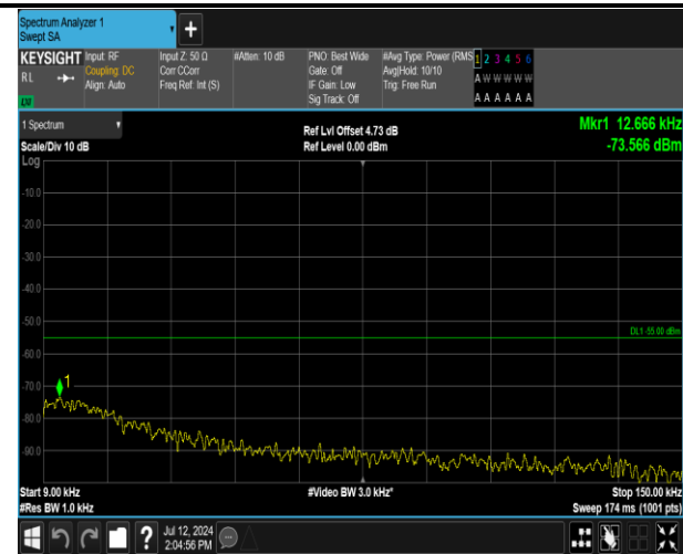
7-7-20MHz-10MHz-QPSK-QPSK-21051-21195-1RB#0-0RB#0-0.009~0.15MHz-PASS
