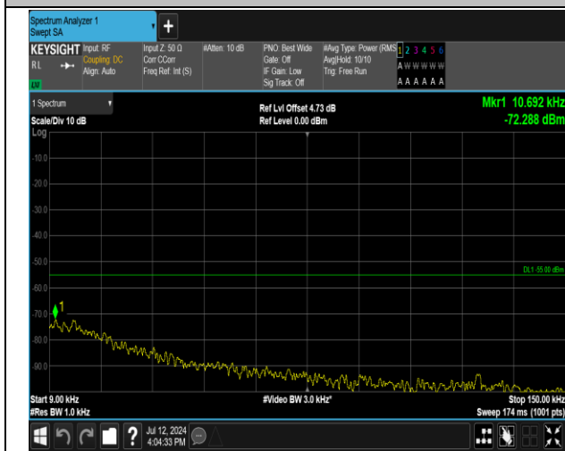
7-7-20MHz-15MHz-QPSK-QPSK-21026-21197-100RB#0-75RB#0-0.009~0.15MHz-PASS
