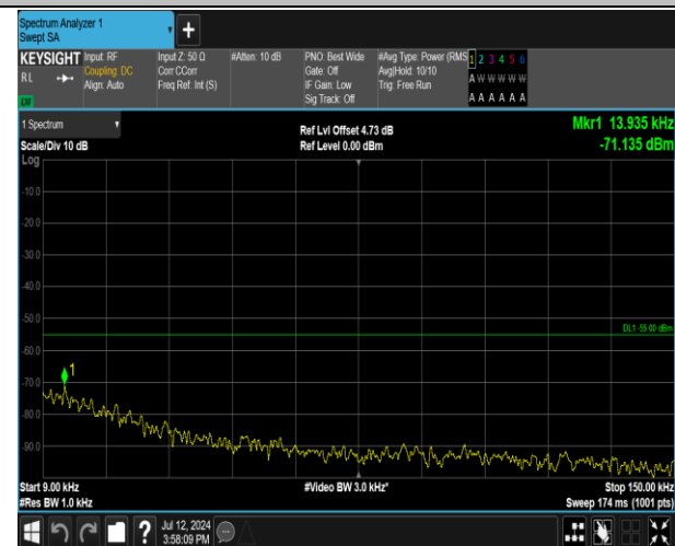
7-7-20MHz-15MHz-QPSK-QPSK-21026-21197-1RB#99-0 RB#0-0.009~0.15MHz-PASS
