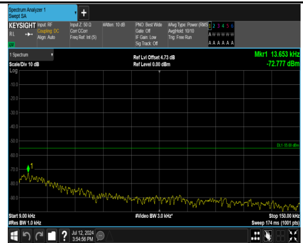
7-7-20MHz-15MHz-QPSK-QPSK-21026-21197-1RB#0-0RB#0-0.009~0.15MHz-PASS
