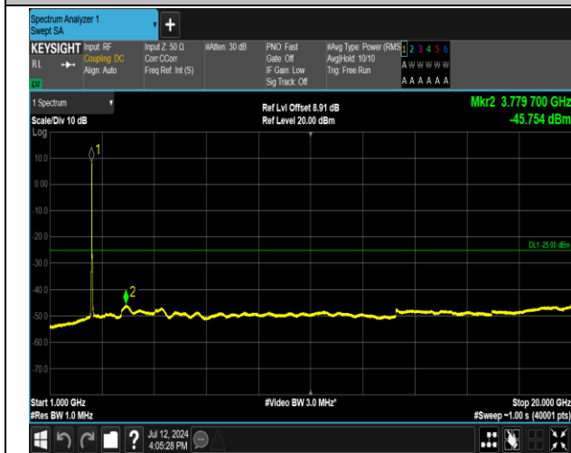
7-7-20MHz-15MHz-QPSK-QPSK-21026-21197-100RB#0-75RB#0-1000~20000MHz-PASS
