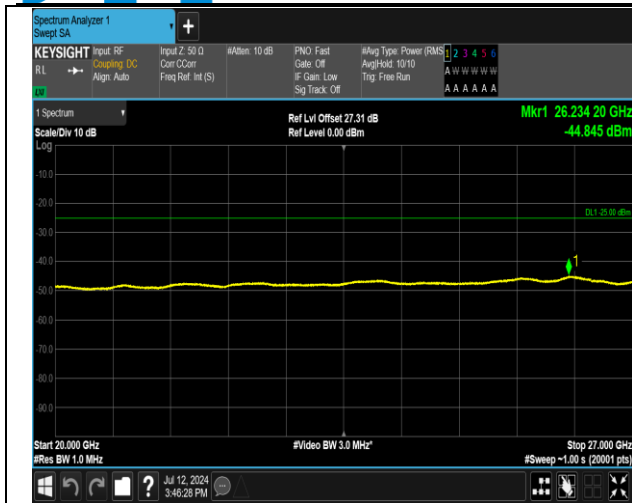
7-7-20MHz-15MHz-QPSK-QPSK-20850-21021-1RB#99-0 RB#0-20000~27000MHz-PASS
