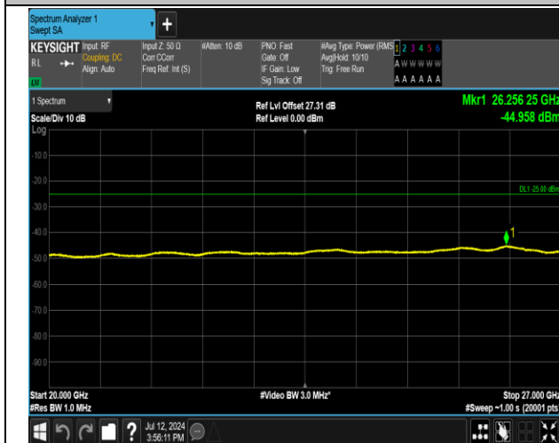
7-7-20MHz-15MHz-QPSK-QPSK-21026-21197-1RB#0-0RB#0-20000~27000MHz-PASS
