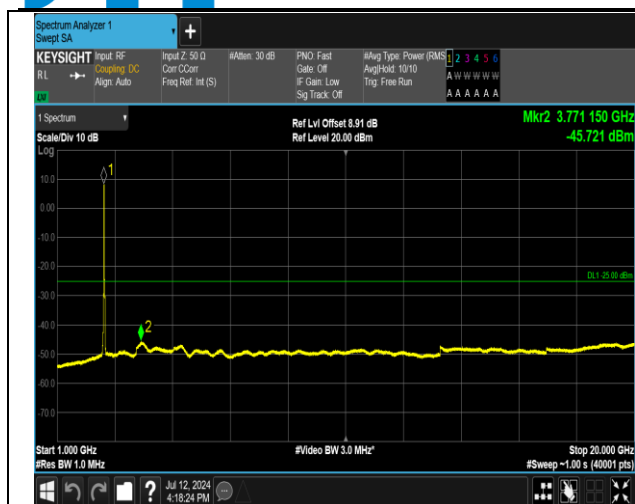
7-7-20MHz-15MHz-QPSK-QPSK-21201-21372-100RB#0- 75RB#0-1000~20000MHz-PASS
