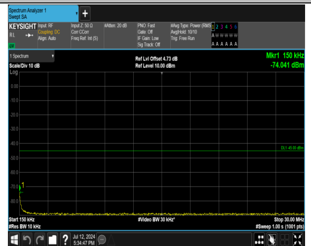
7-7-20MHz-20MHz-QPSK-QPSK-20850-21048-1RB#0-1R B#99-0.15~30MHz-PASS
