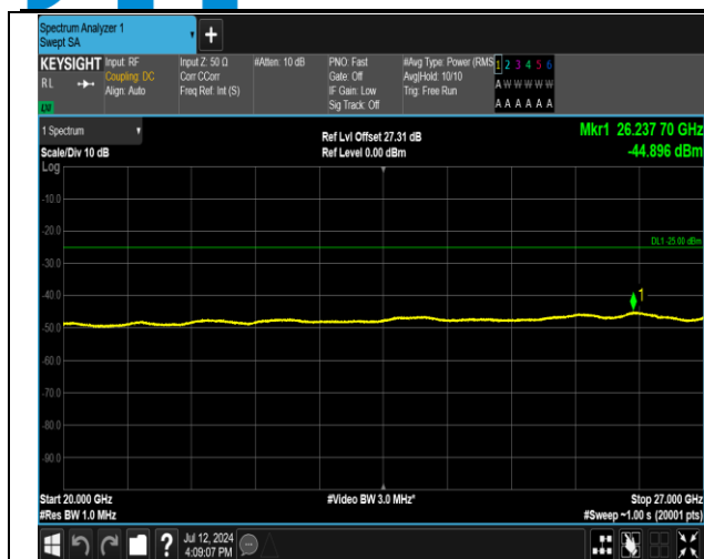
7-7-20MHz-15MHz-QPSK-QPSK-21201-21372-1RB#0-0R B#0-20000~27000MHz-PASS
