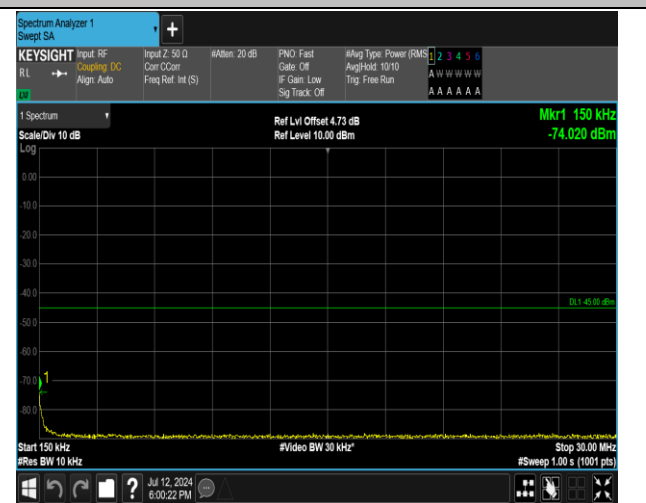
7-7-20MHz-20MHz-QPSK-QPSK-21152-21350-1RB#0-1R B#99-0.15~30MHz-PASS
