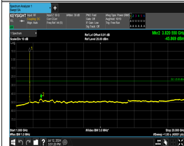
7-7-20MHz-20MHz-QPSK-QPSK-21001-21199-100RB#0- 100RB#0-1000~20000MHz-PASS
