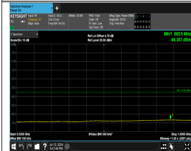
7-7-20MHz-20MHz-QPSK-QPSK-21001-21199-1RB#0-1R B#99-30~1000MHz-PASS
