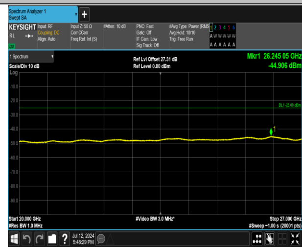
7-7-20MHz-20MHz-QPSK-QPSK-21001-21199-1RB#0-1R B#99-20000~27000MHz-PASS
