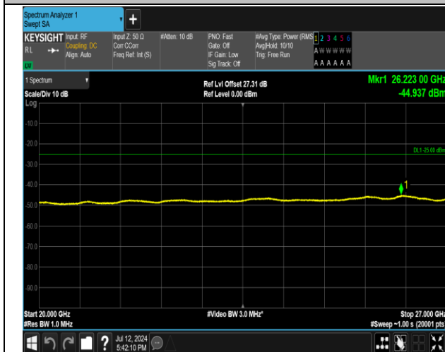
7-7-20MHz-20MHz-QPSK-QPSK-21001-21199-1RB#0-0RB#0-20000~27000MHz-PASS
