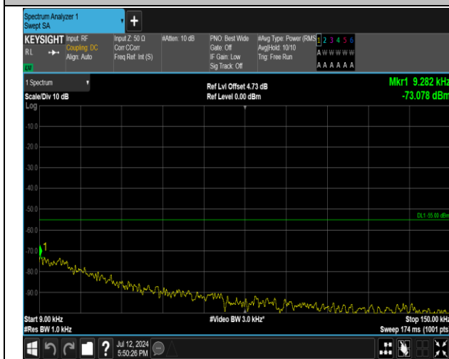
7-7-20MHz-20MHz-QPSK-QPSK-21001-21199-100RB#0- 100RB#0-0.009~0.15MHz-PASS
