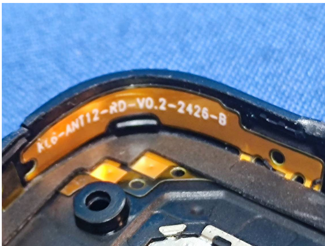
GPS Antenna(ANT 12)
