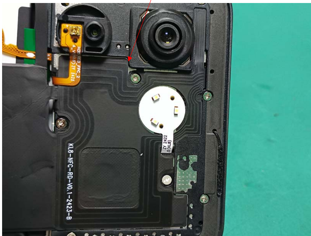
NFC Antenna
