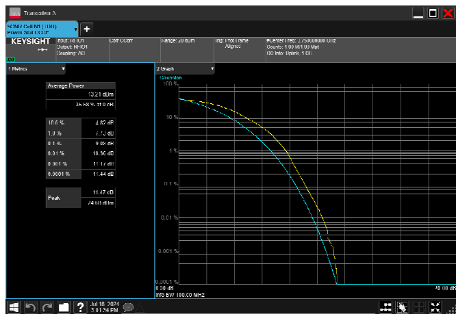
n78_3_100MHz_30kHz_3750MHz_CP-OFDM QPSK_RB273@0 10.96dB
