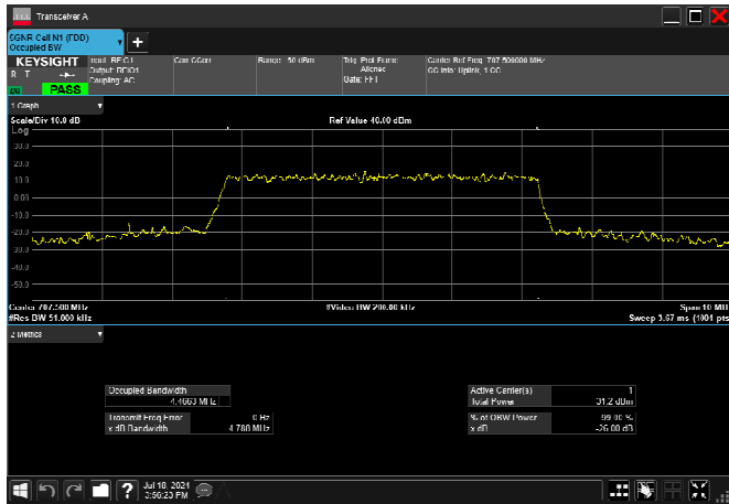
n12_5MHz_15kHz_707.5MHz_CP-OFDM 256 QAM_RB25@0 4.465MHz
