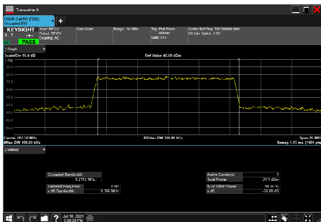
n12_10MHz_15kHz_707.5MHz_DFT-s-OFDM QPSK_RB50@0 9.211MHz
